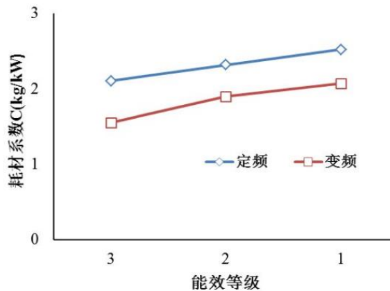
图15.铜耗材系数随能效比增加而增大
