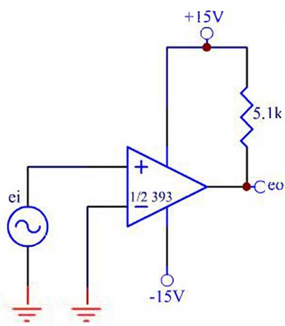
过零检波器
