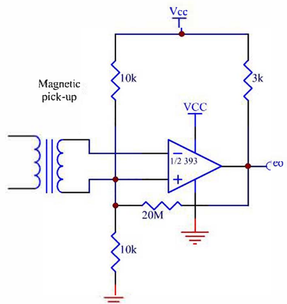
换能放大器
