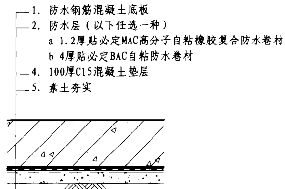
②地下室底板二级防水构造
