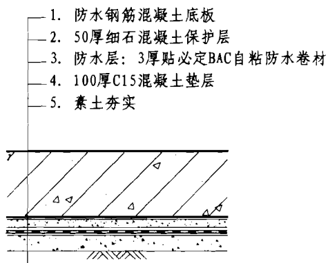
①地下室底板二级防水构造
