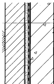
③ 地下室外墙二级防水构造（外防内贴）
