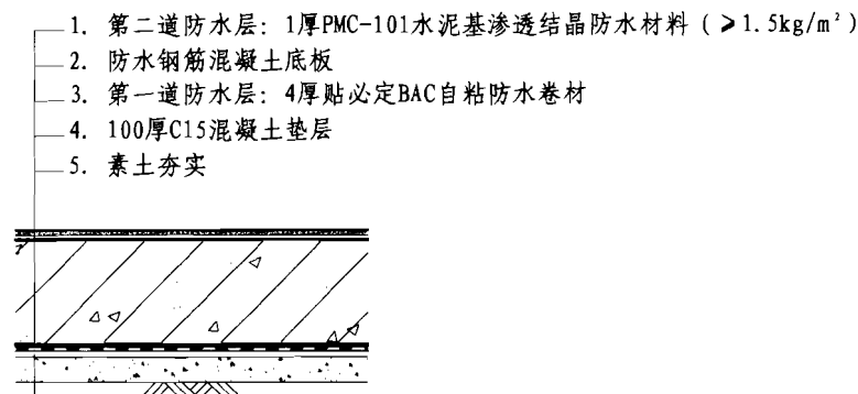
④地下室底板一级防水构造
