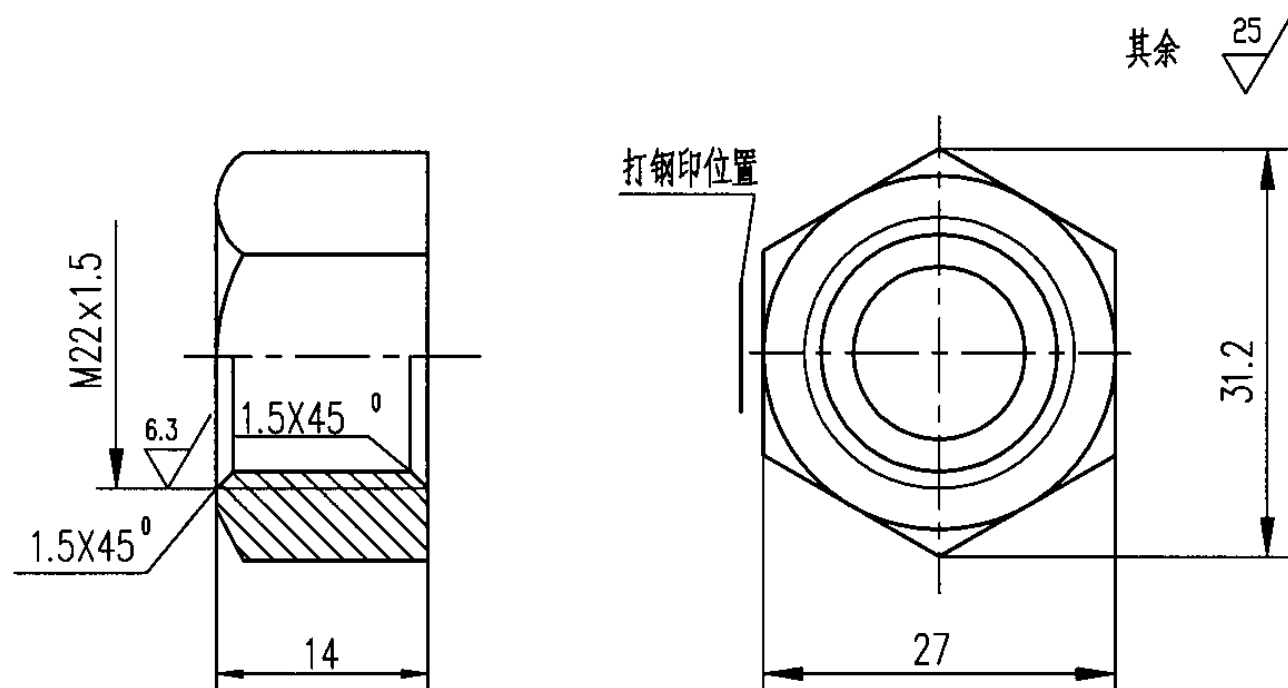
螺母
