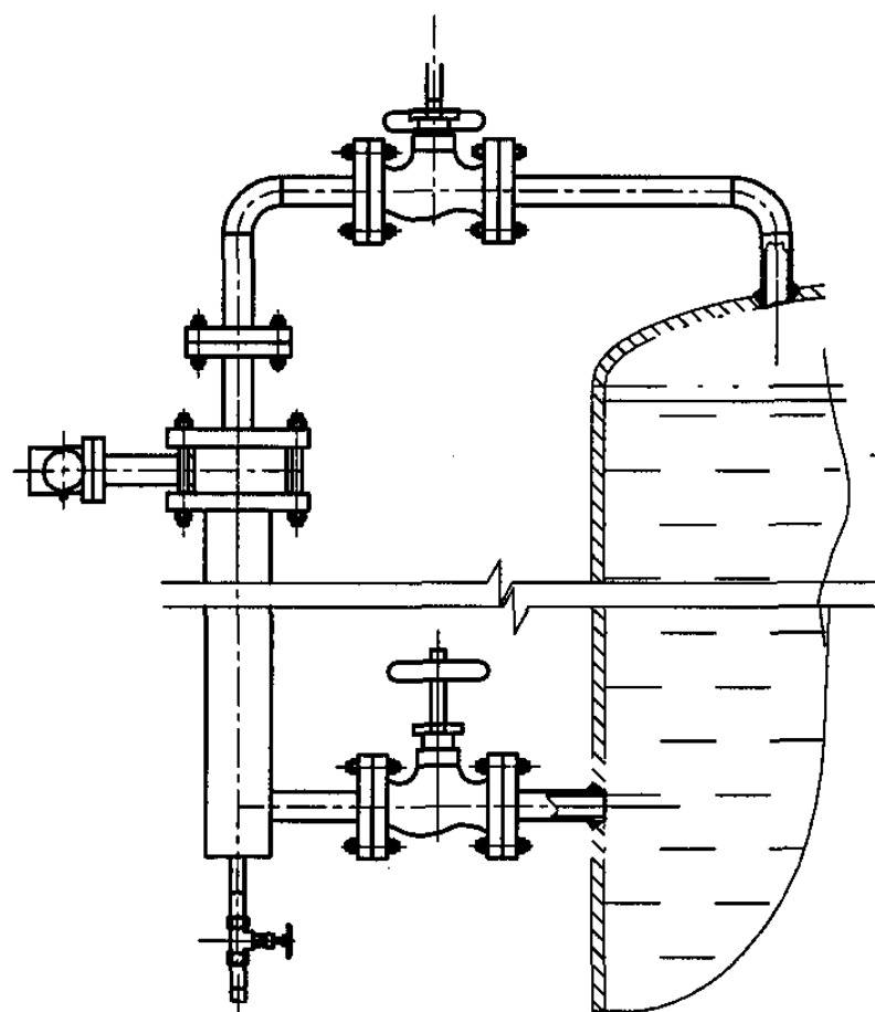
顶侧式安装方案
