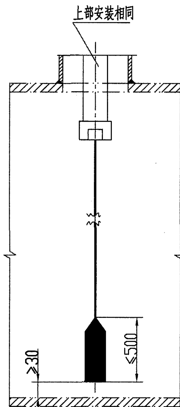
柔性探头顶置式安装方式
