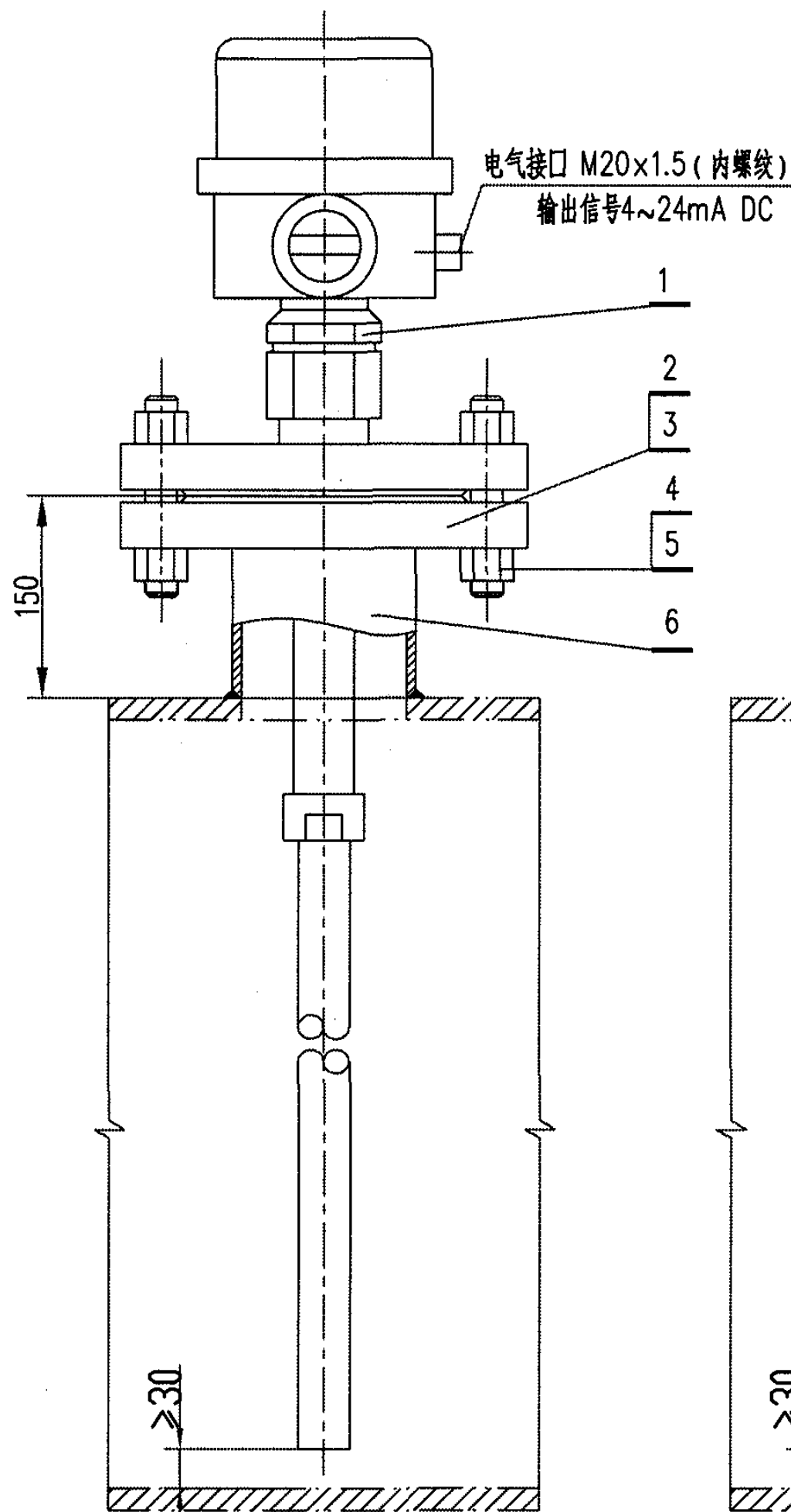
刚性探头顶置式安装方式
