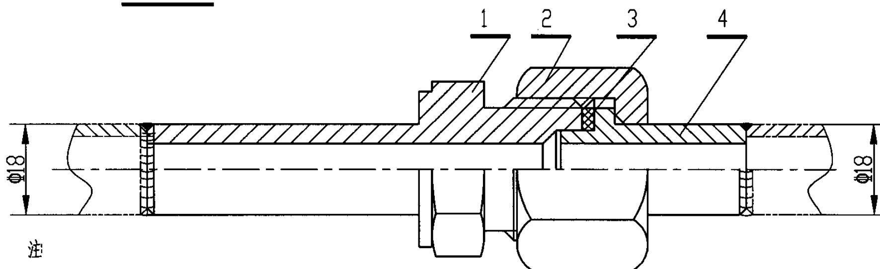
直通中间接头总图
