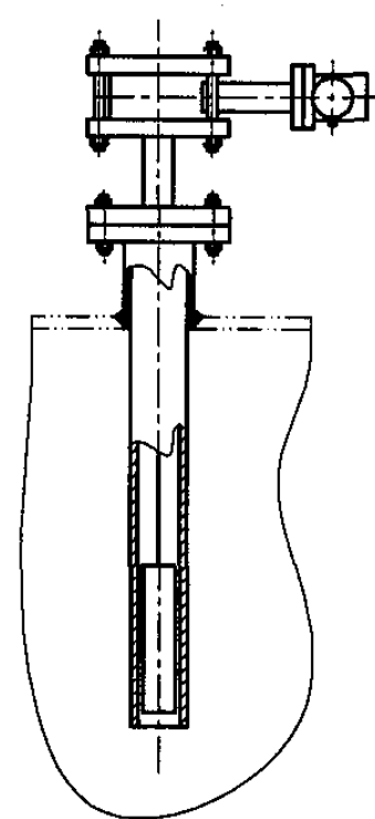
顶置式安装方案(带稳流罩)
