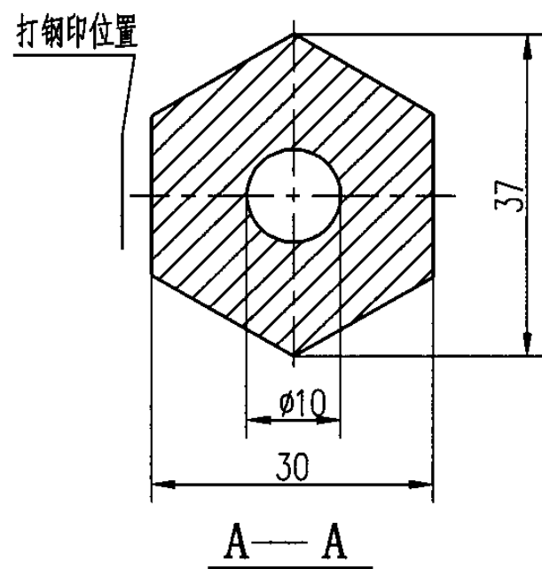
直通中间接头体
