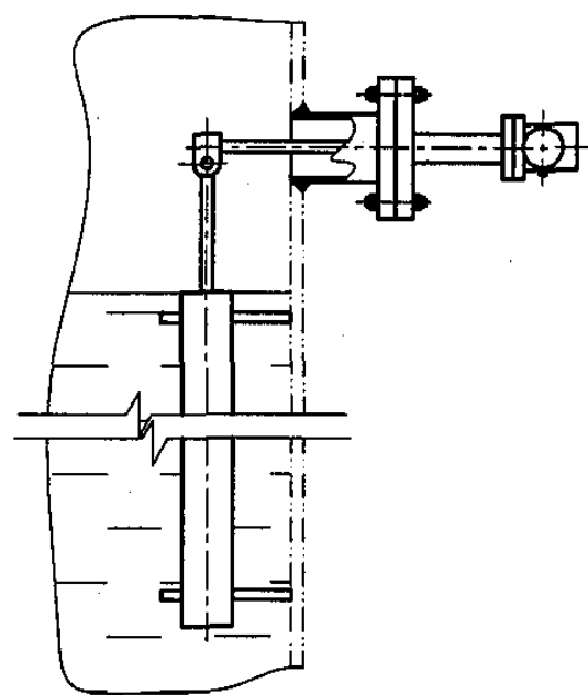
侧置式安装方案(带稳流罩)
