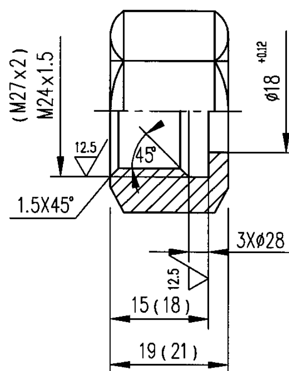
外套螺母 M24×1.5、M27×2
