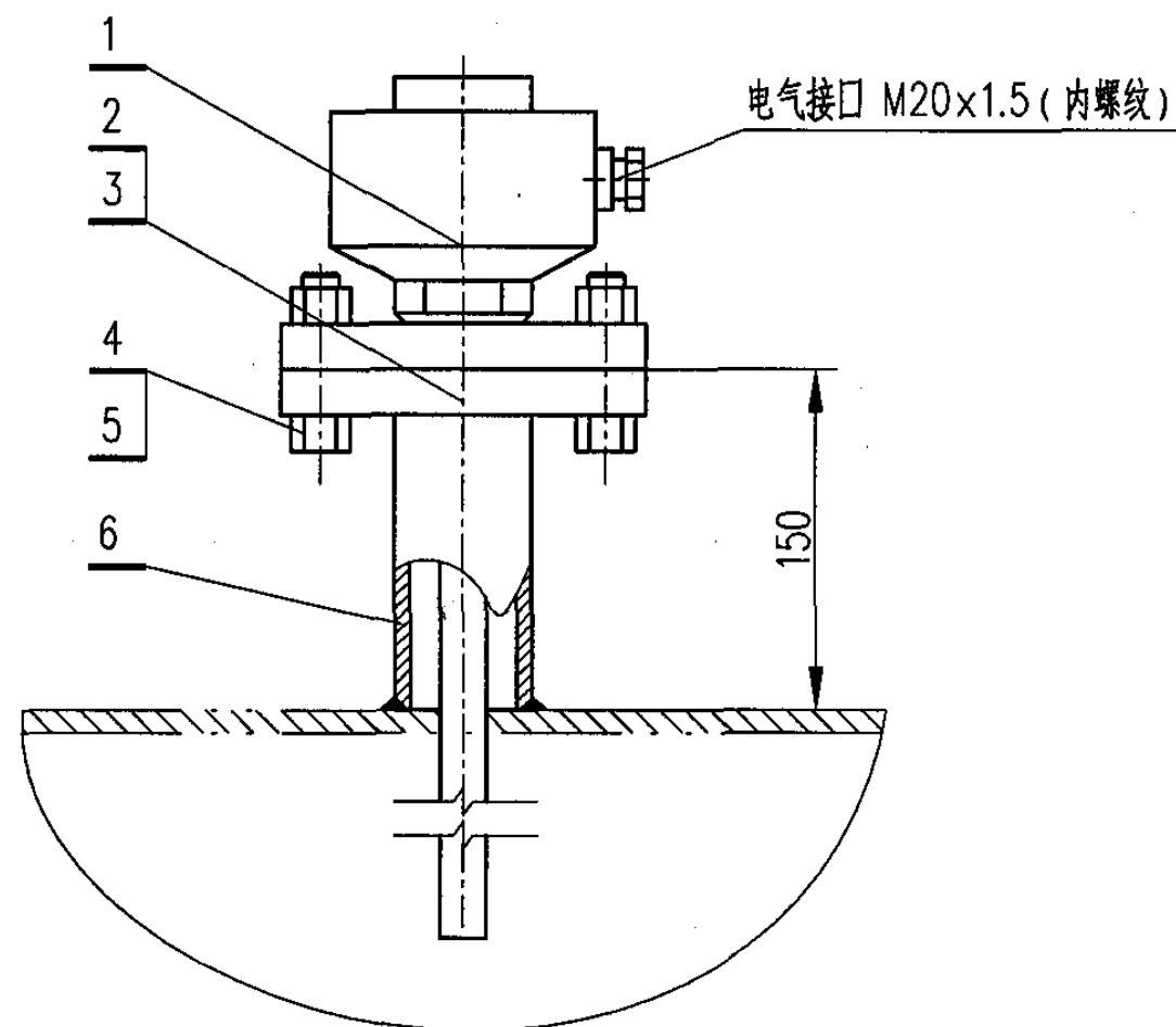
顶部安装方案
