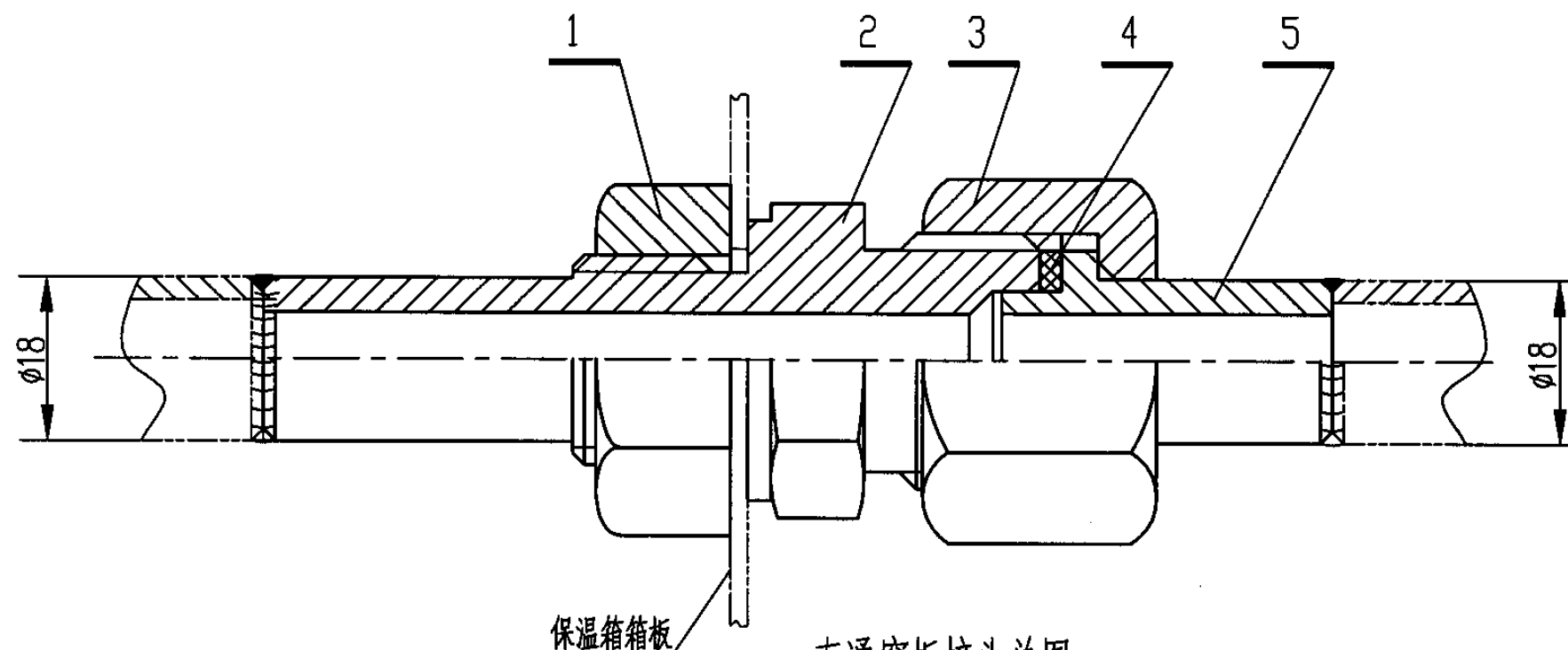
直通穿板接头总图
