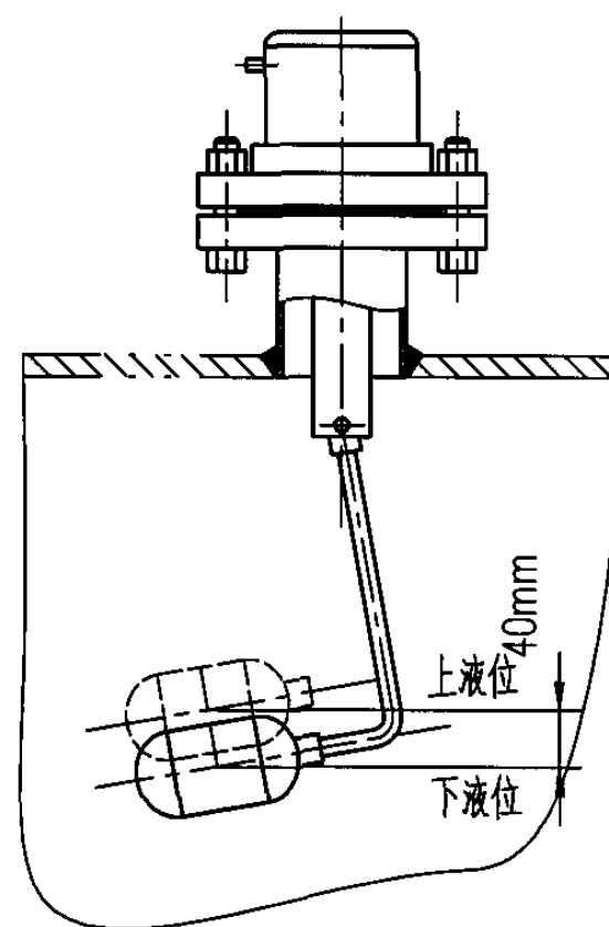
UQK-01T 安装方案
