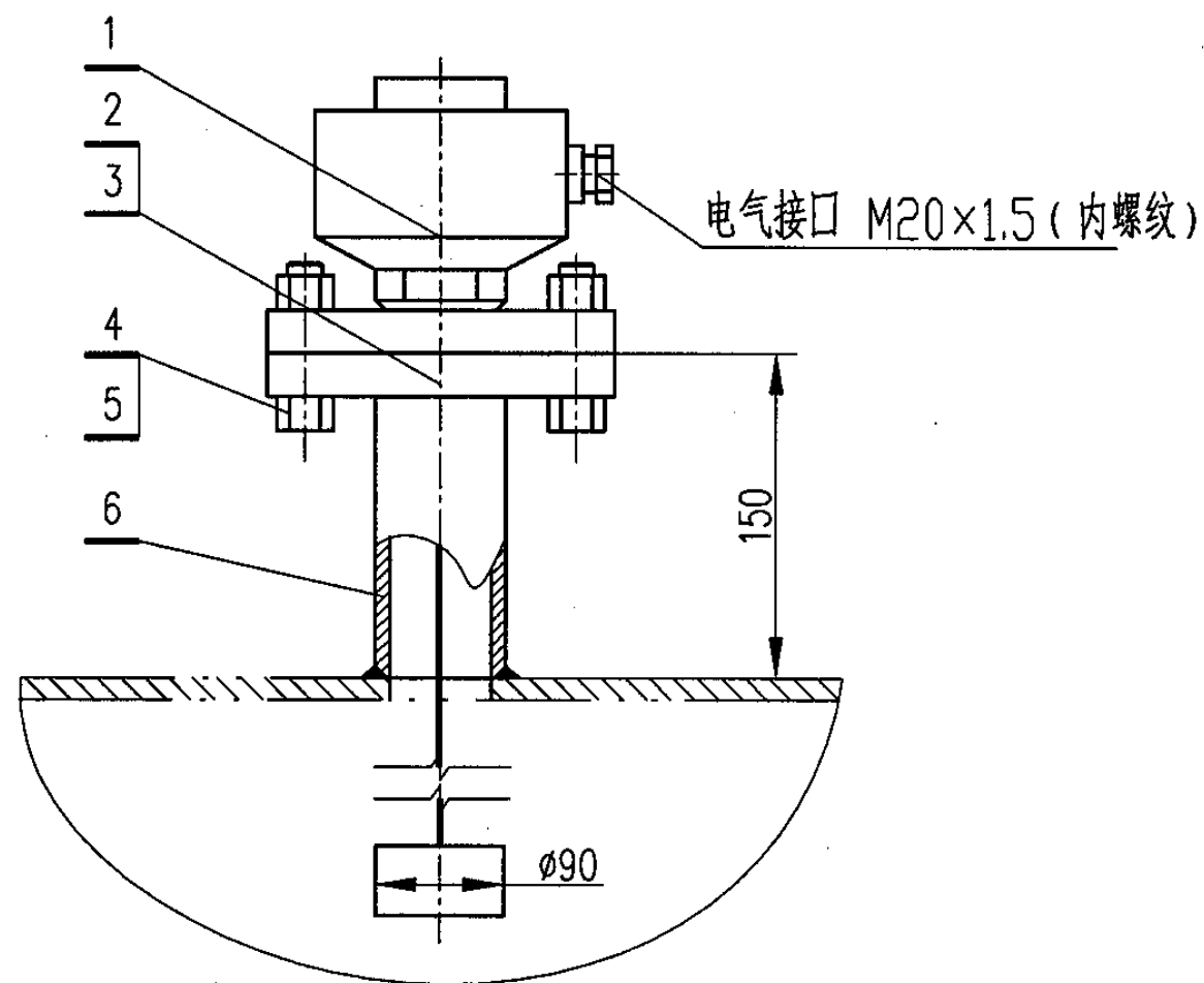
缆式探极安装方案
