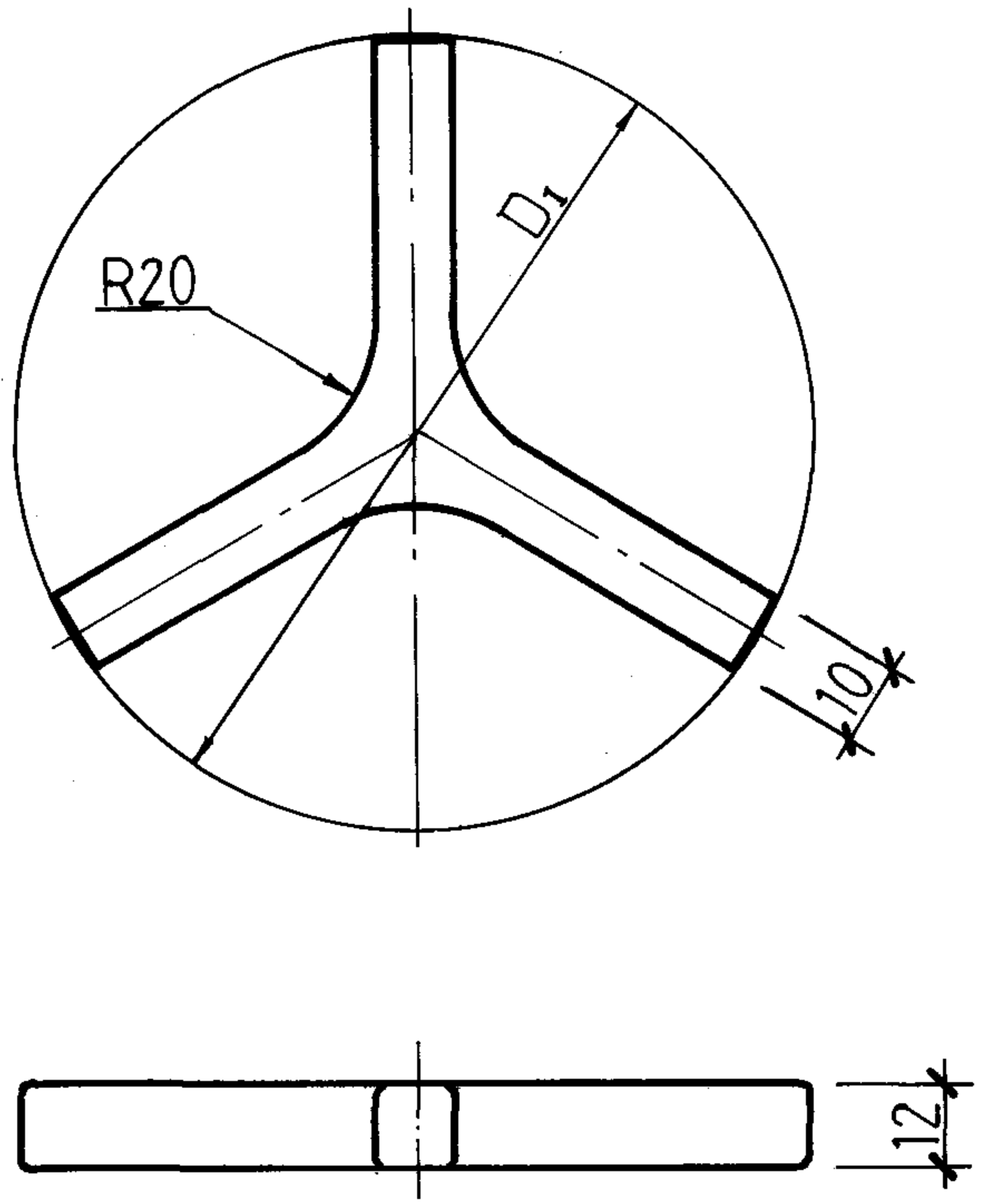
三芯瓷隔板
