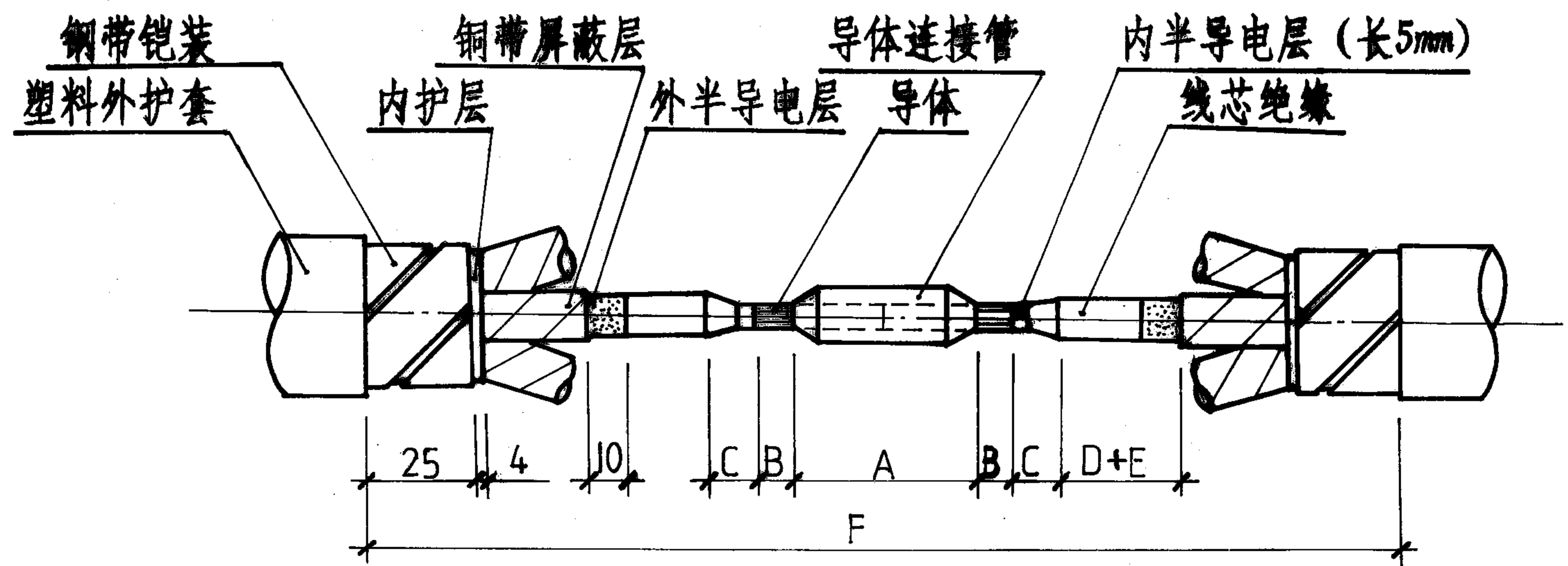
交联聚乙烯电缆剥切尺寸
