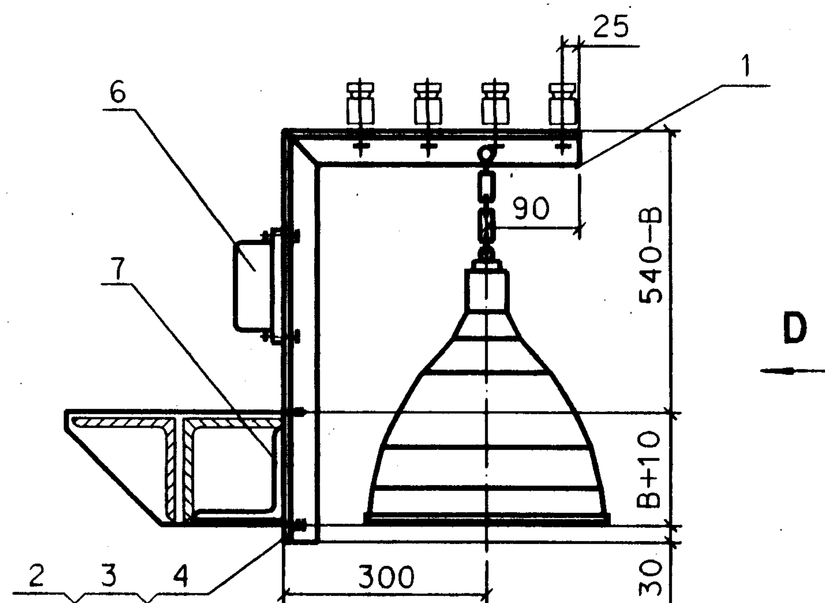
I型(无吊车)
