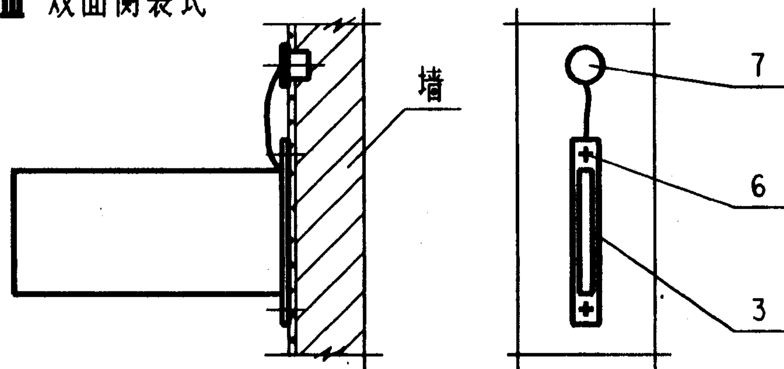
Ⅲ 双面侧装式
