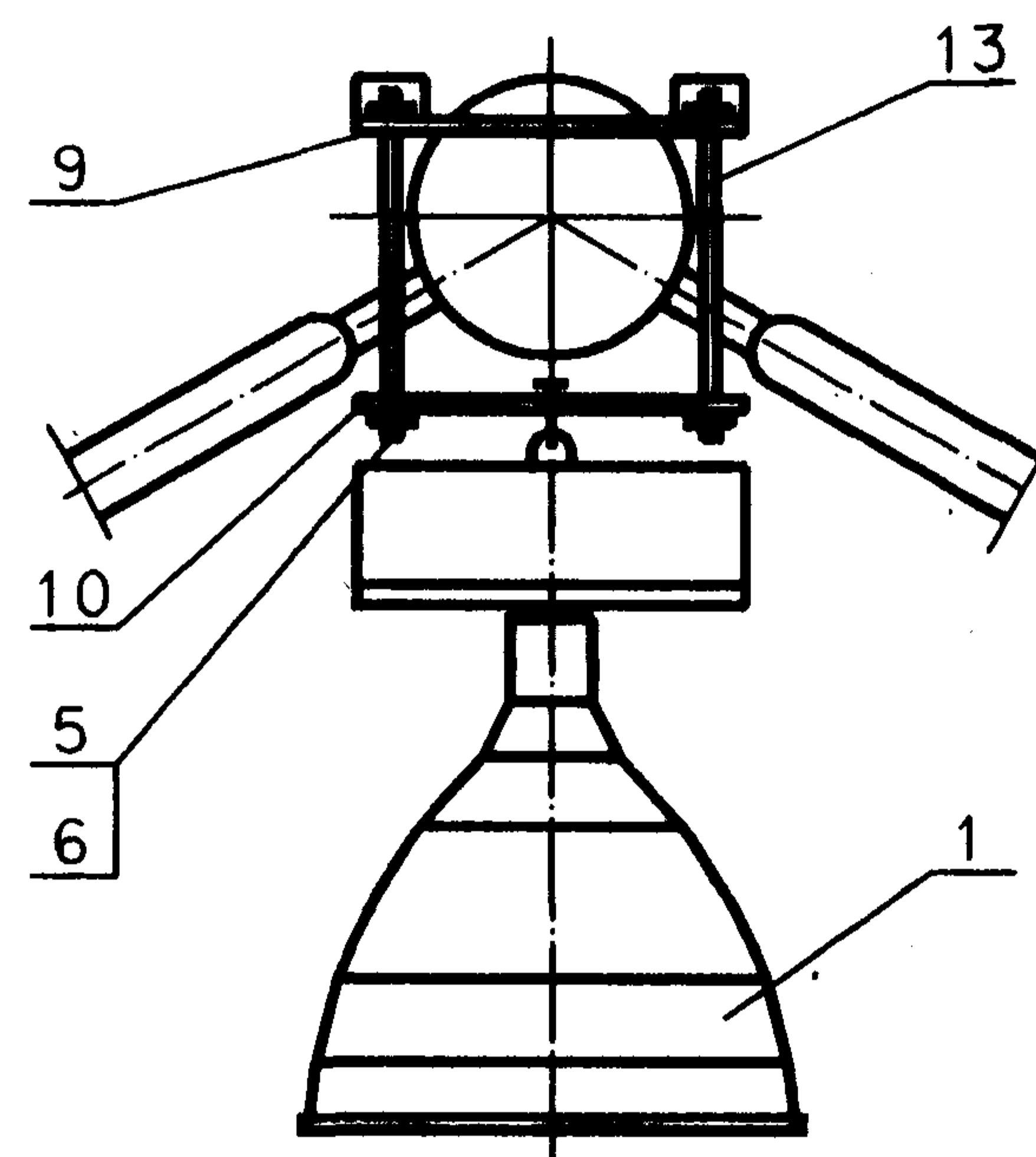
Ⅴ 上球头灯具安装图
