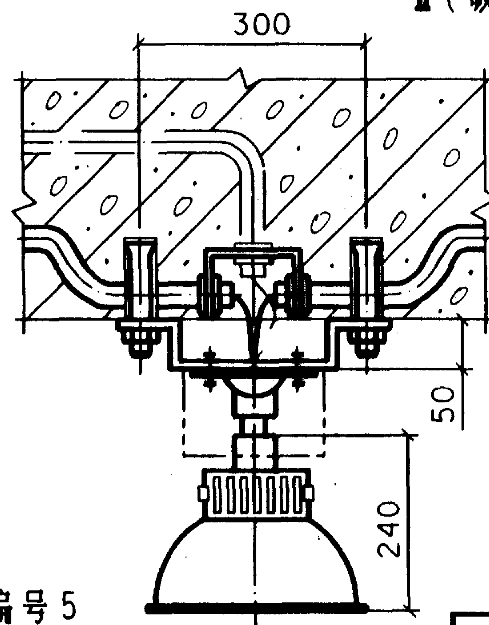
II (吸顶安装)
