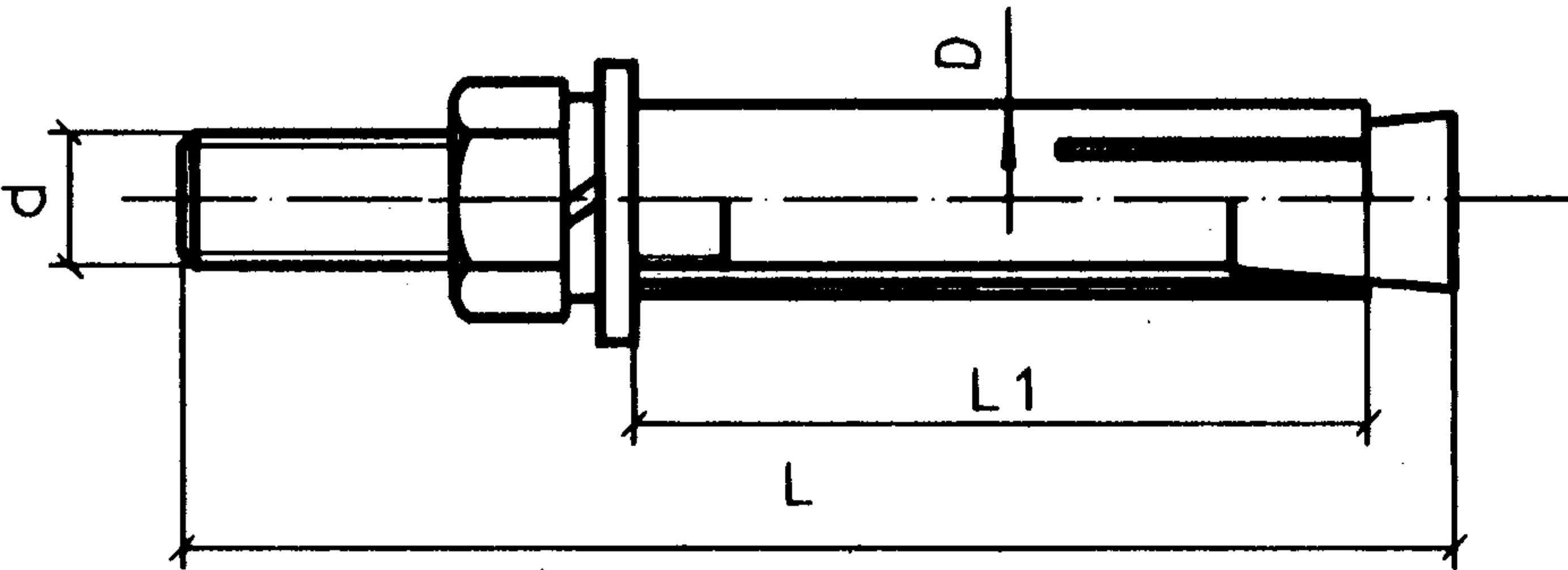
膨胀螺栓
