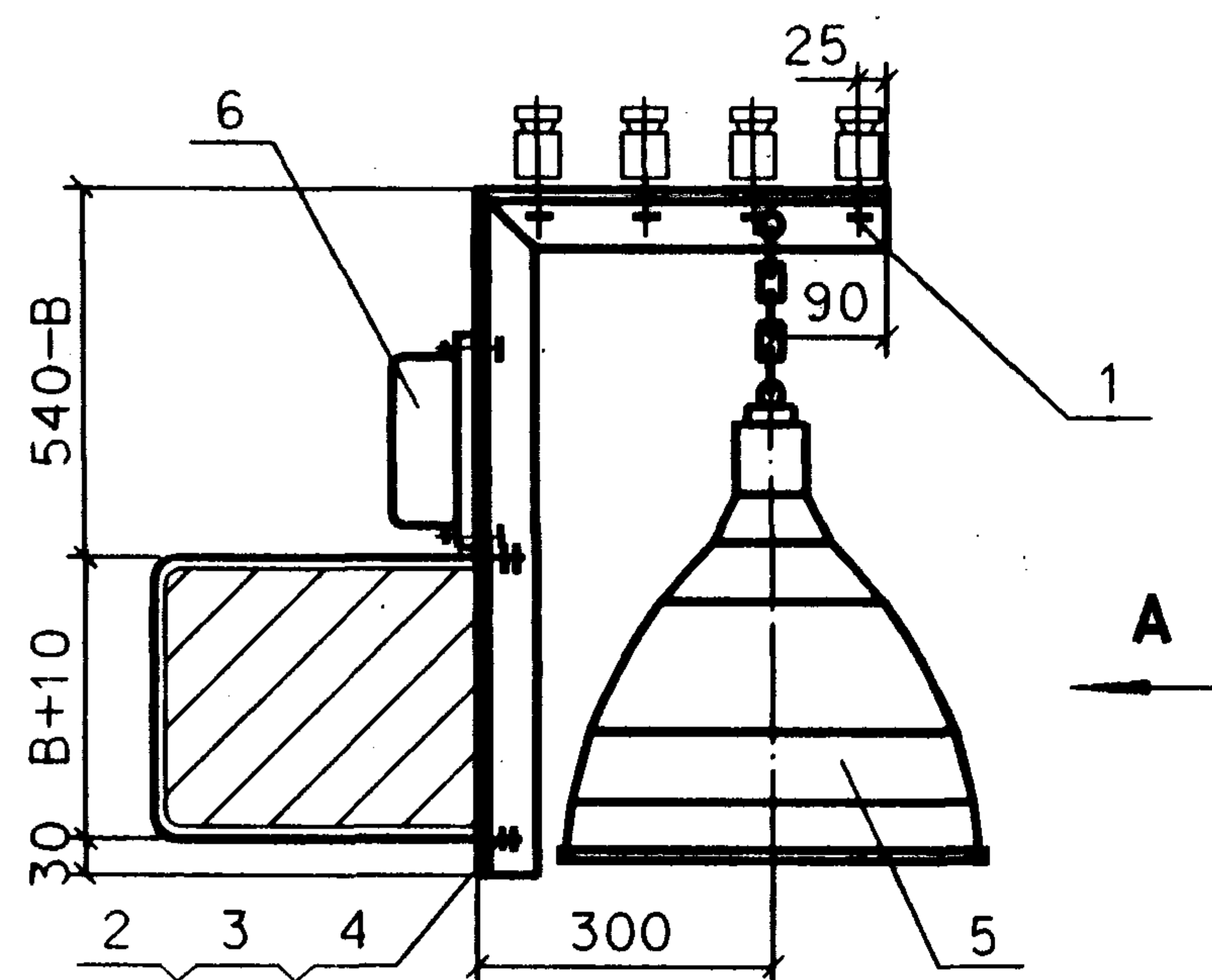
Ⅰ型(有吊车)
