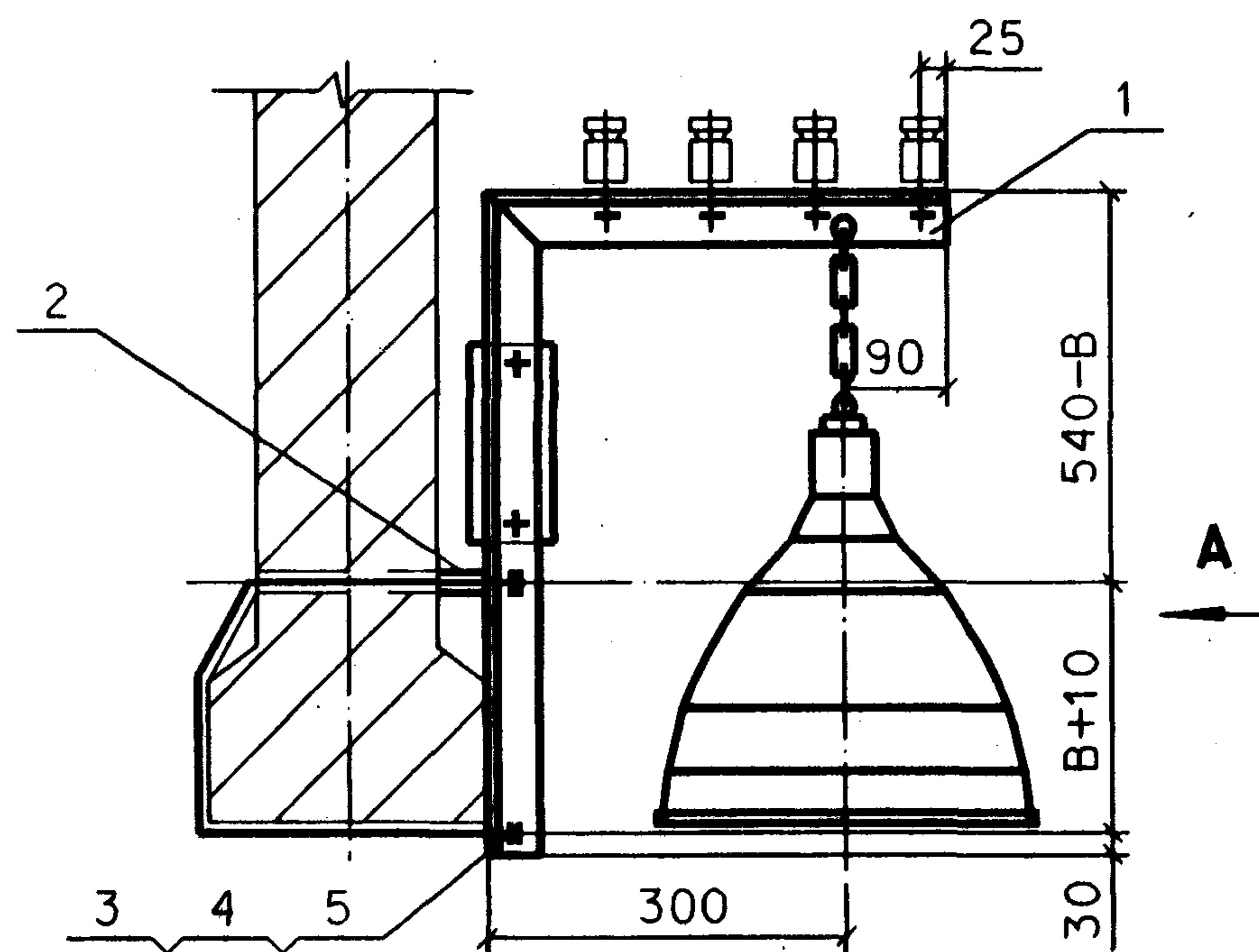
Ⅱ型(有吊车)
