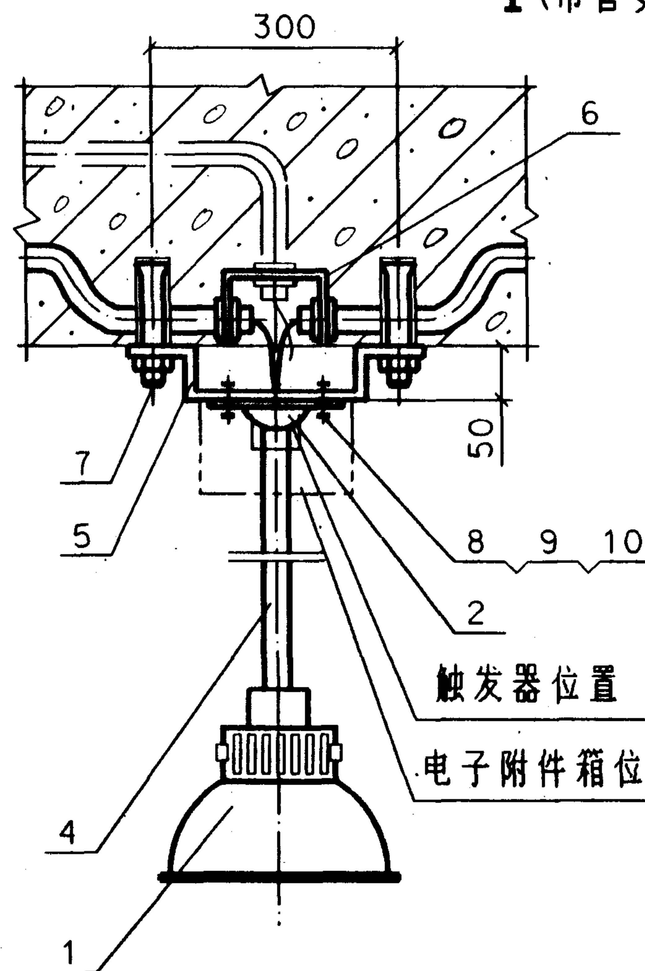
I (吊管安装)
