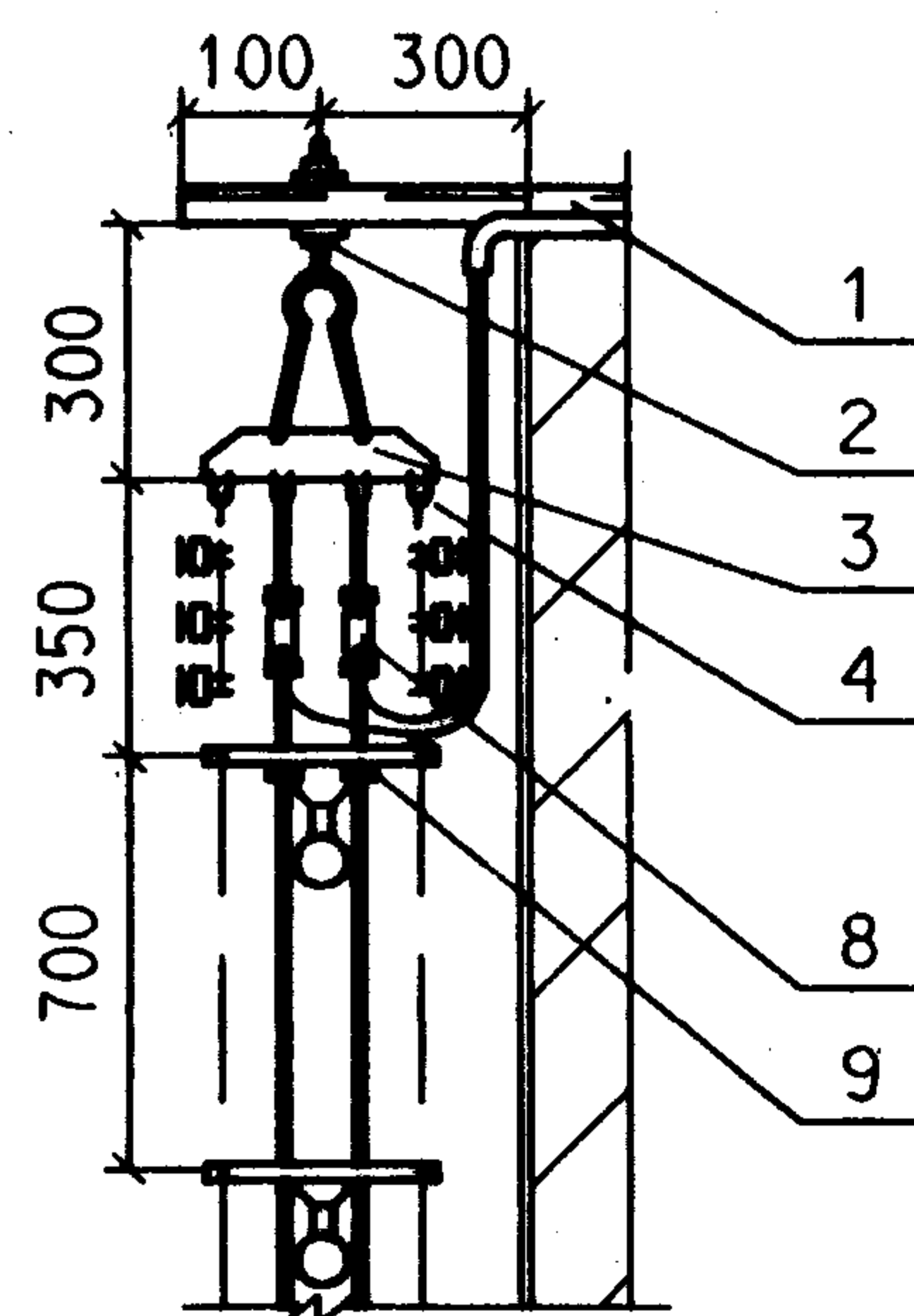
垂直彩灯顶部安装做法
