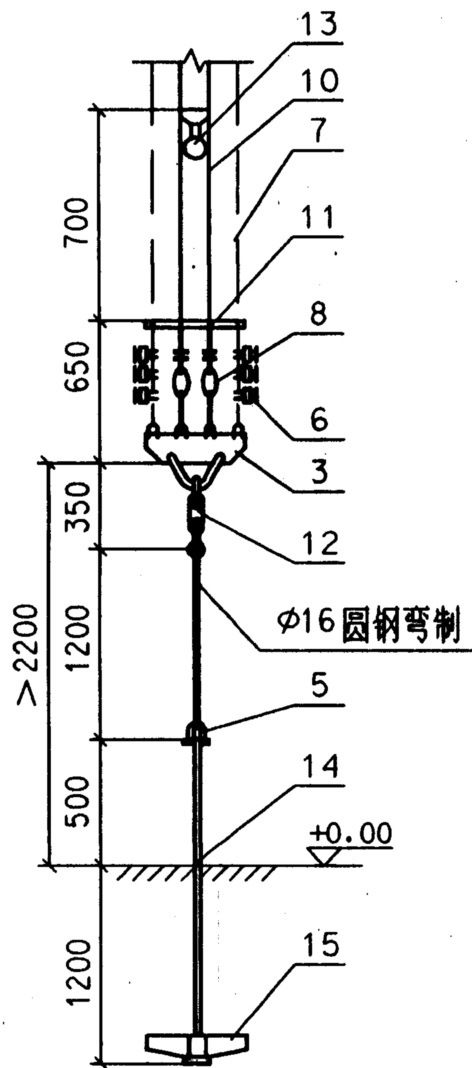
垂直彩灯底部安装做法
