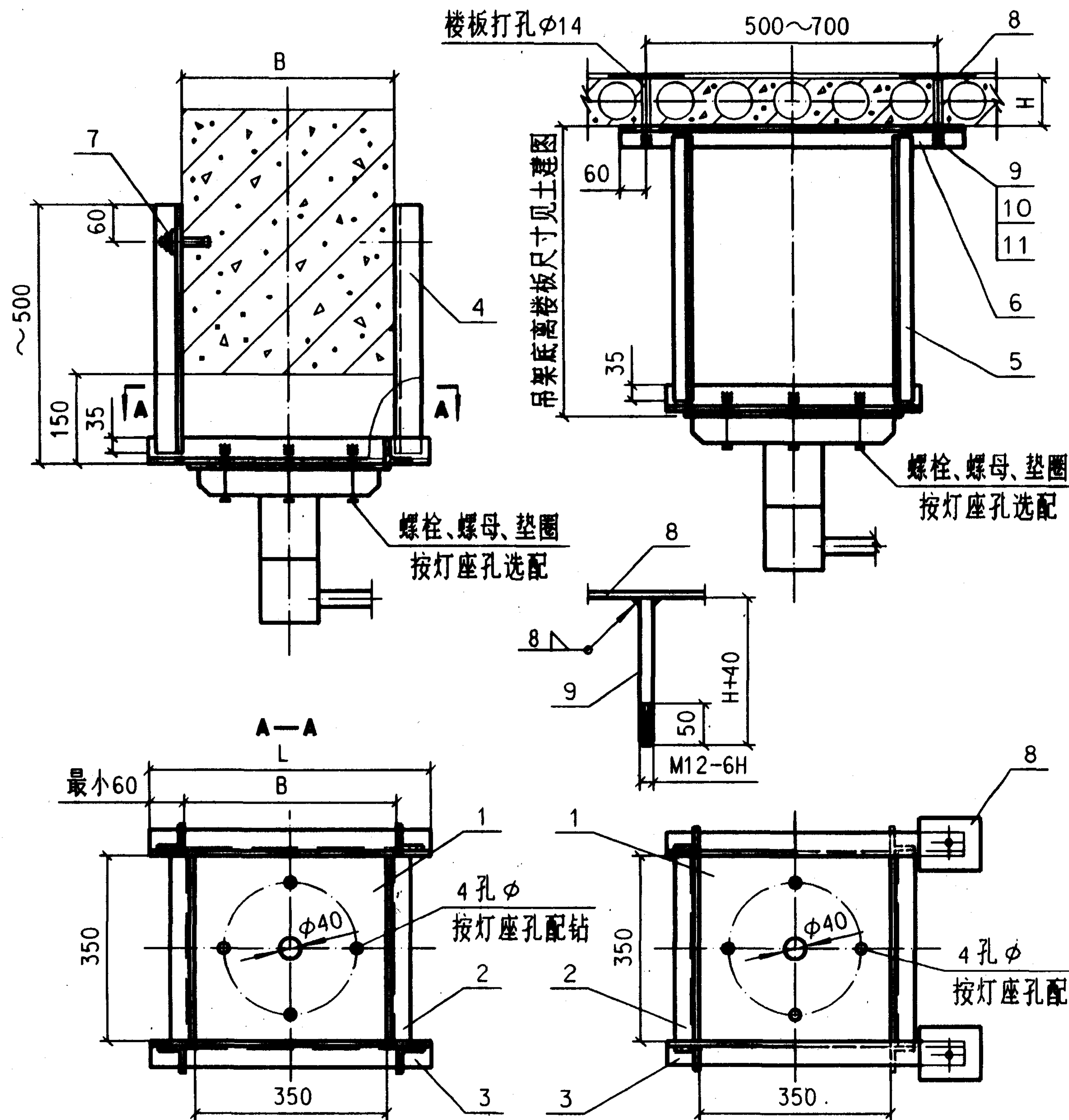
方案 I (预制梁上安装)
