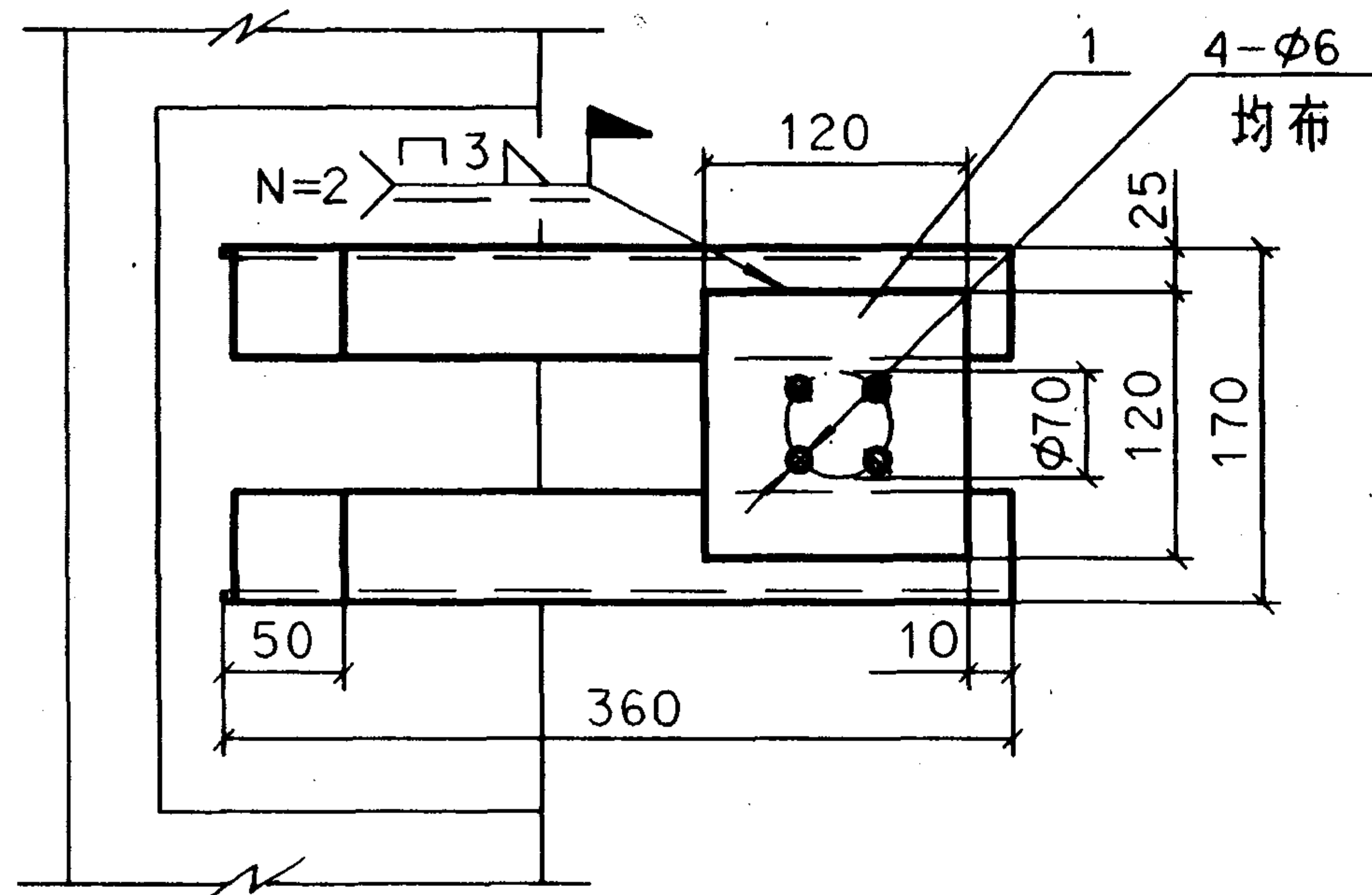
编号 1, 2 零件焊接图
