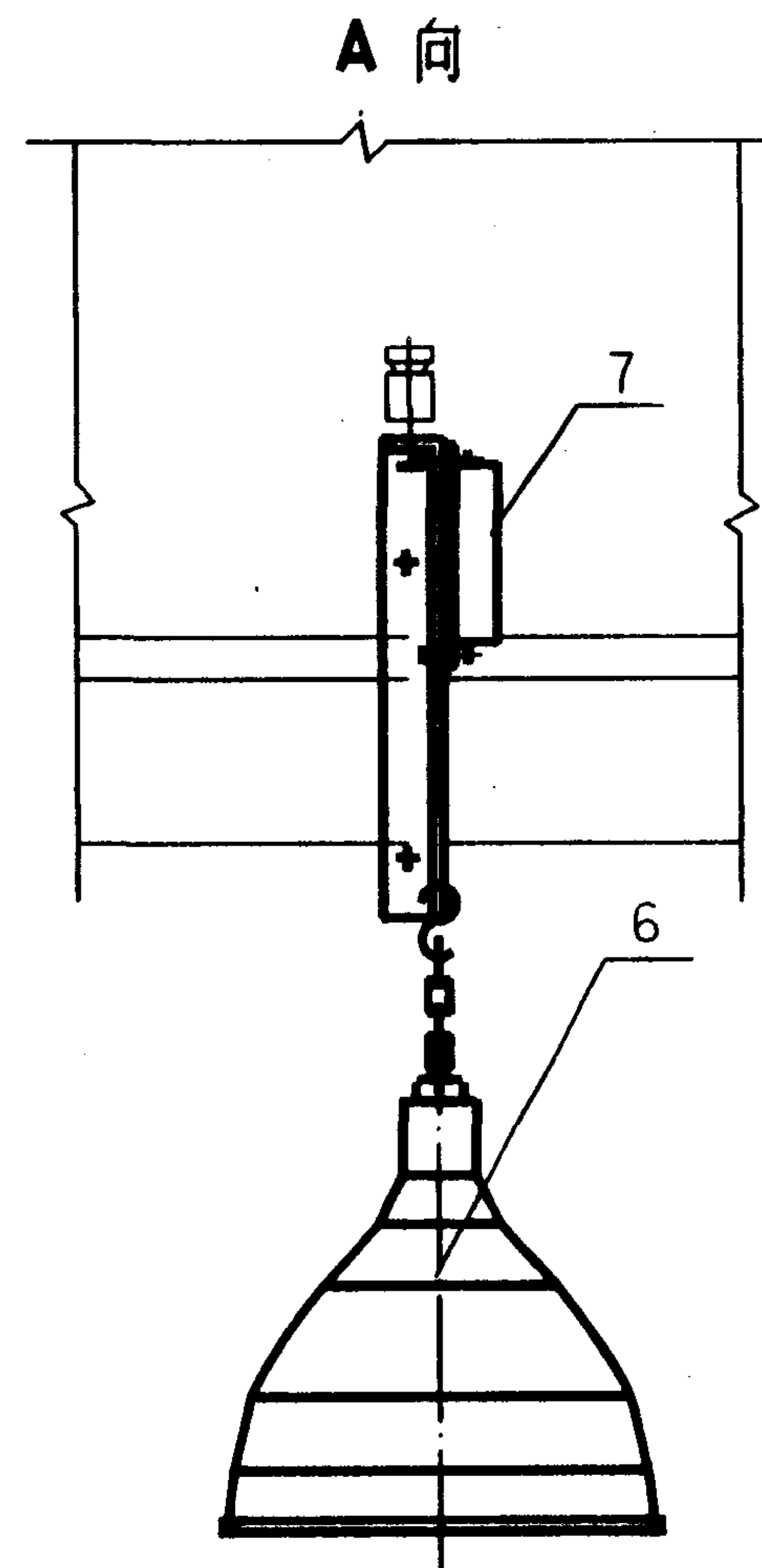
Ⅰ型(无吊车)
