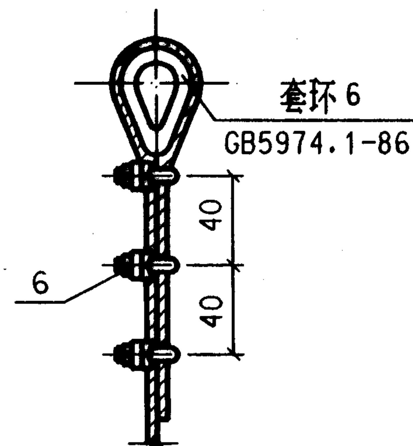
钢丝绳端头夹紧法
