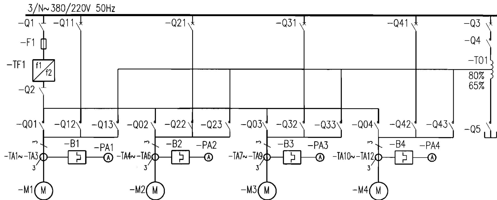
—变频调节三用一备泵(补偿起动)概略图
