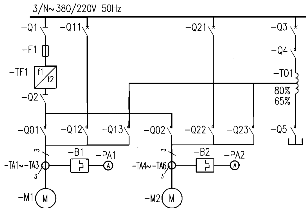
—变频调节一用一备泵(补偿起动)概略图
