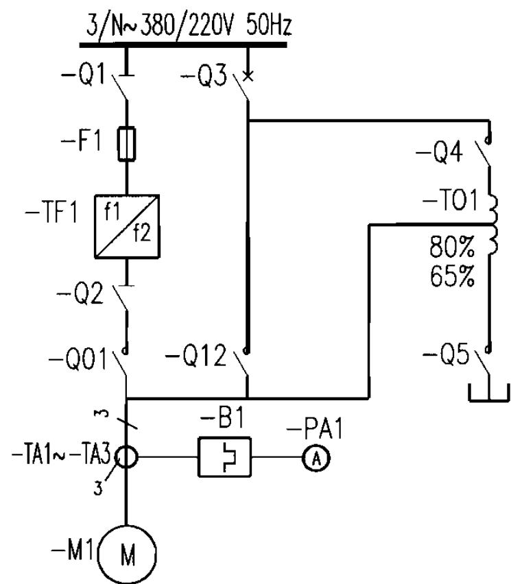
—变频调节一泵(补偿起动)概略图
