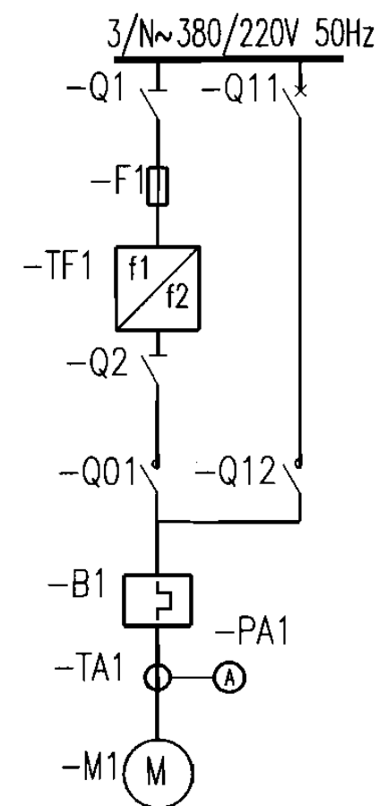
一变频调节一泵(直起)概略图
