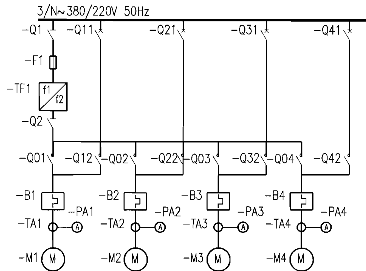
一变频调节三用一备泵(直起)概略图
