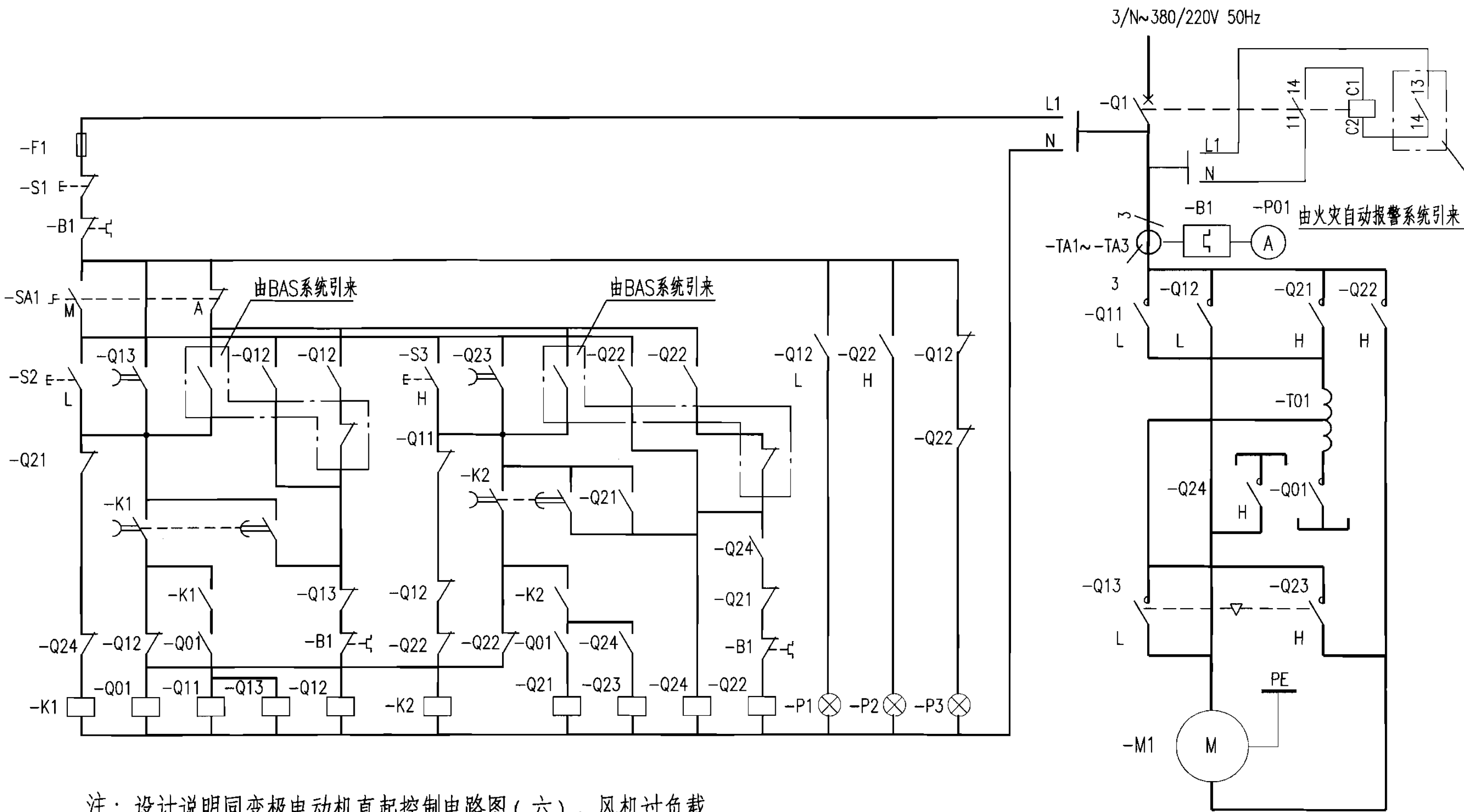
变极电动机自耦降压起动电路图（三）
