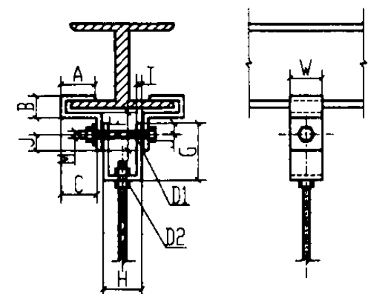
HKI型吊具
