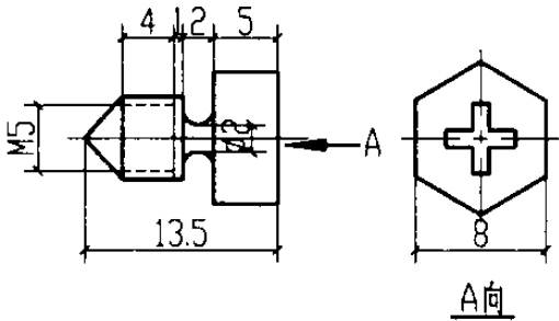
紧定螺钉 I
