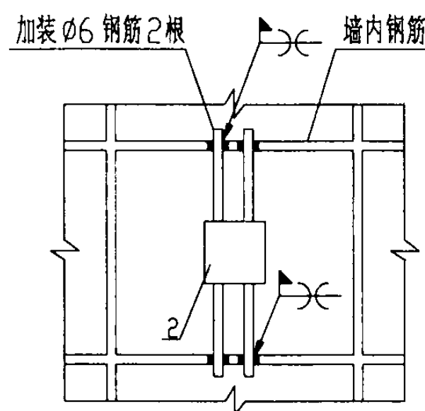
弓型支撑板在钢筋网上加固处理
