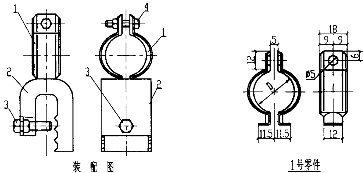
托盘管卡规格、尺寸
