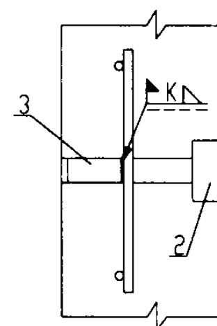
弓型支撑板在钢筋网上加固处理
