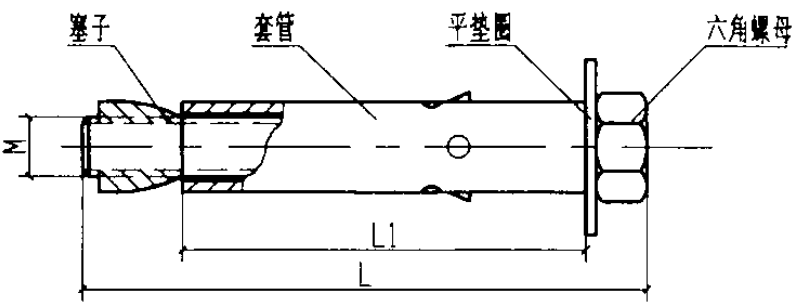
SHFA型扭转式平头胀锚螺栓
