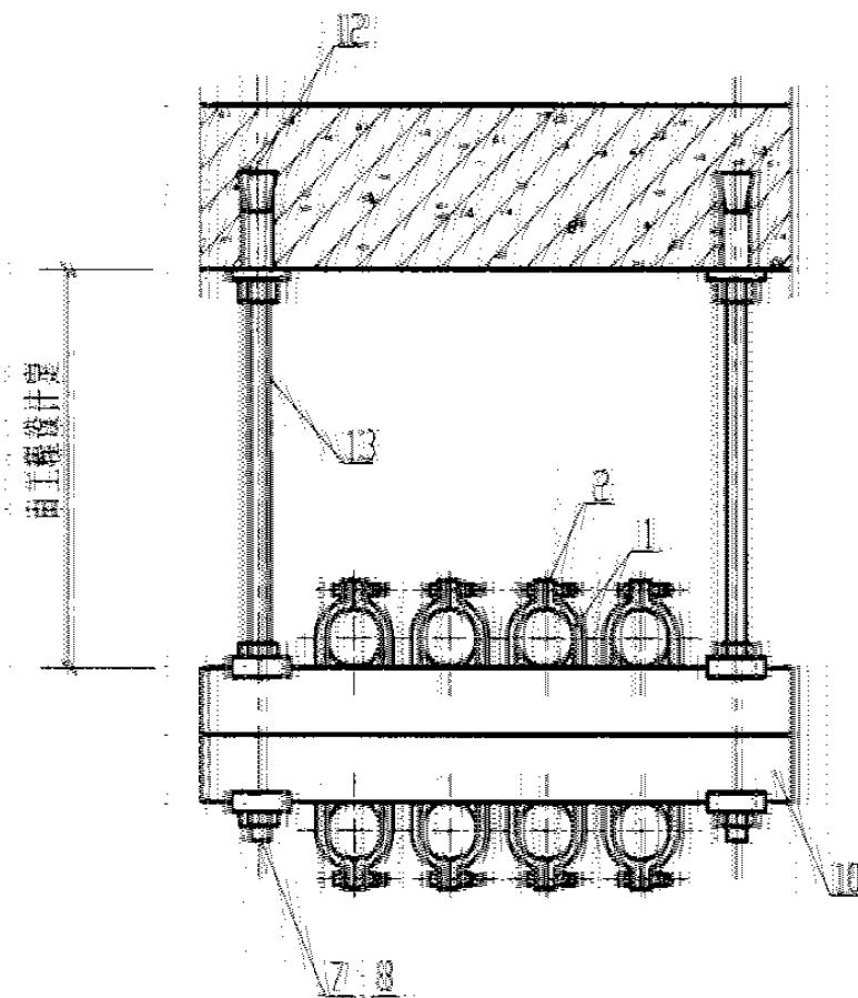
III 在吊架上敷设
