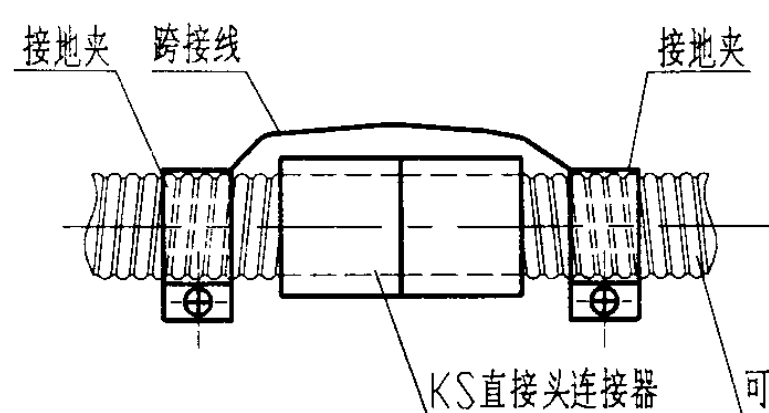
可挠金属电线保护管连接
