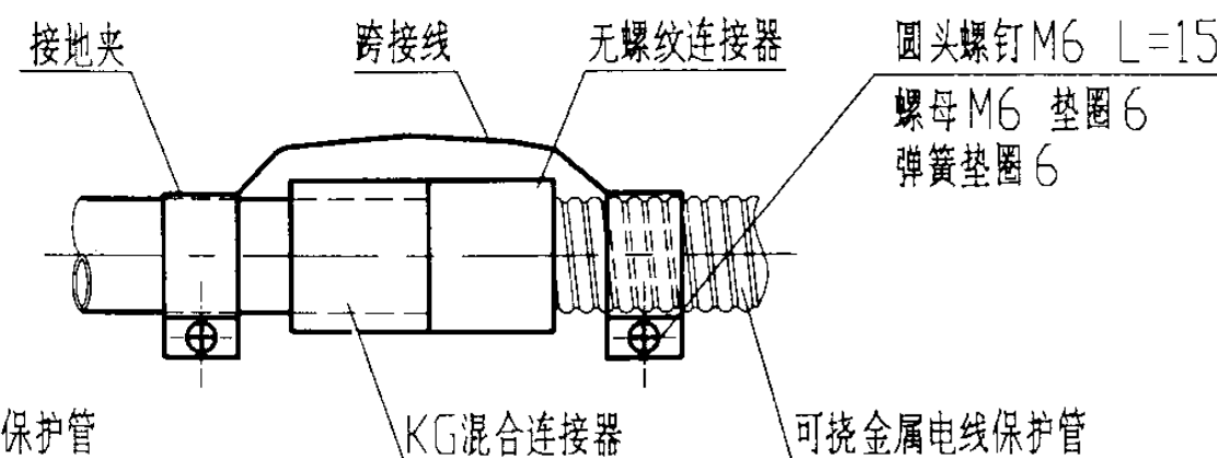
可挠金属电线保护管与钢管连接
