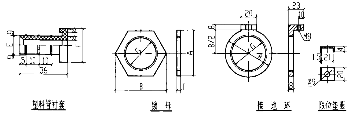
锁母规格、尺寸
