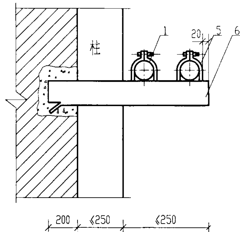
II 沿墙跨柱敷设
