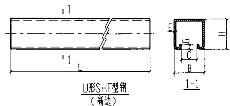
U形SHF型钢规格, 尺寸(高边)
