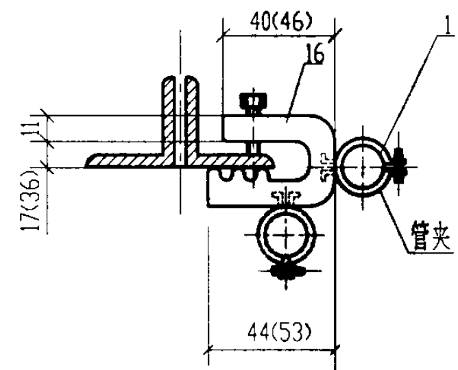
III 沿屋架下弦侧敷设
