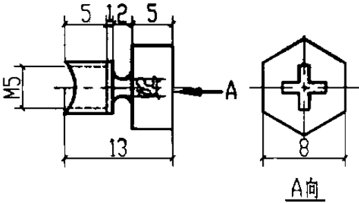
紧定螺钉 II
