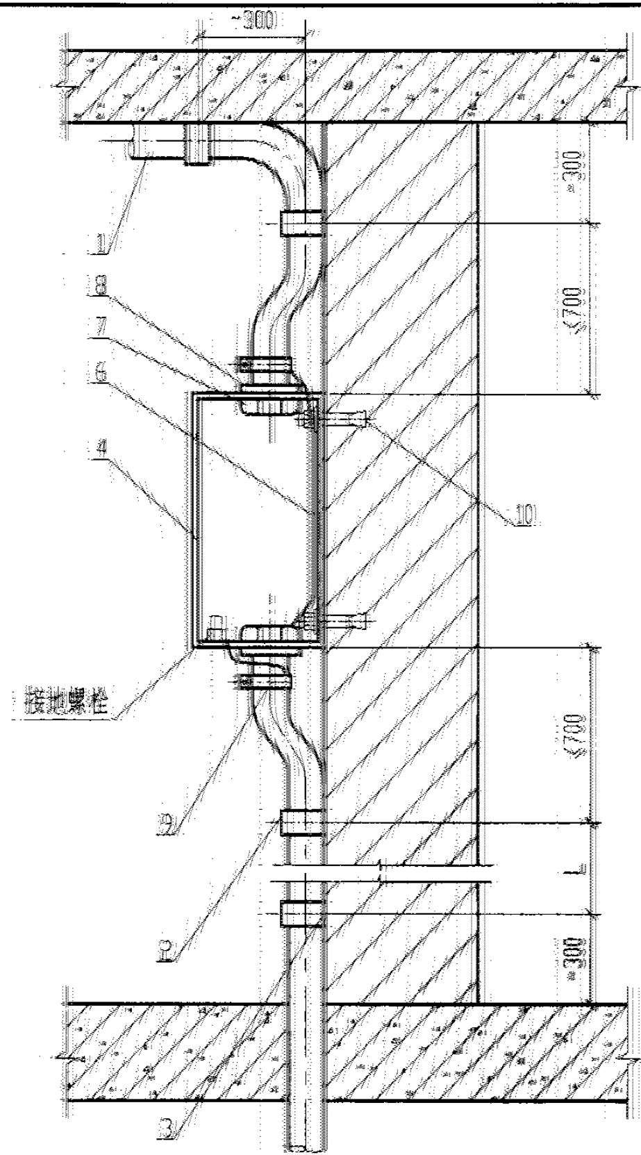
挂墙式配电装置明管进出安装
