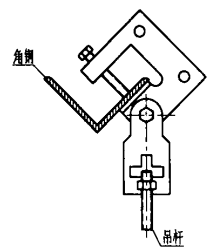
KH型万向吊架40kg 配置立面图
