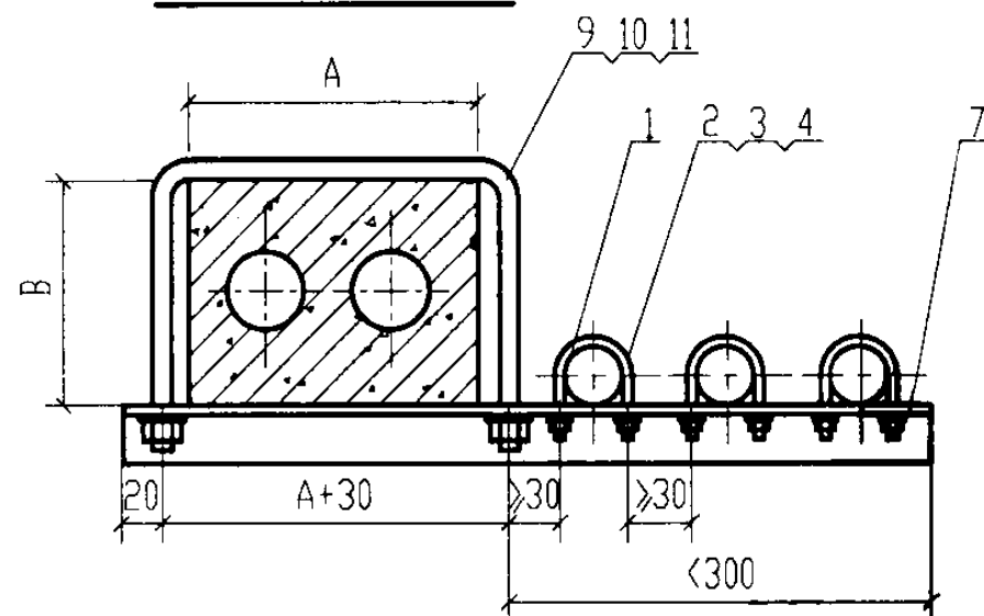
II 沿屋架下弦侧敷设
