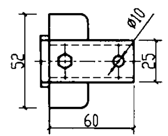
KH型万向吊架
