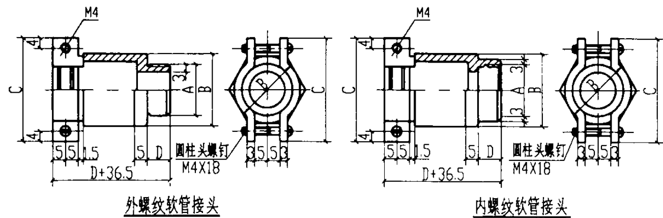
内、外螺纹软管接头规格、尺寸
