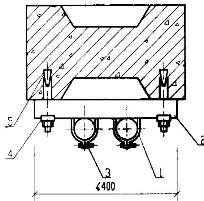
II 沿柱垂直敷设
