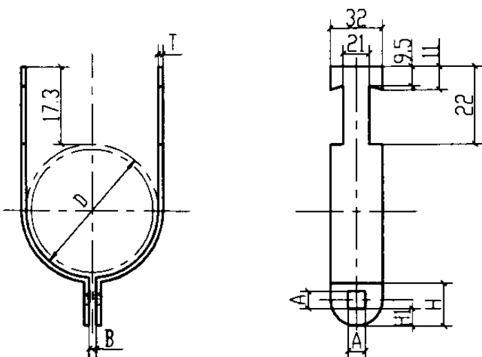
U型SHF管卡
