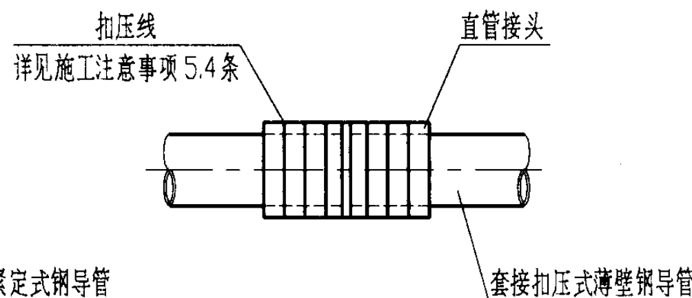
套接扣压式薄壁钢导管扣压连接
