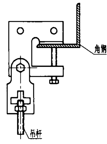
KH型万向吊架100kg 配置立面图
