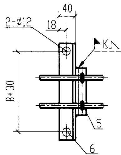
A向
