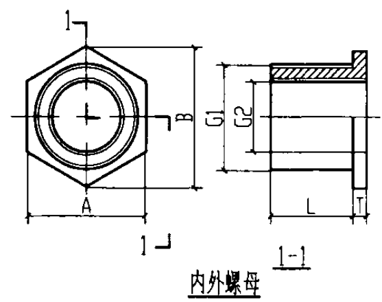
内外螺母规格、尺寸
