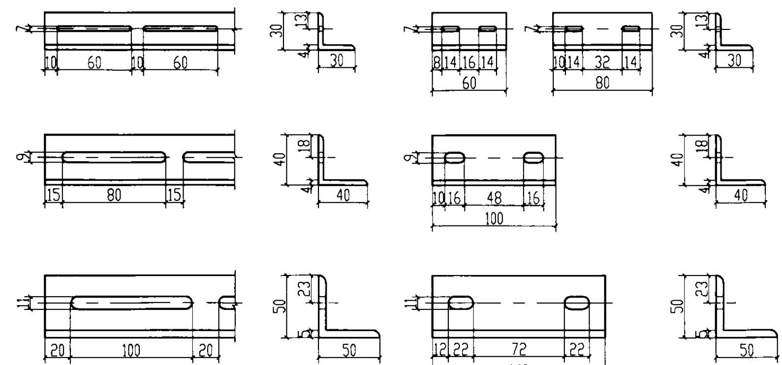
多管角钢支架
