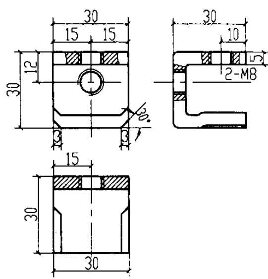
1号零件
