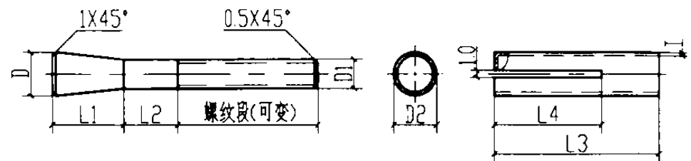
胀锚螺栓
