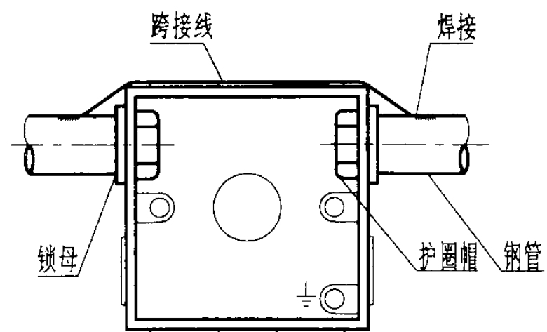
钢管与接线盒连接
