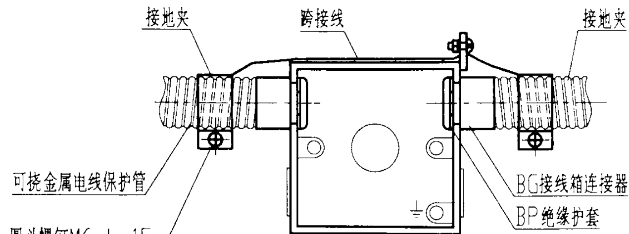
可挠金属电线保护管与接线盒连接
