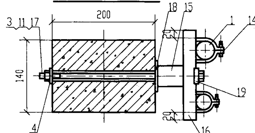
IV 沿屋架下弦侧敷设
