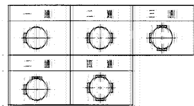
圆形接线盒形式
