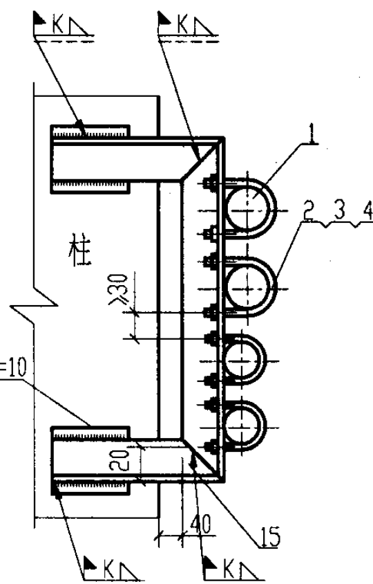
IV 跨柱水平排列敷设
