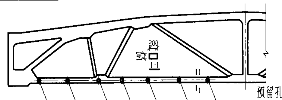
95G314 钢筋混凝土折线形屋架外形图
