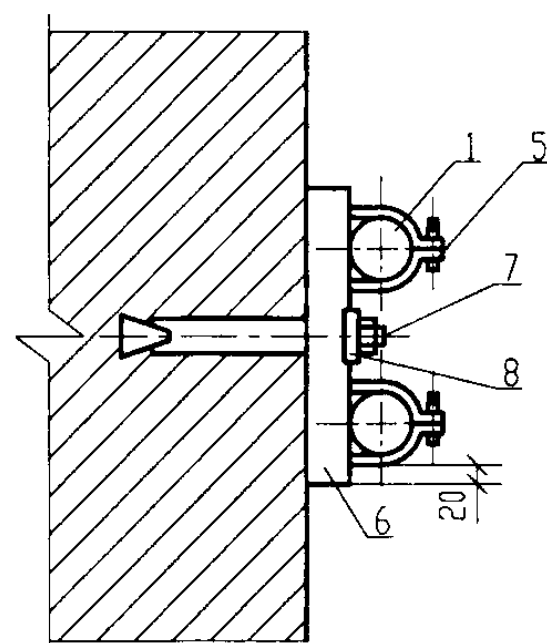
I 沿墙敷设
