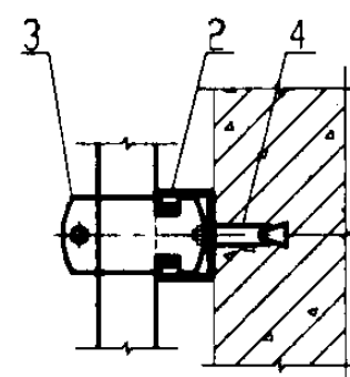
甲详图
