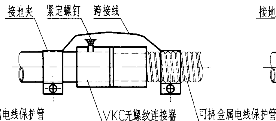
可挠金属电线保护管与钢管连接
