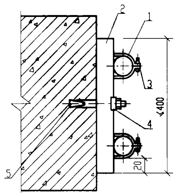
V 跨柱水平排列敷设
