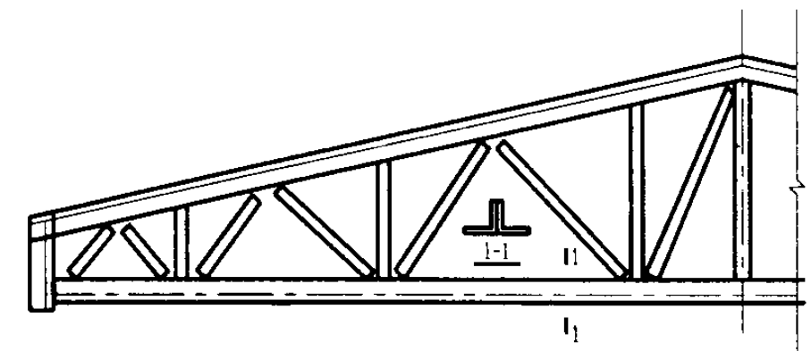
97G511 钢屋架外形图
