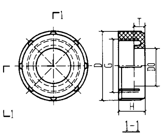
护圈帽规格, 尺寸
