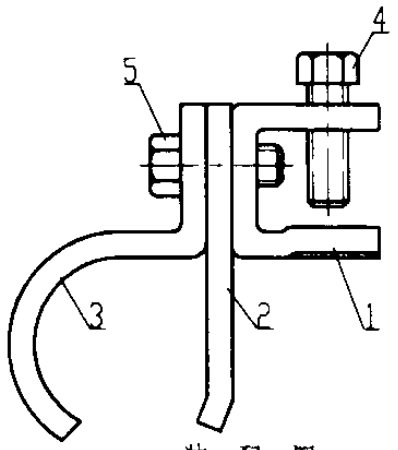
装配图
