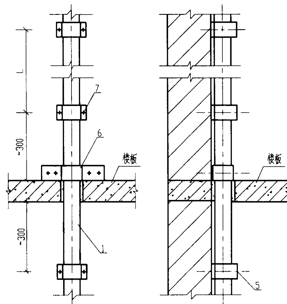
II 单管沿墙敷设
