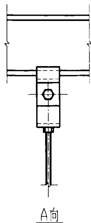
I沿轻钢结构钢梁吊杆敷设
