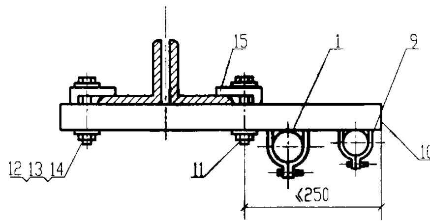
II 沿屋架下弦侧敷设
