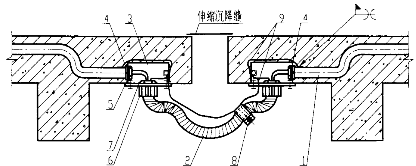
II 沿楼板过伸缩沉降缝敷设
