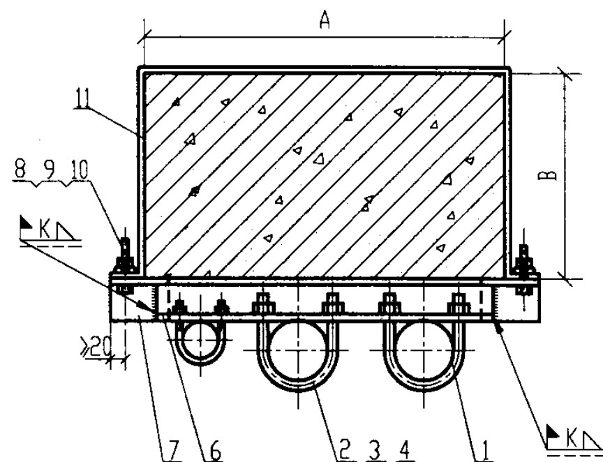
II 沿柱垂直敷设
