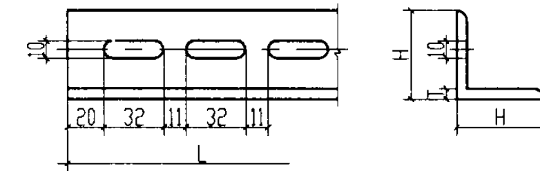
角钢支架(AGH)
