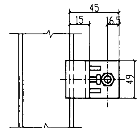
C型钢吊架
