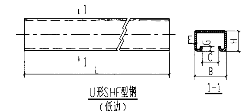
U形SHF型钢规格, 尺寸(低边)
