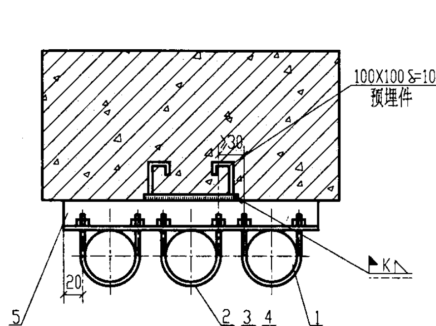
I 沿柱垂直敷设
