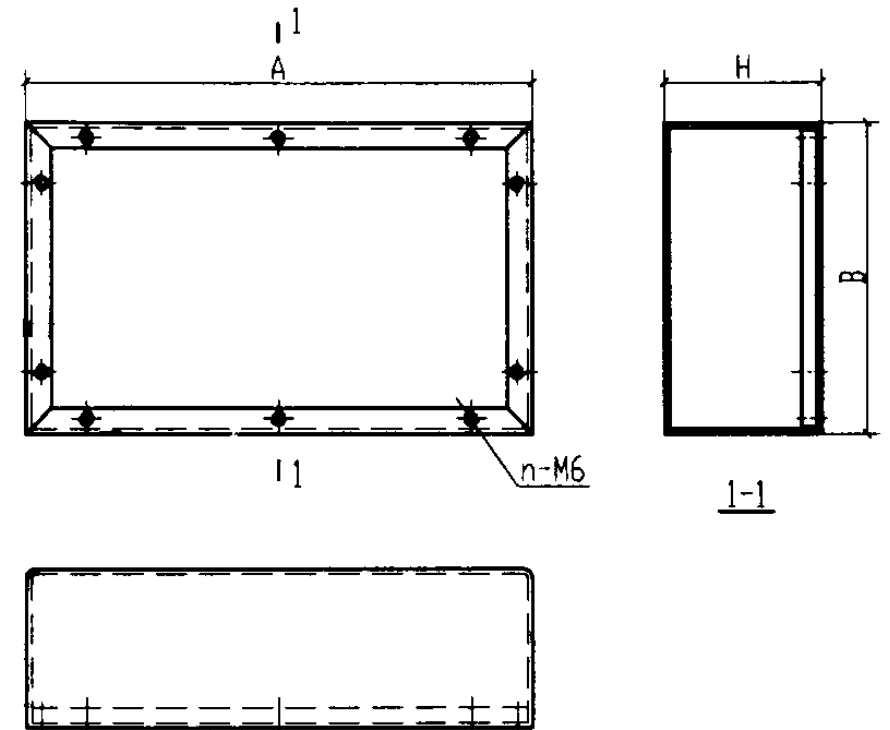
5~8号拉线箱
