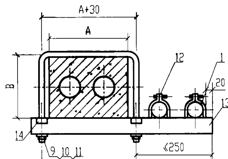
IV 沿屋架下弦侧敷设
