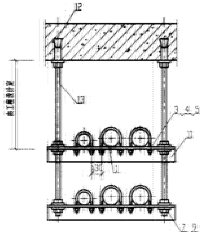
IV 在吊架上敷设
