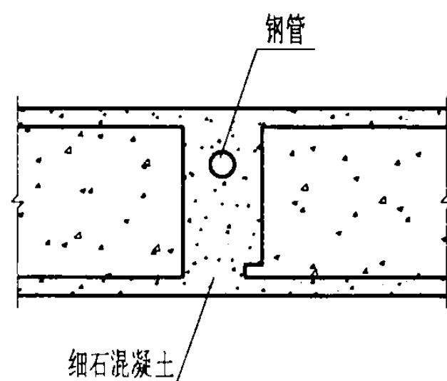
沿加气混凝土板板缝内敷设
