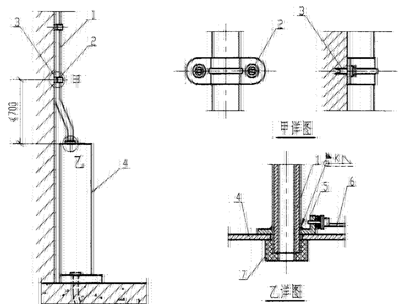
落地式配电装置明管进出安装
