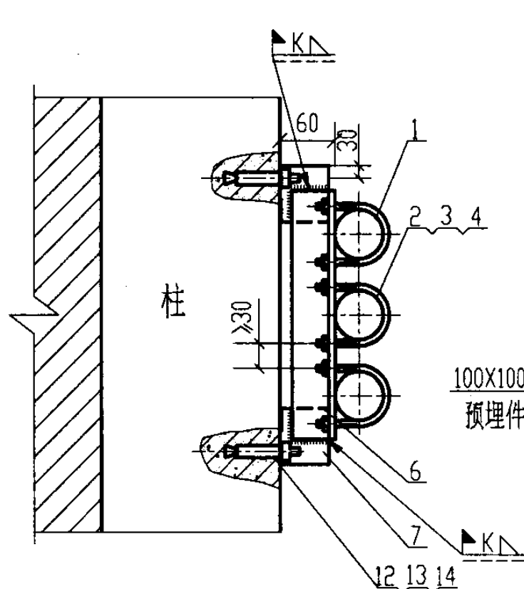
III 跨柱水平排列敷设
