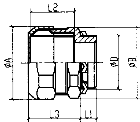
WBG防水型接线箱连接器规格、尺寸
