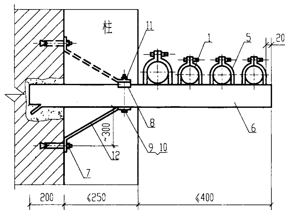
IV 沿墙跨柱敷设
