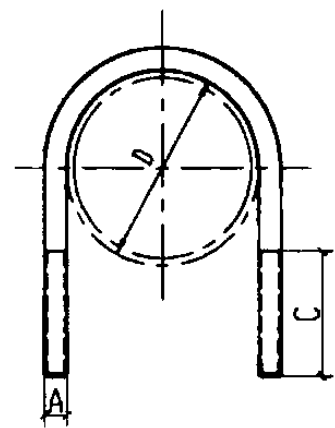
U型SHF螺丝管卡
