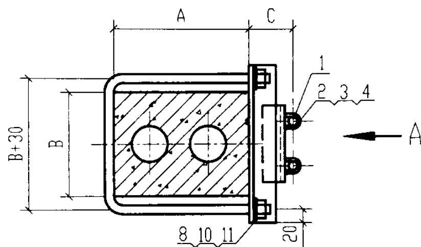
I 沿屋架下弦侧敷设
