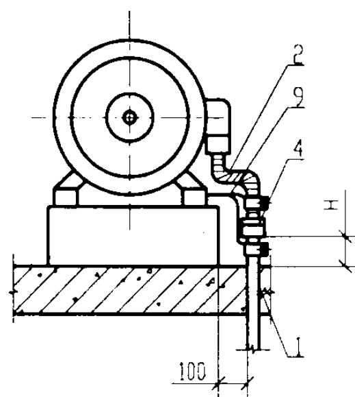
II 室内电机暗配线敷设
