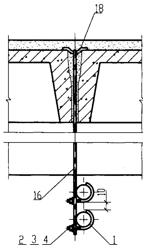
IV 沿预制板板缝下敷设(梁下)
