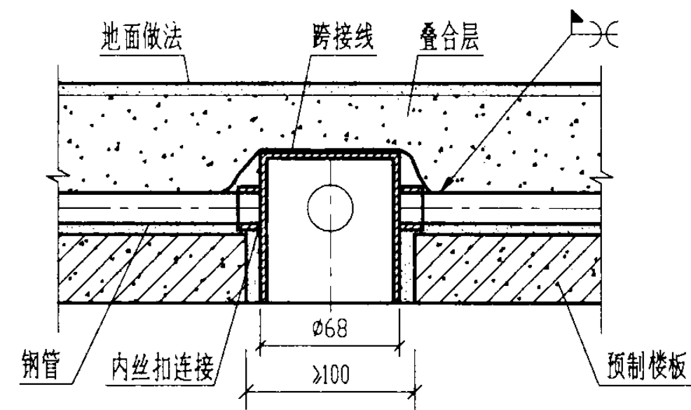
高身接线盒预制楼板上安装
