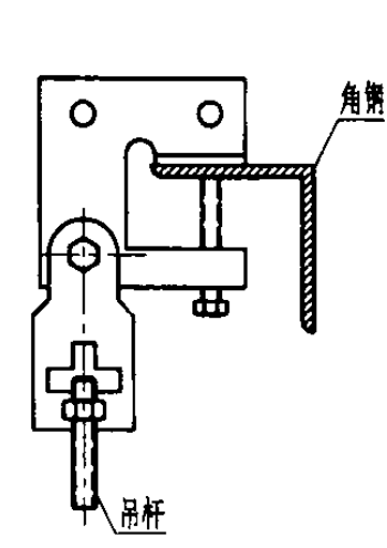
KH型万向吊架110kg 配置立面图
