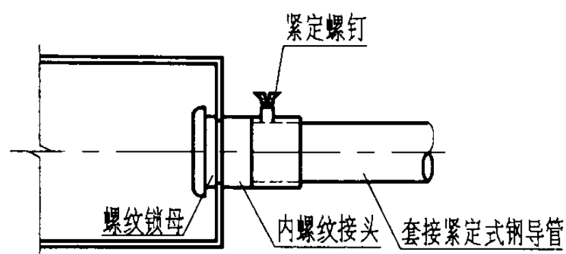
套接紧定式钢导管与接线盒连接
