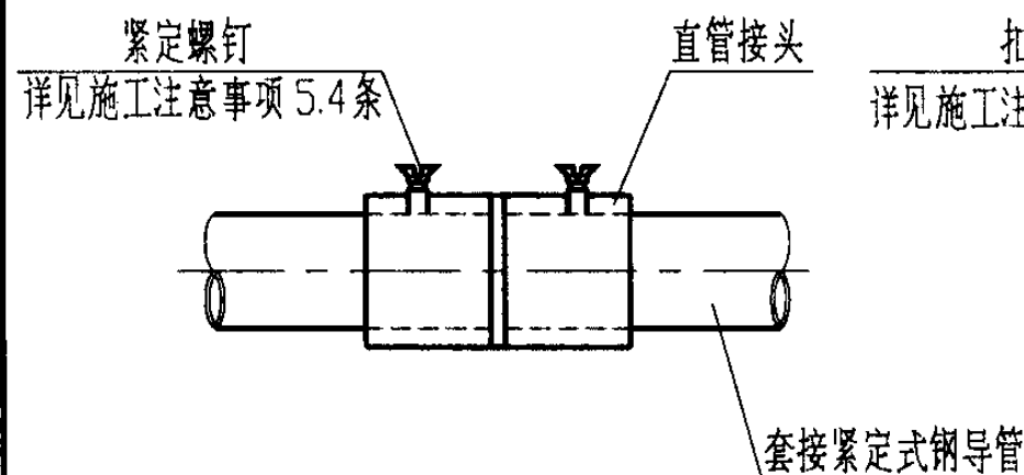
套接紧定式钢导管紧定螺钉连接
