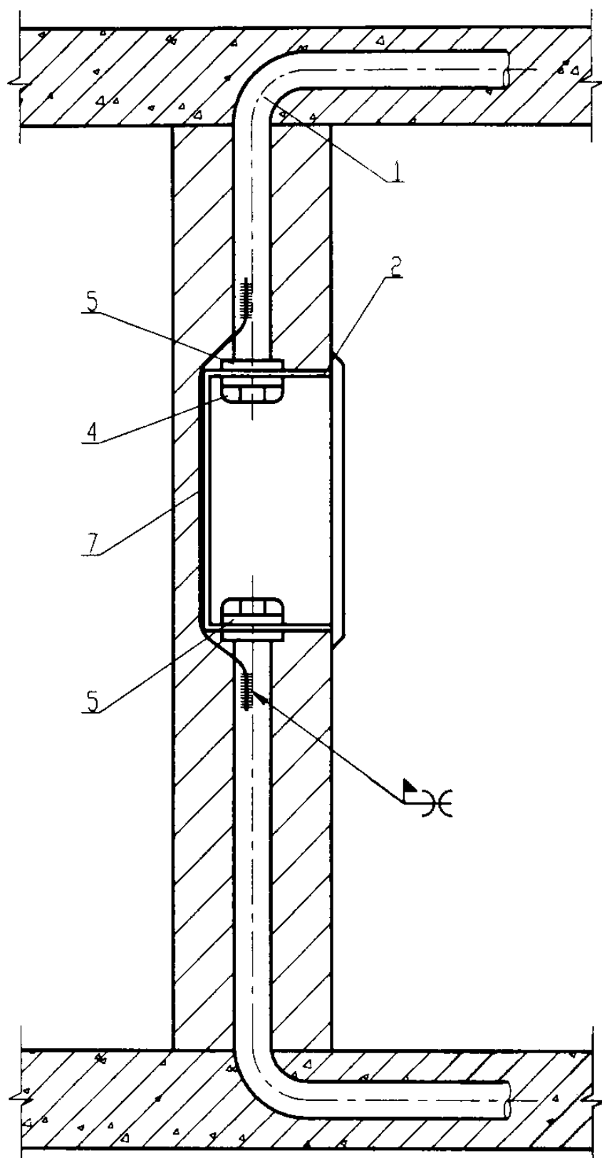
I 嵌入式配电装置暗管进出安装
