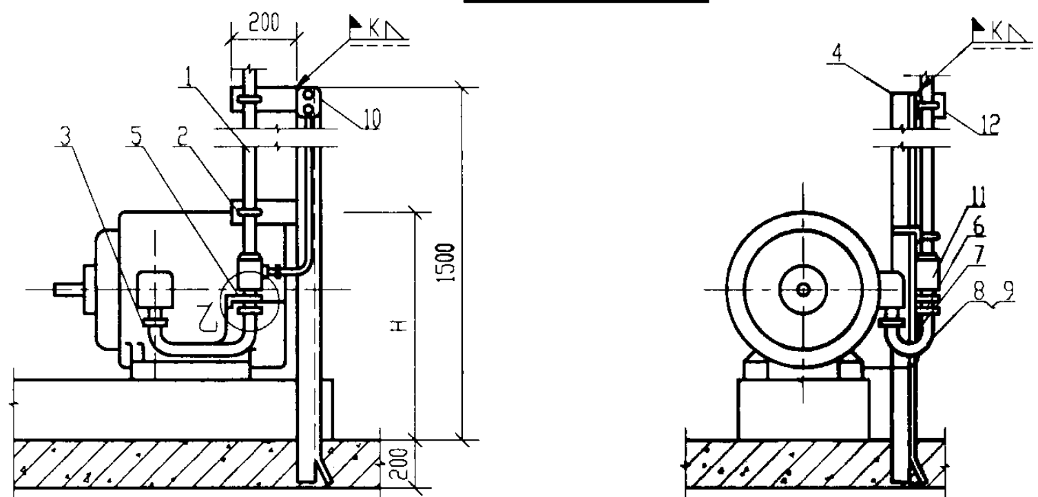
I 室内电机明配线敷设
