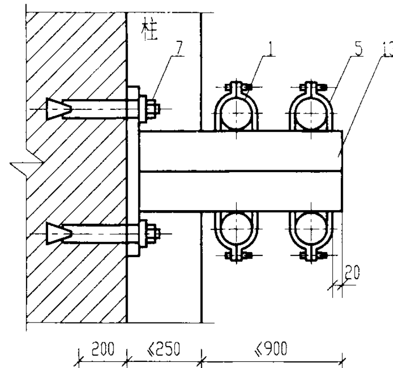
V 多管沿墙跨柱敷设
