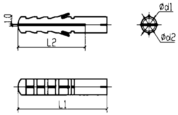
塑料胀管
