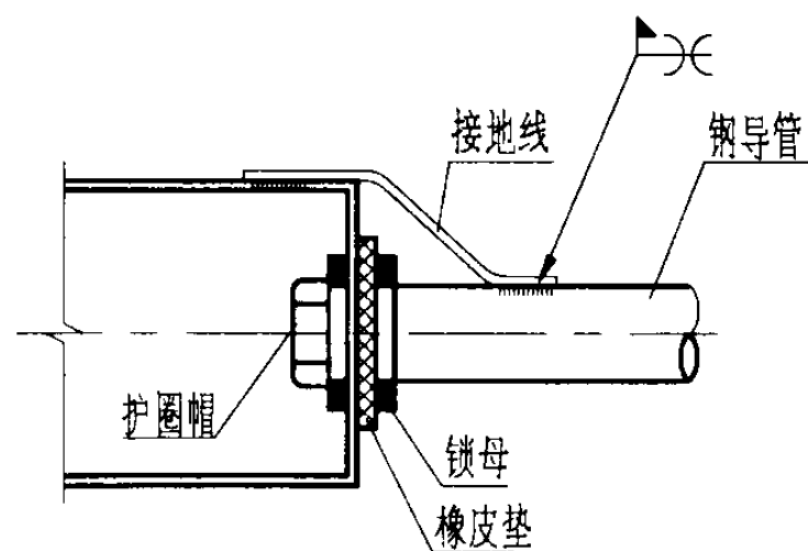
钢管与接线盒连接
