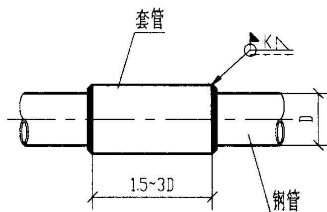
钢管套管连接
