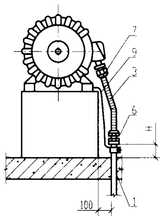
I 室外防水电机暗配线敷设
