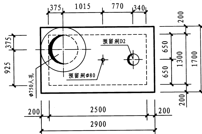
顶板平面图
