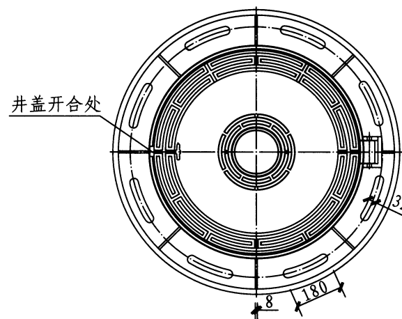
Ø 800防寒成品井盖
