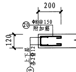
1-1 剖面图
