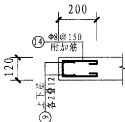
1-1 剖面图
