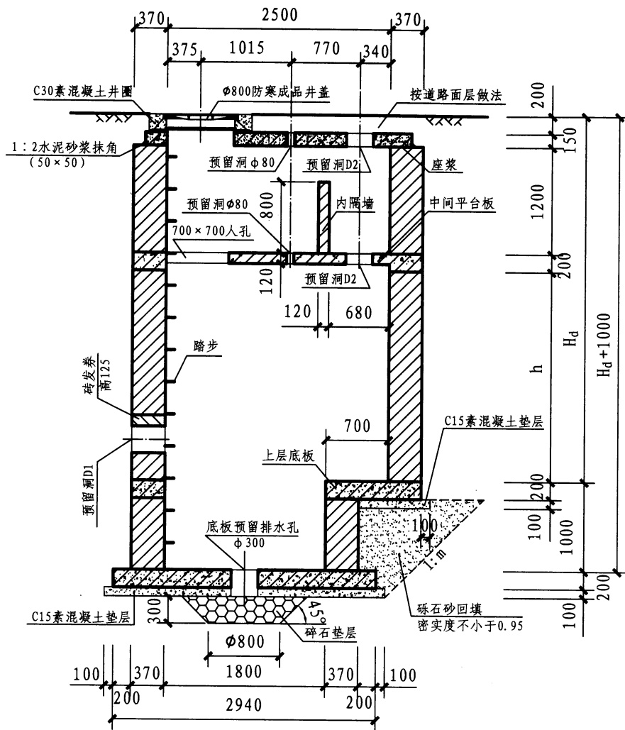
1-1 剖面图
