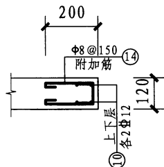
2-2 剖面图
