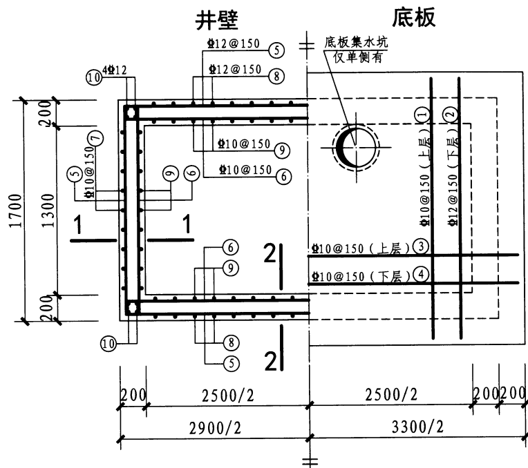
井壁、底板配筋平面图
