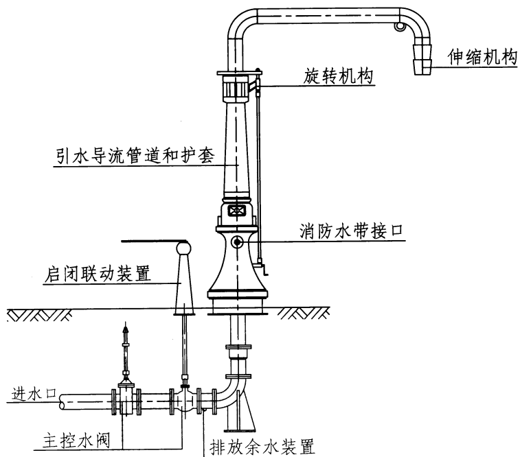
图2 消防水鹤简图
