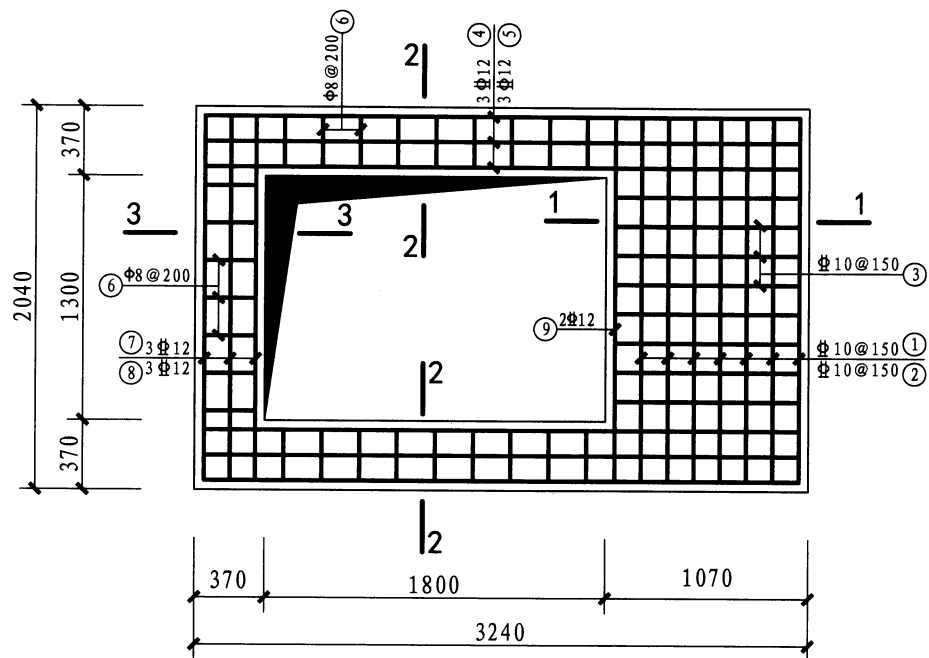
上层底板配筋平面图
