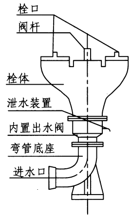
室外地下式消防栓
