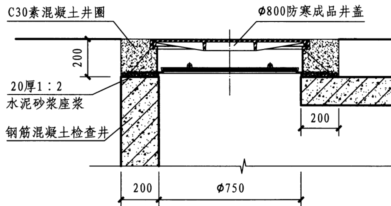
Ø 800防寒成品井盖安装图 (二)
