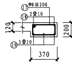
L2配筋图
