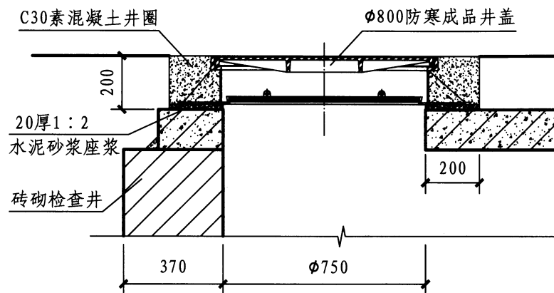
Ø 800防寒成品井盖安装图 (一)
