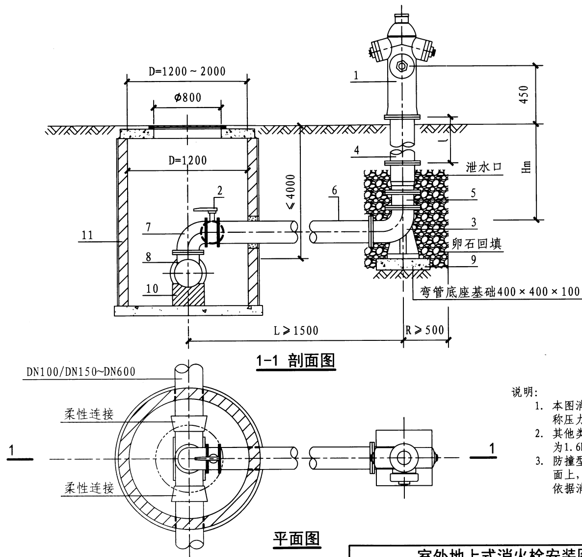
室外地上式消防栓安装图 (有检修阀 干管安装)
