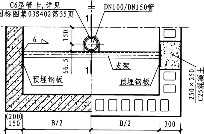
矩形闸阀井支架平面图
