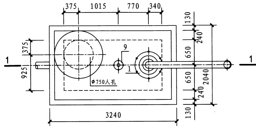
上层平面图
