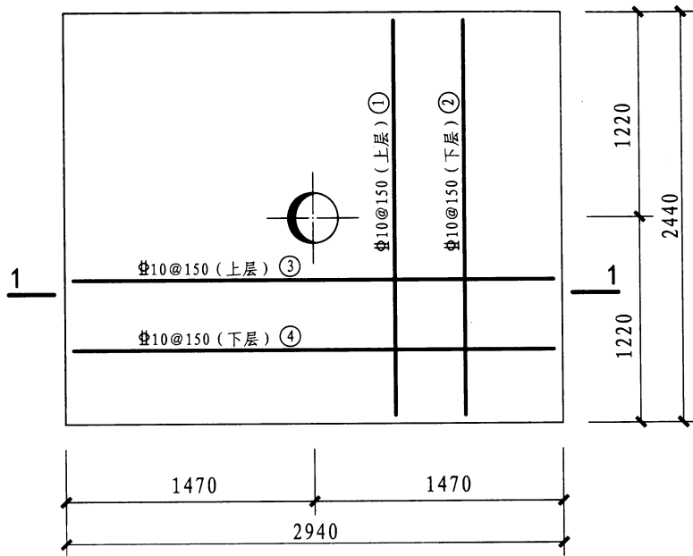
下层底板配筋平面图
