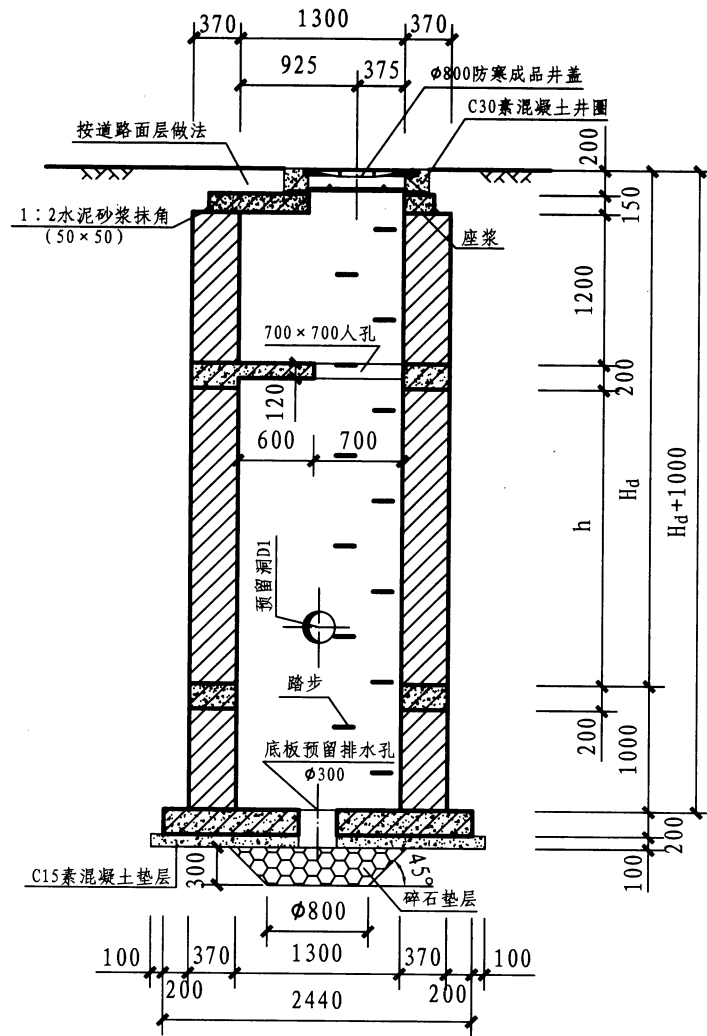
2-2 剖面图
