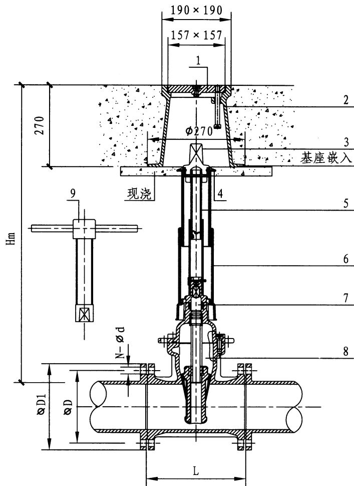
闸阀直埋安装图
