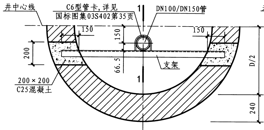
圆形闸阀井支架平面图
