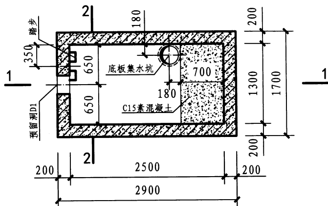
下部平面图
