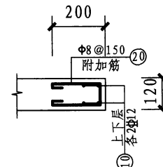
2-2 剖面图
