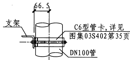
1-1 剖面图
