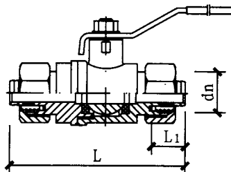
卡套式球阀
