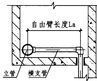
支管连接(四)平面
