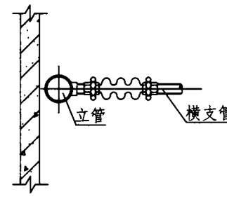
支管连接(五)平面
