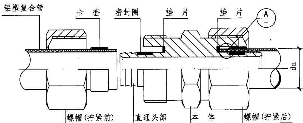
卡套式连接
