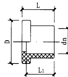
法兰连接件
