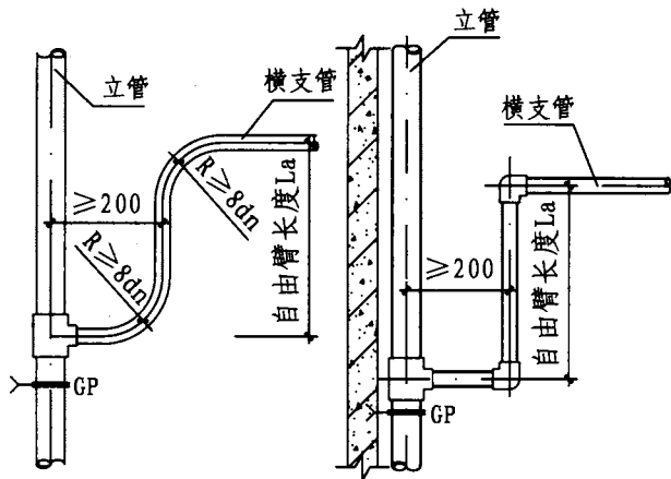
支管连接(一)立面 ( dn \leq 32 )
