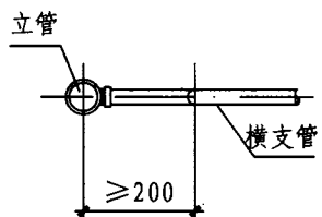
支管连接(一)平面 ( dn \leq 32 )
