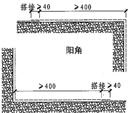
阴角 图B86
