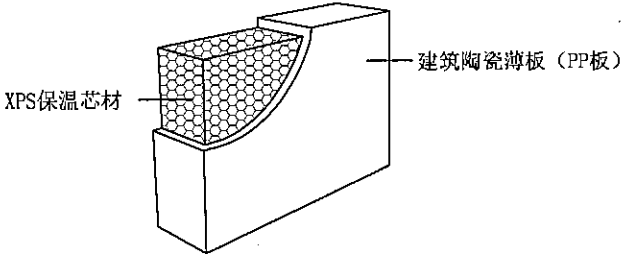
图1 保温装饰板构造（一）
