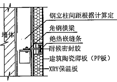
图9 干挂系统竖向节点大样
