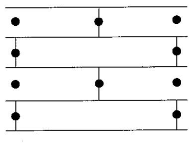
图H6 岩棉带锚栓分布图
