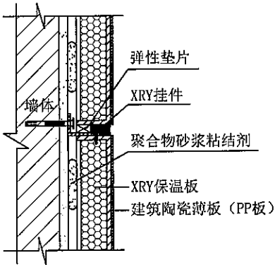
图7 挂贴系统竖向节点大样
