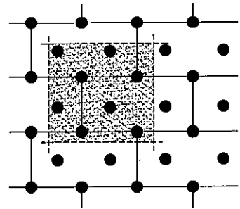
图H5 岩棉板锚栓分布图
