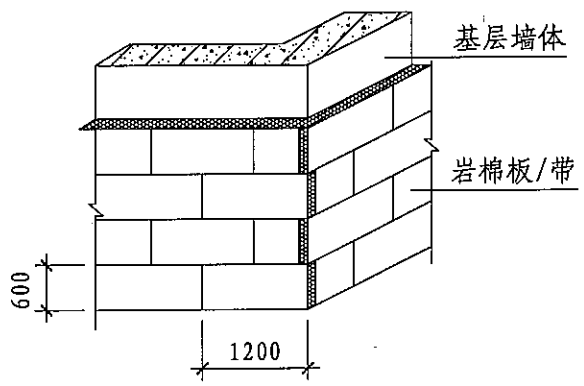
图H3 墙角处保温板排列
