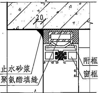
图B29 抹止水砂浆
