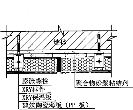
图6 挂贴系统横向节点大样
