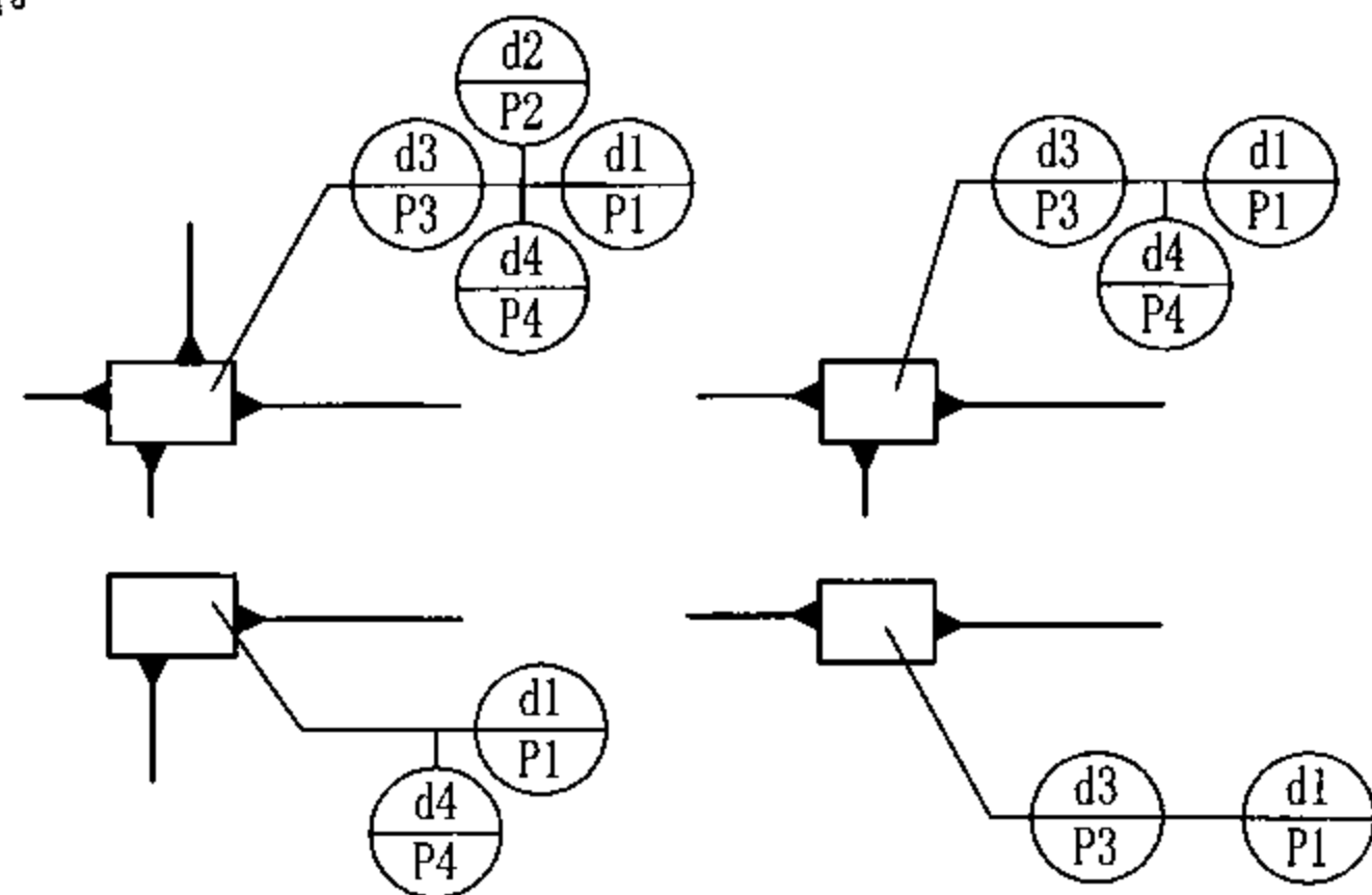
图3 梁柱节点详图的索引方式举例
