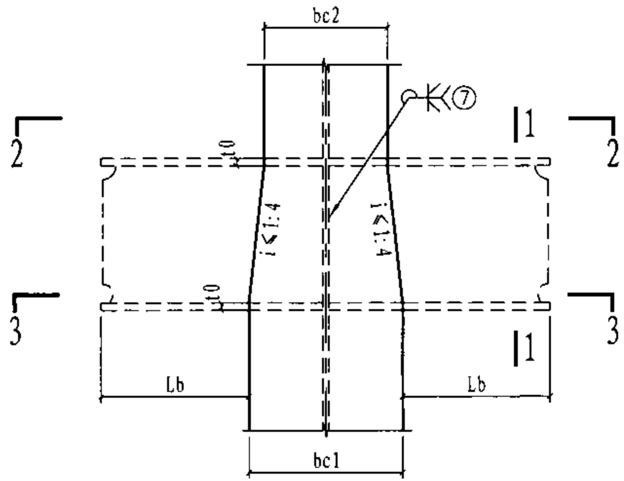
41 未标注焊缝为7号焊缝
