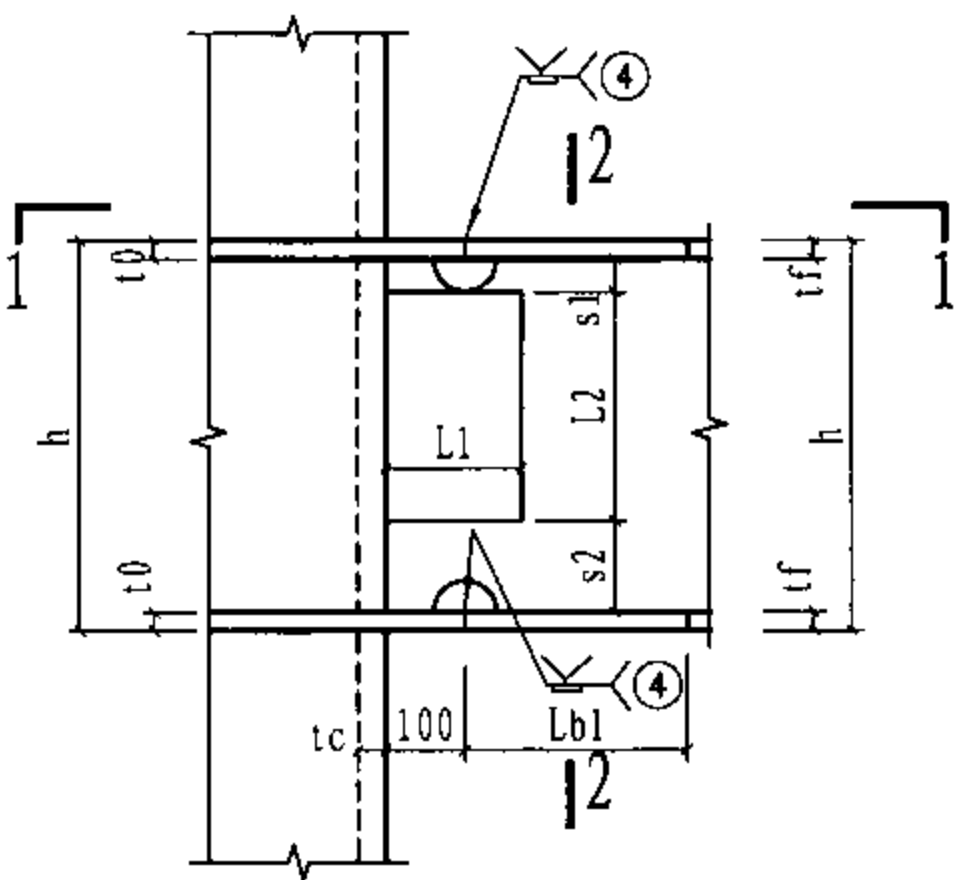
13 节点区未标注焊缝为7号焊缝
