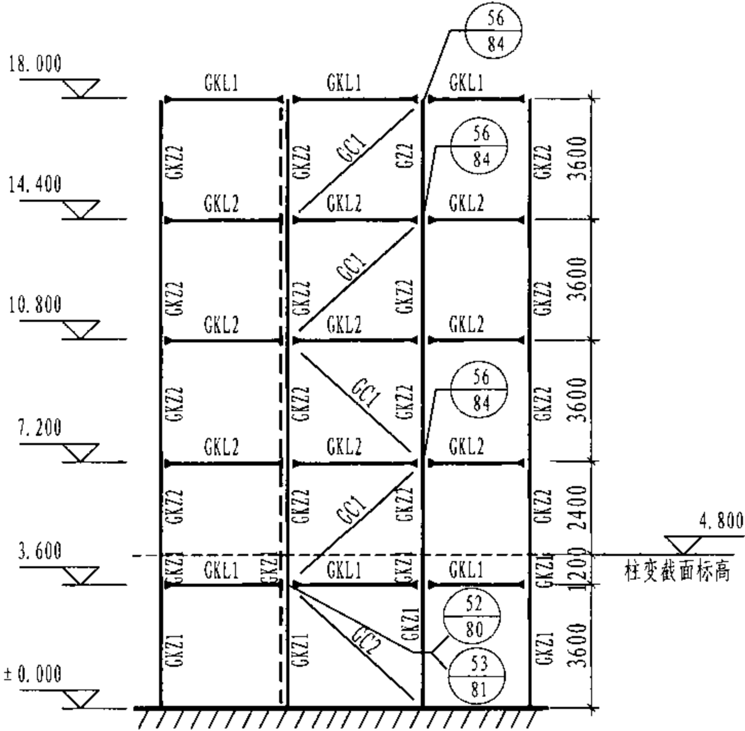
图8 某工程GKC1立面的布置图
