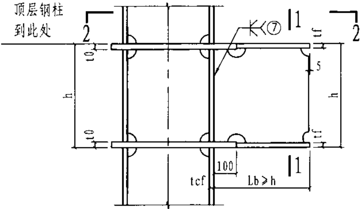
24 未标注焊缝为7号焊缝
