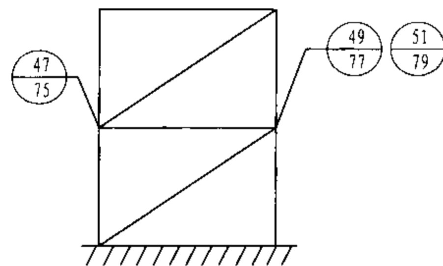
图14 箱形柱强轴在框架平面内且支撑转轴时节点参数法详图索引
