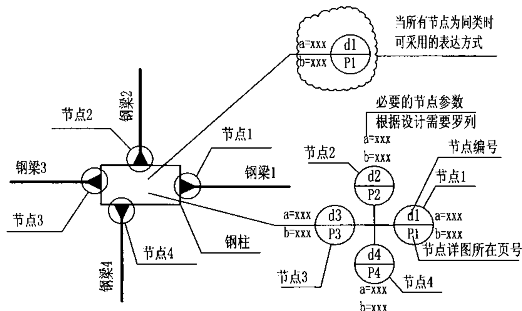
图2 梁柱节点详图索引示意图及说明
