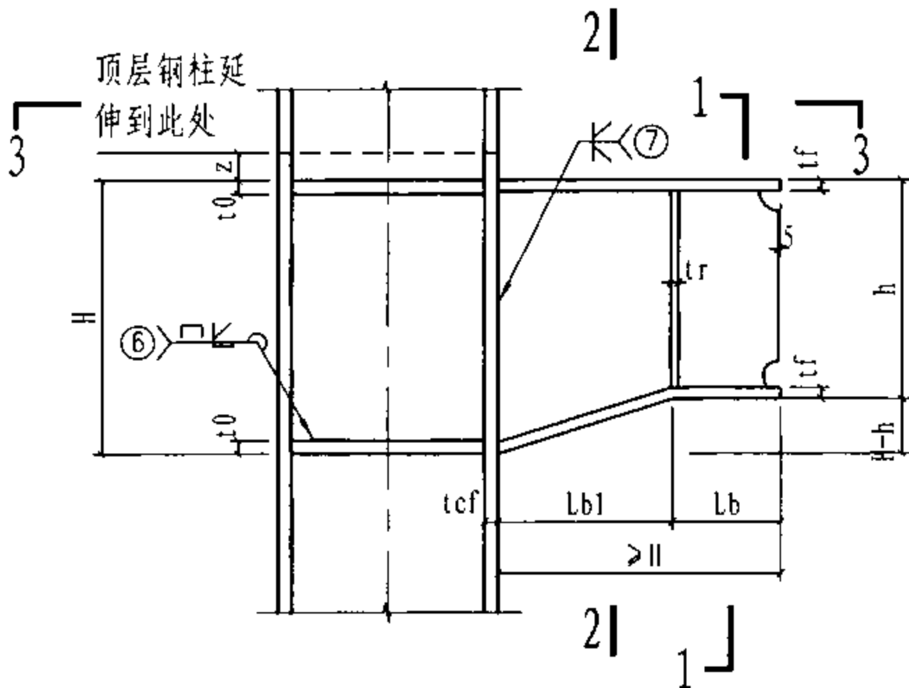
18 未标注焊缝为7号焊缝
