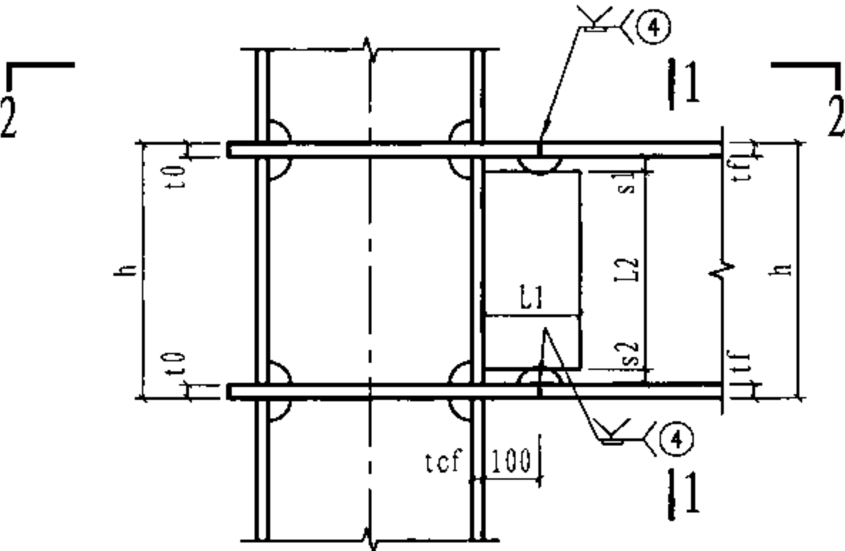
28 节点区未标注焊缝为7号焊缝
