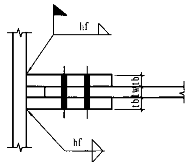
C 用于梁腹板剪力较小时的双剪连接
