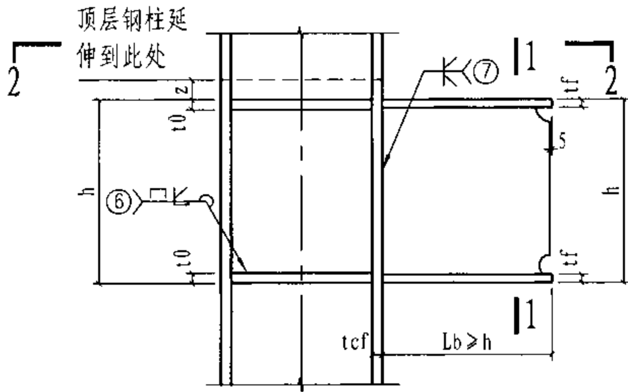
16 未标注焊缝为7号焊缝
