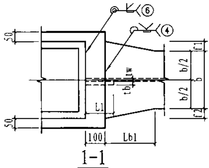
13 节点区未标注焊缝为7号焊缝
