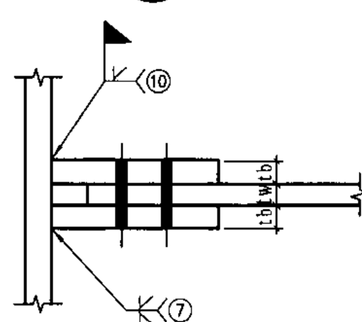
D 用于梁腹板剪力较大时的双剪连接
