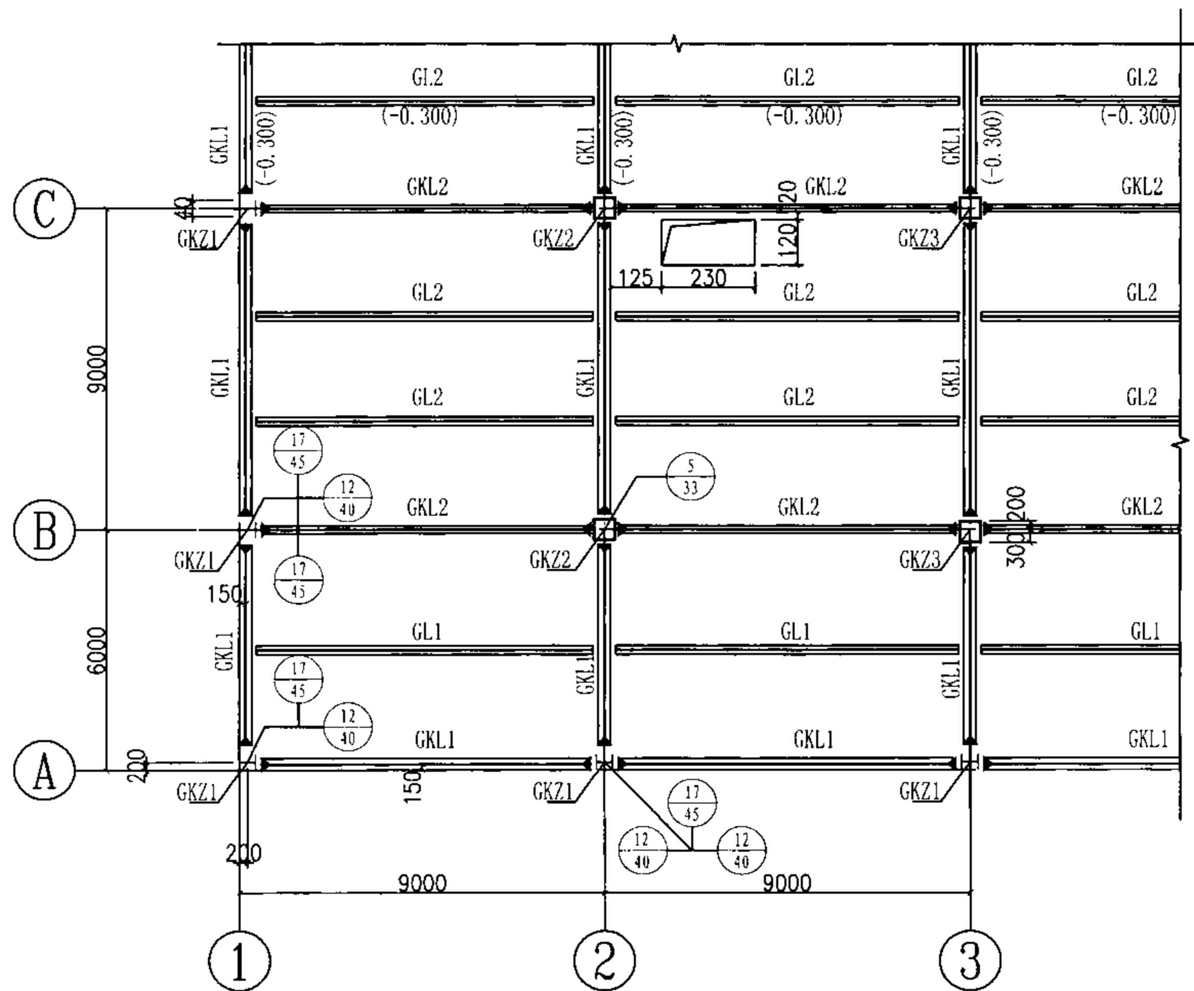
图 3 二层结构平面布置图 (梁顶标高6.000 m)
