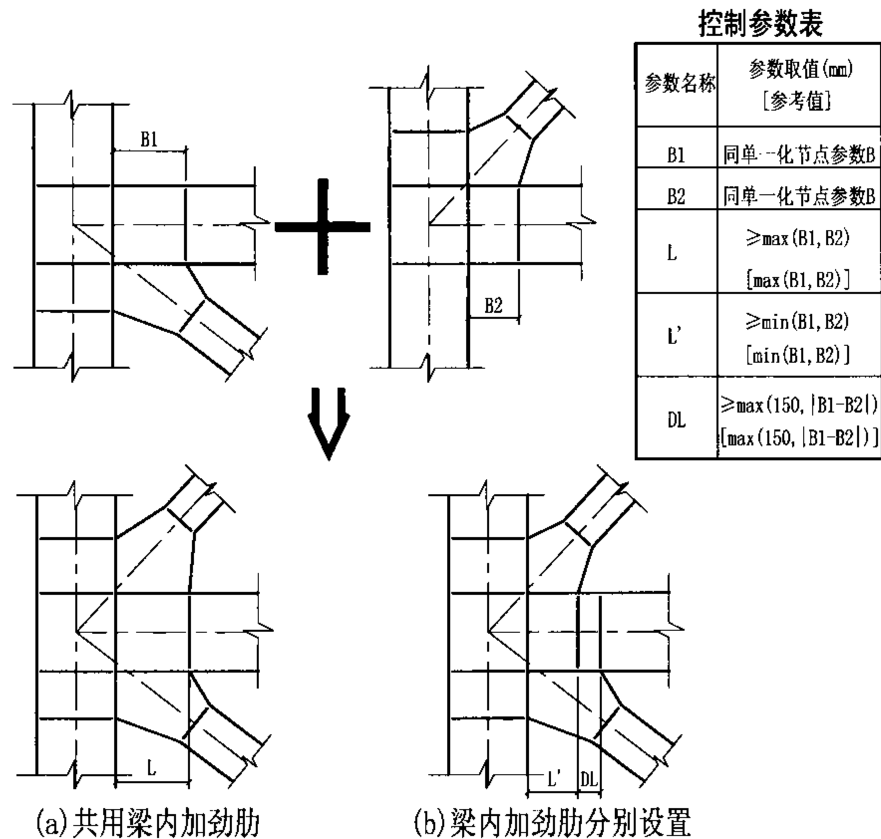
图12 支撑与梁汇交的组合
