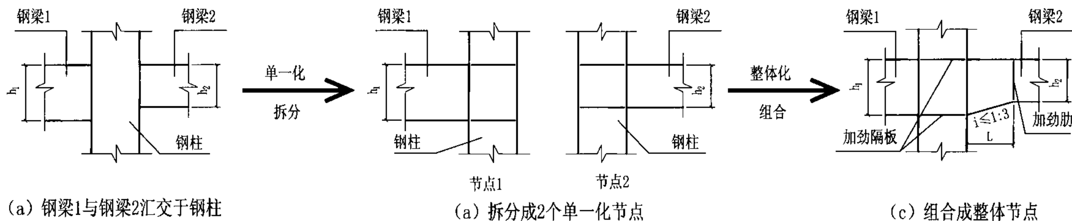
图1 参数化节点设计原理示意图
