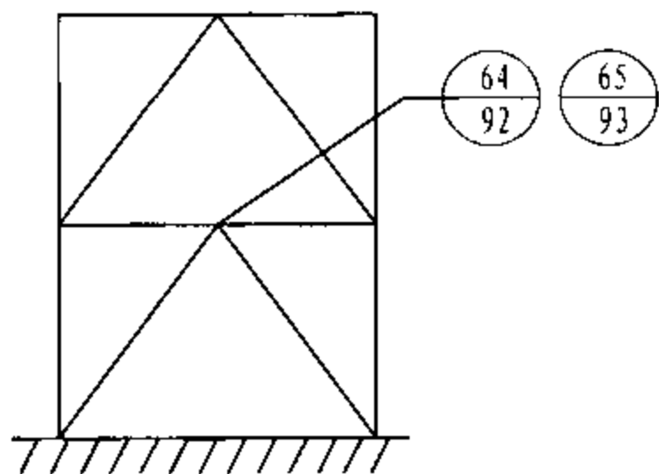
图15 与H形梁连接的人字形、V字形支撑节点节点参数法详图索引
