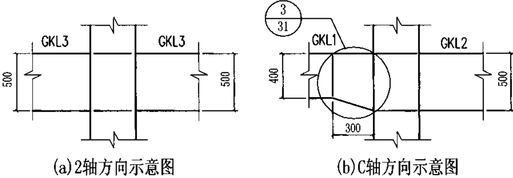
图19 梁柱节点组合结果简图
