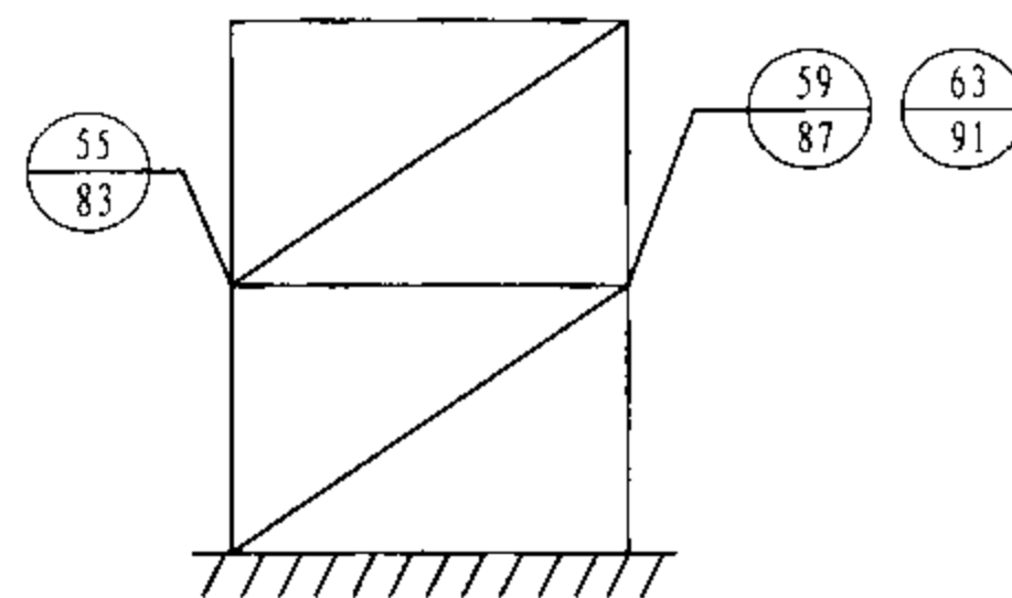
图12 H形柱强轴在框架平面外且支撑转轴时节点参数法详图索引
