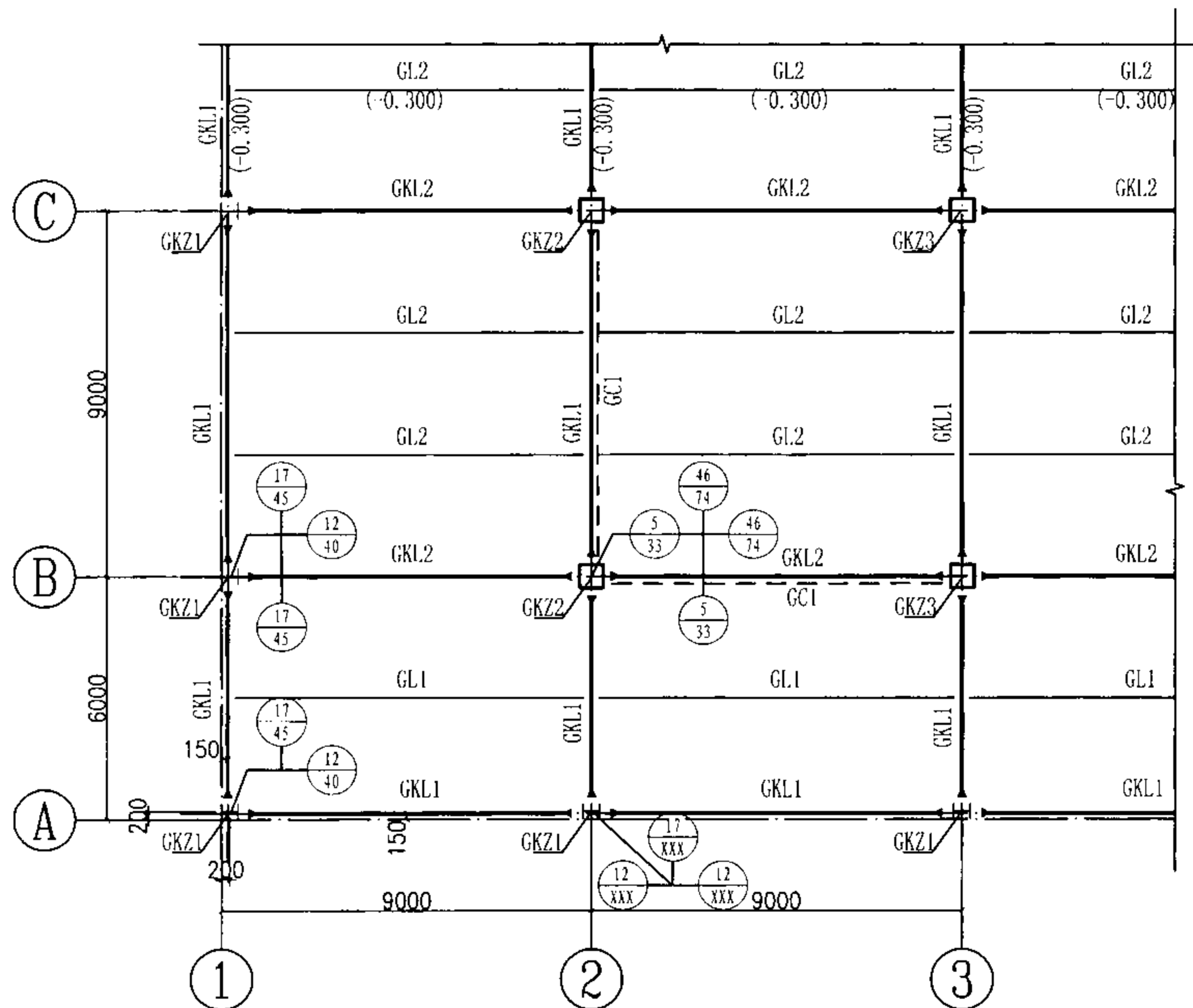
图 4 二层结构平面布置图 (梁顶标高 6.000 m)
