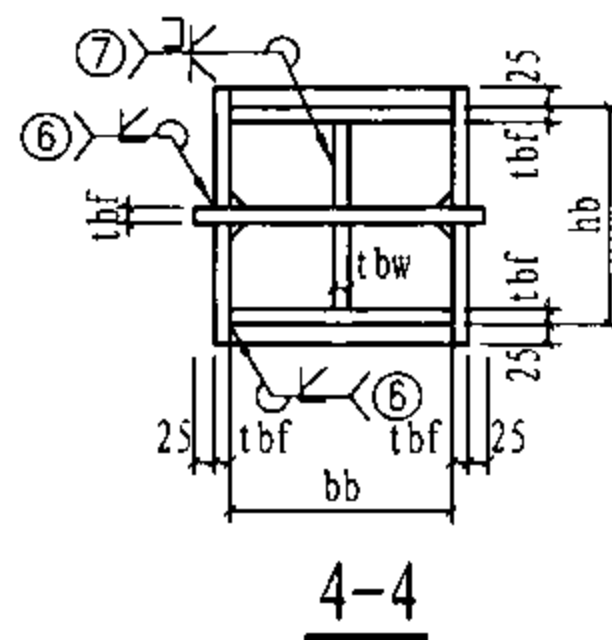
H形柱-支撑节点
