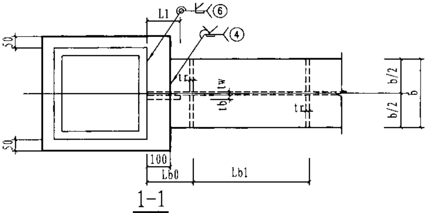
14 节点区未标注焊缝为7号焊缝
