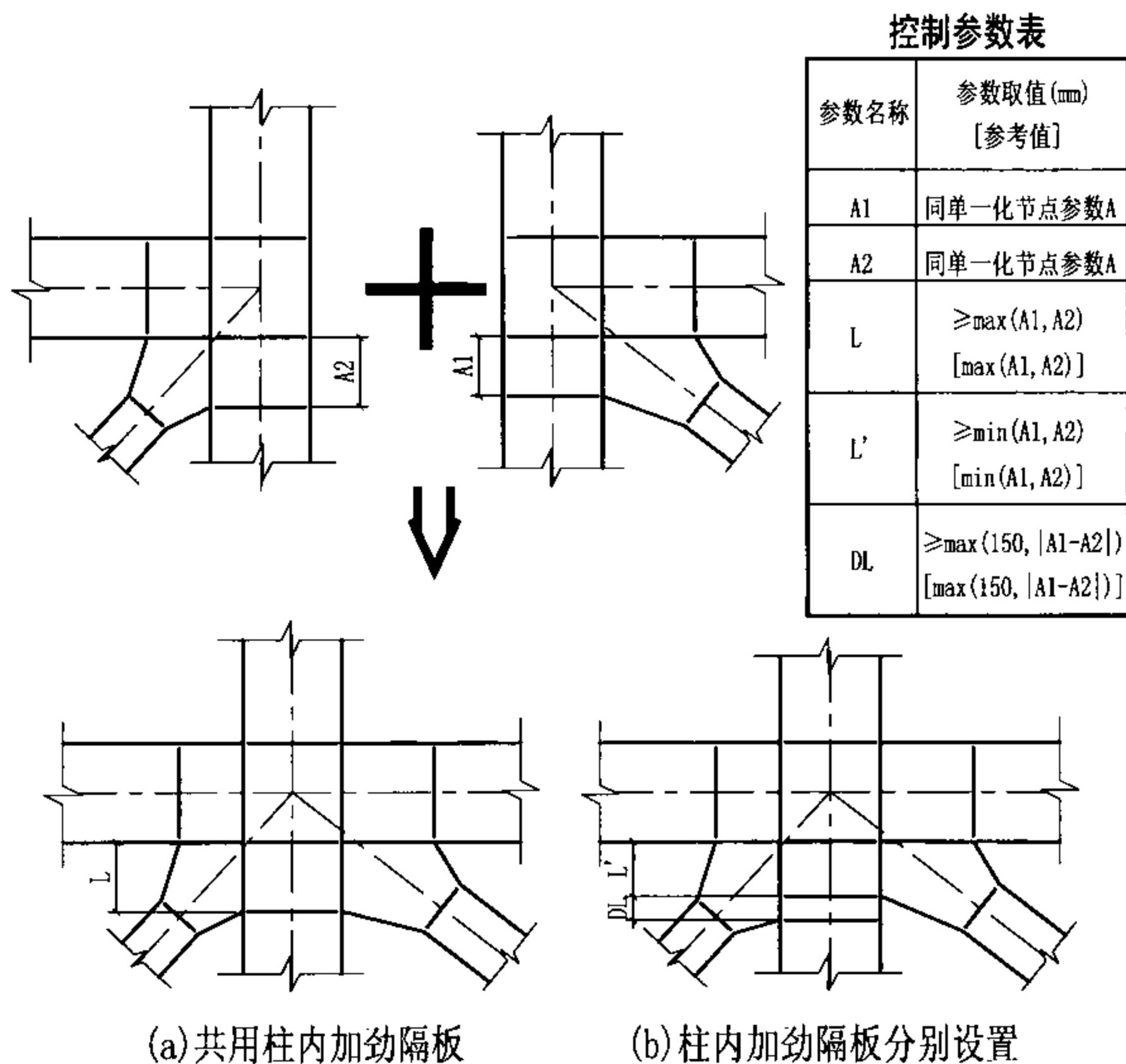
图11 支撑与柱汇交的组合
