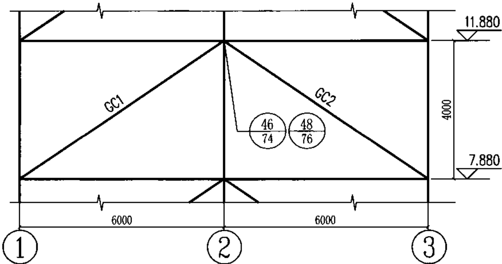
图18 局部立面布置图（GKC1） (GC1、GC2与框架梁轴线投影重合)
