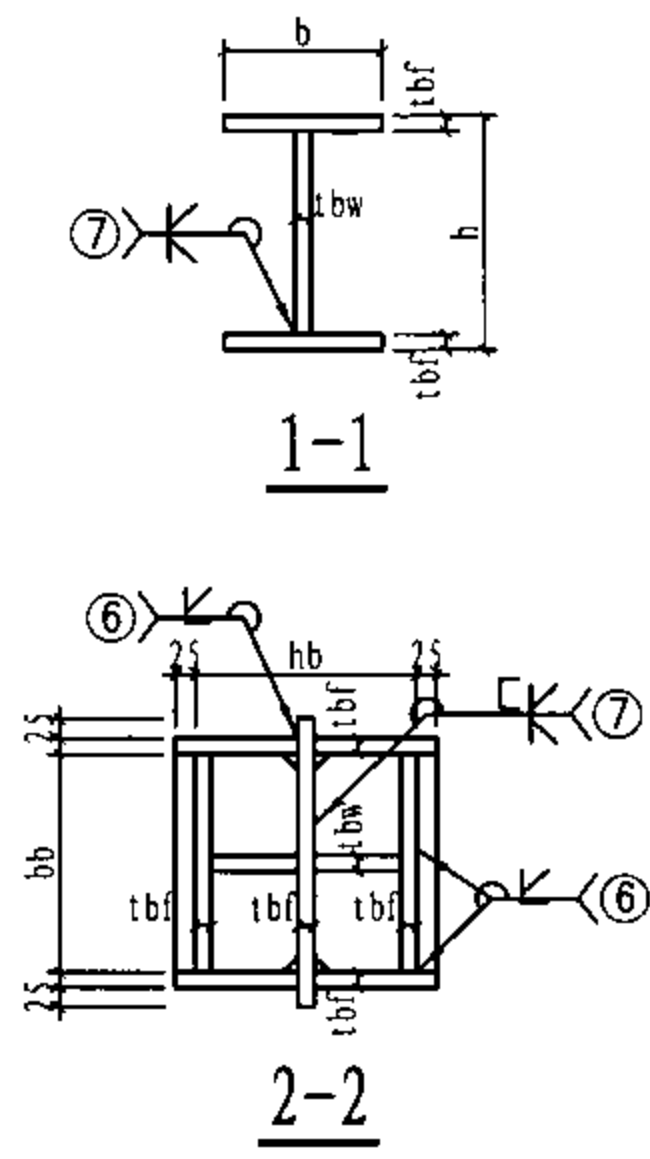
箱形柱-支撑节点
