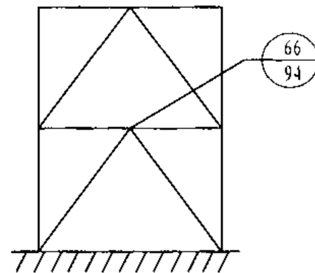
图16 与H形梁连接的人字形、V字形支撑（转轴）节点参数法详图索引
