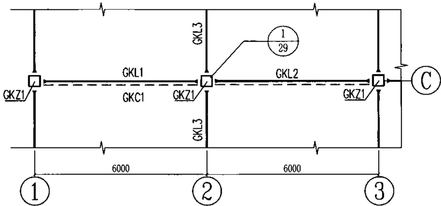
图17 3层局部平面布置图 (梁顶标高7.880m)
