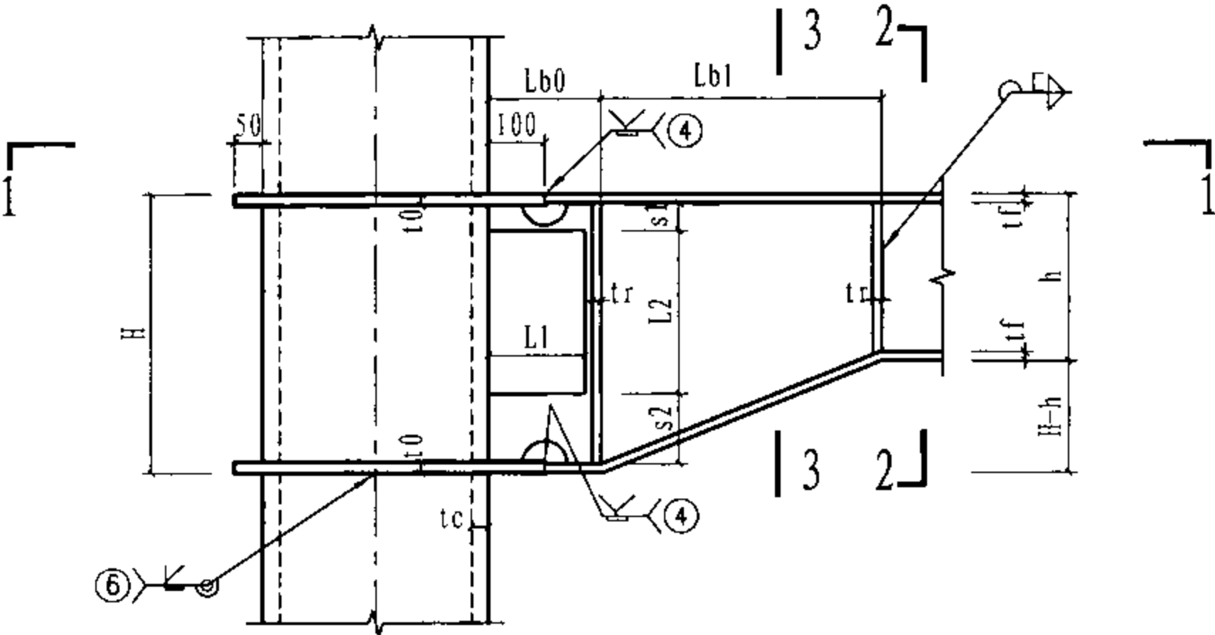
14 节点区未标注焊缝为7号焊缝
