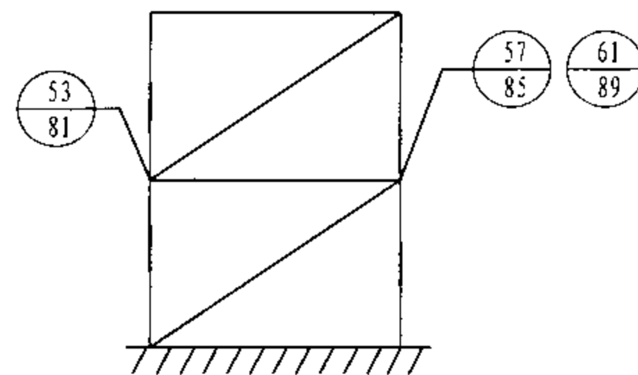
图10 H形柱强轴在框架平面内且支撑转轴时节点参数法详图索引
