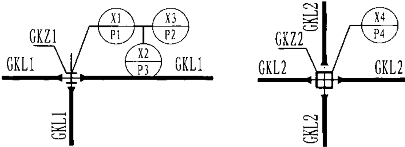
图 2 节点注写示意图
