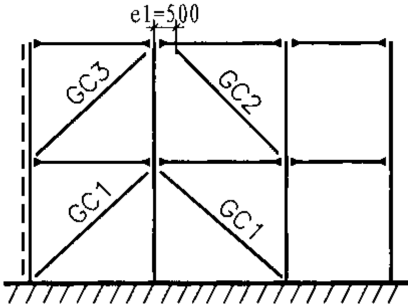
图6 立面布置图中钢支撑的注写规则
