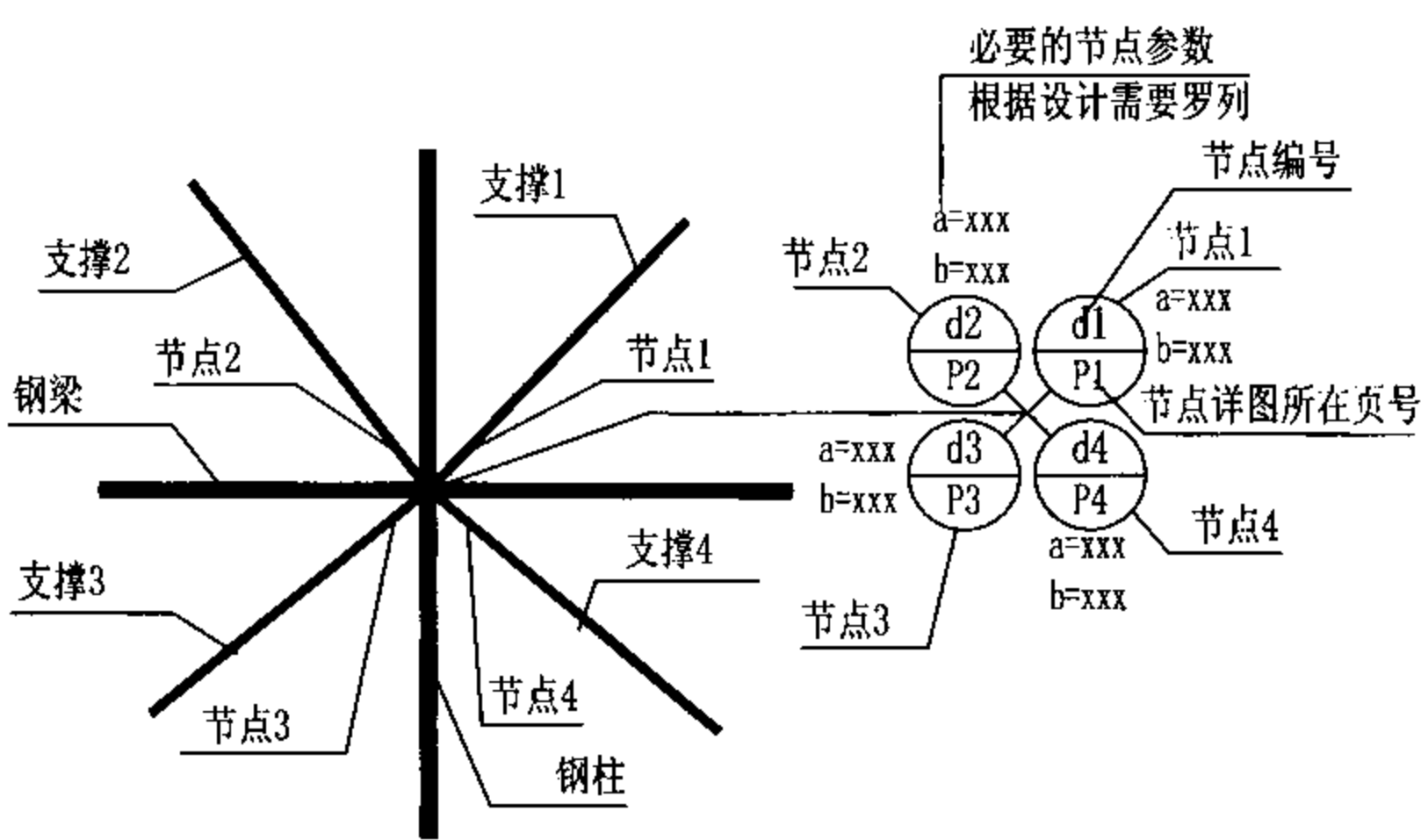
图8 支撑节点详图索引示意图及说明
