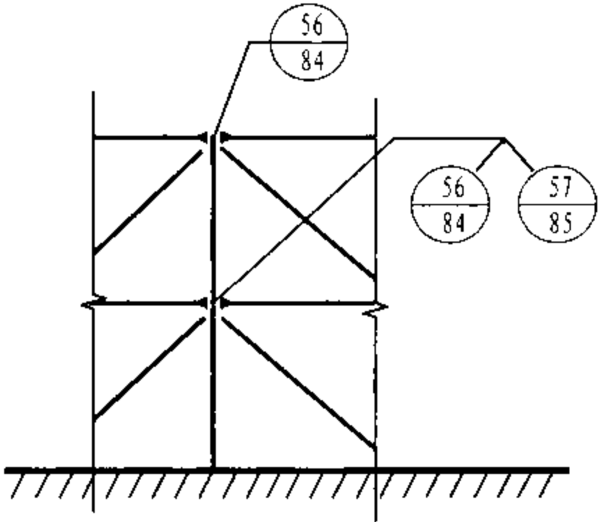
图7 立面布置图中节点的注写规则
