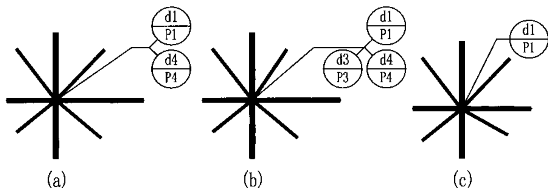
图10 梁柱节点索引的简化标注
