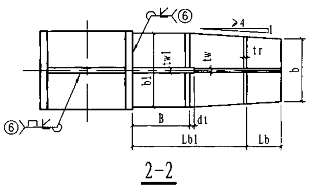
H形柱-支撑节点
