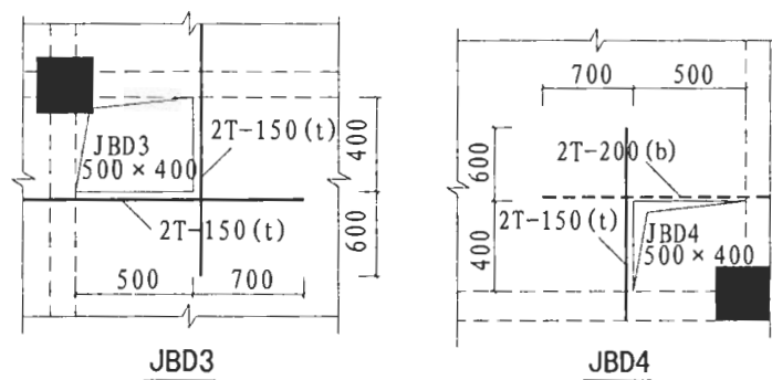
图 4.2.5 碳纤维加固楼板洞口平面注写方法示例
