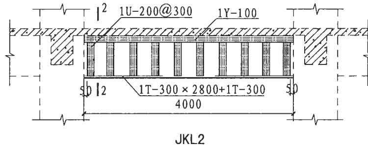
图 3.2.2 (b) 碳纤维加固梁底示意图
