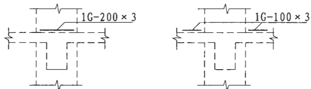
图 3.2.3 (d) 粘钢加固梁支座截面示意图
