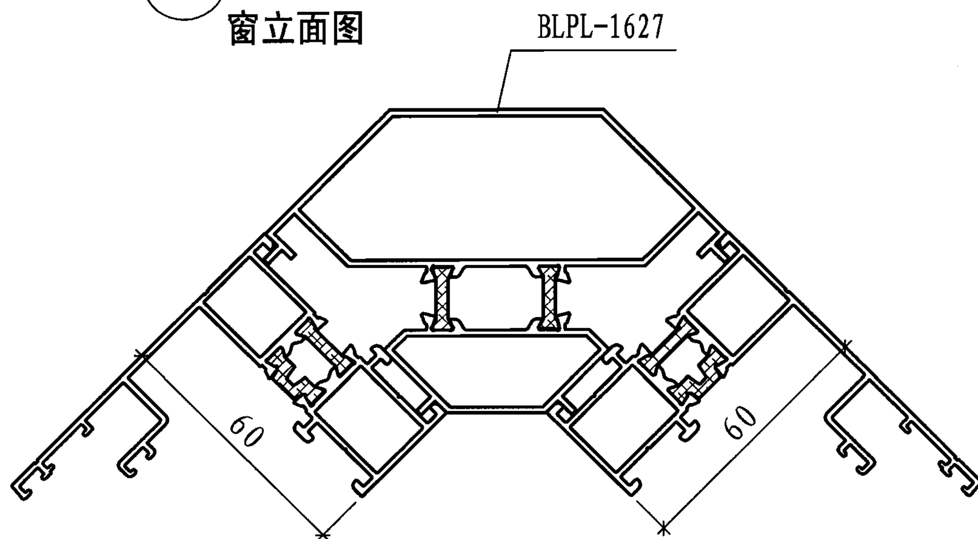
窗转角
