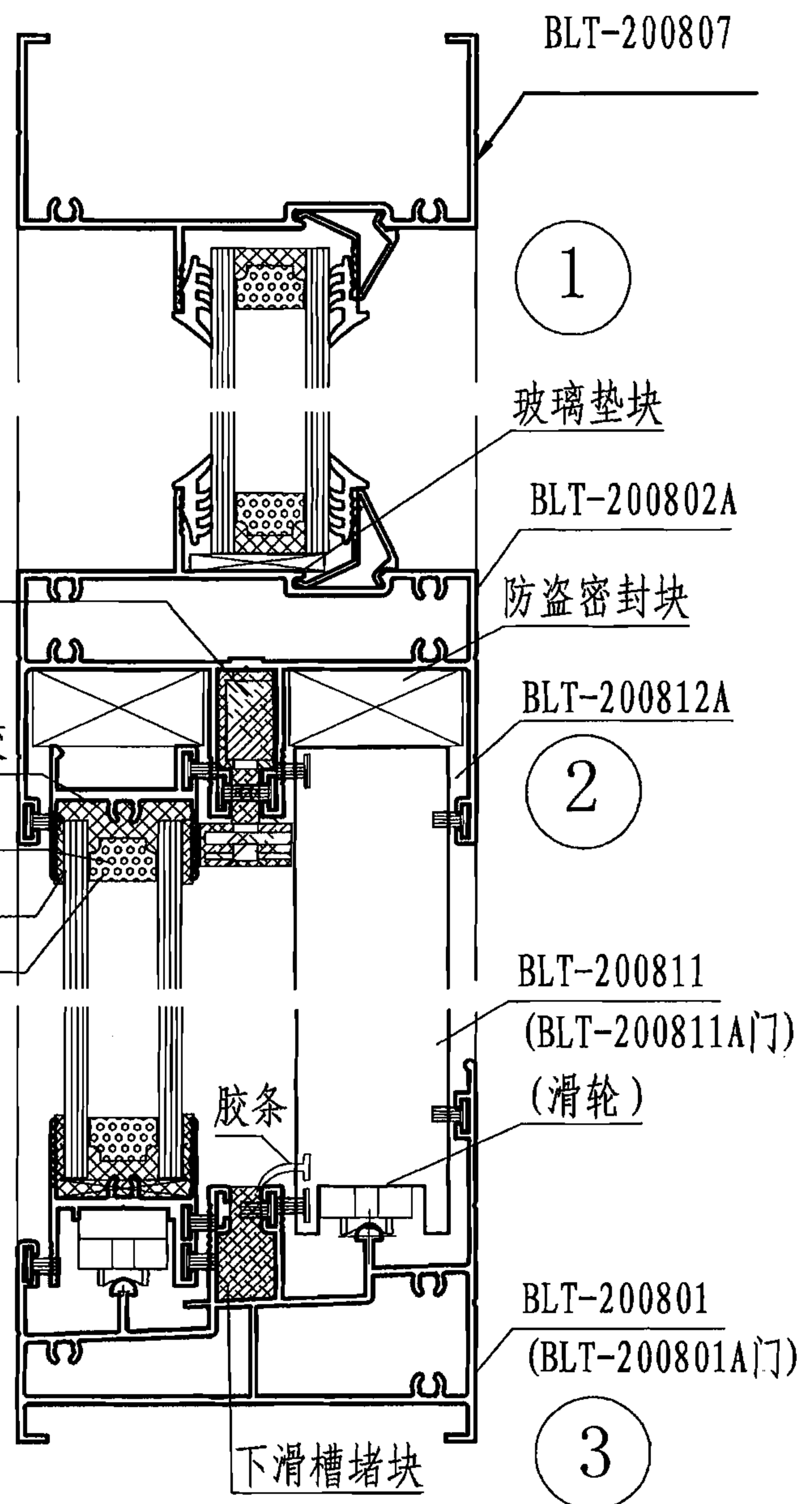
BLT2008系列无框推拉窗(门)节点图
