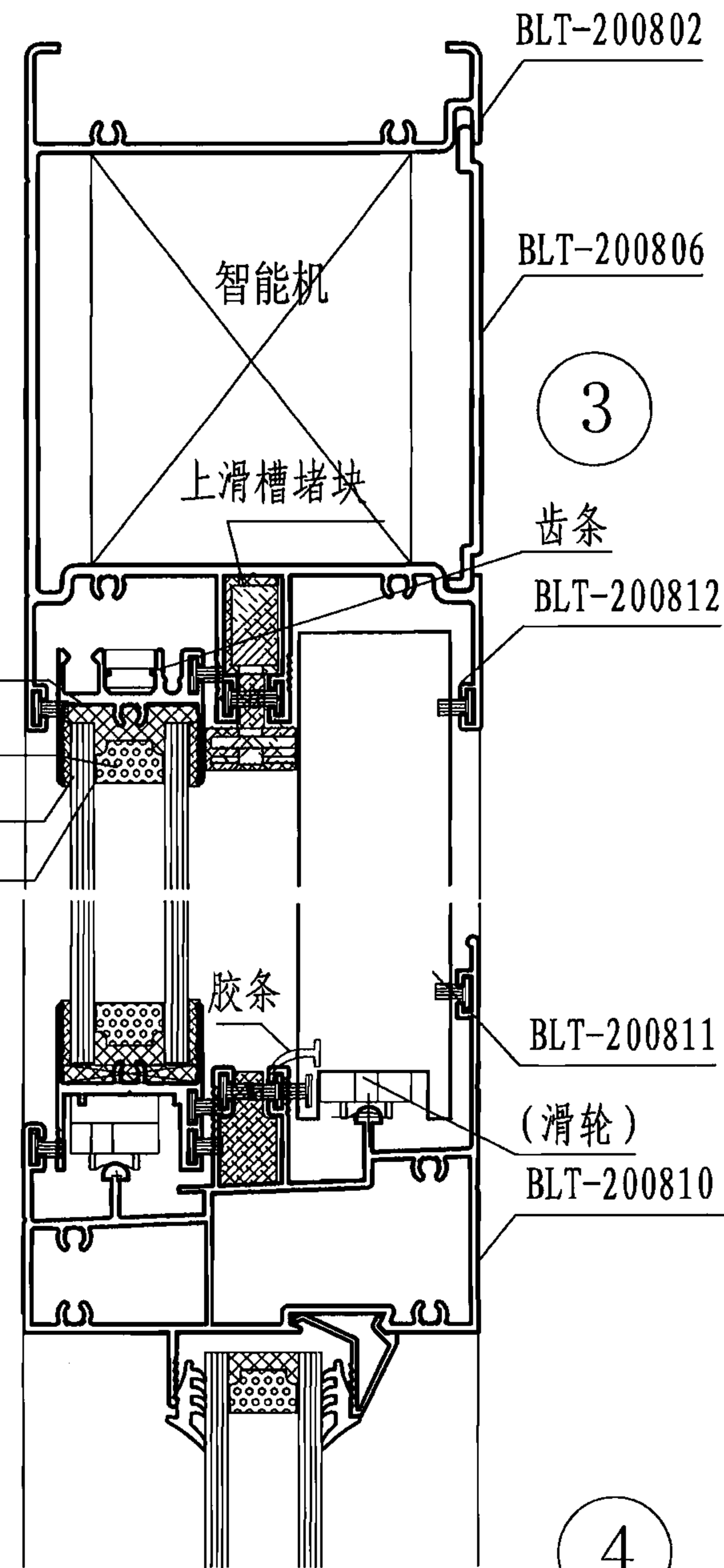
BLT2008系列无框推拉窗(门)节点图
