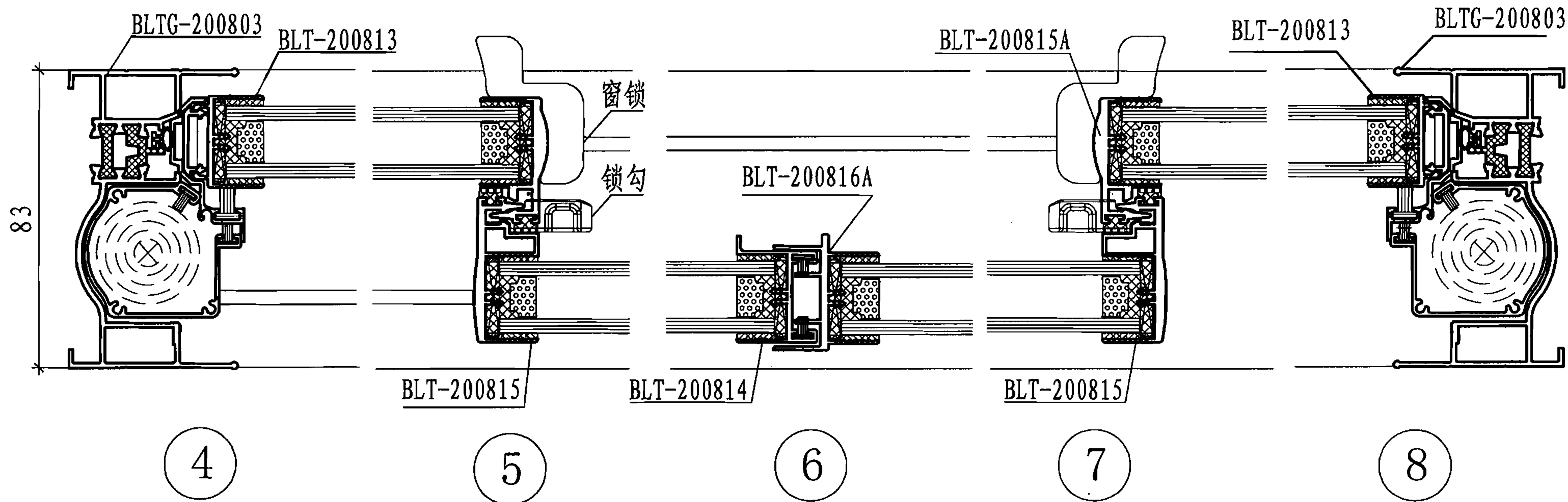
BLT2008系列断桥无框推拉窗（门）节点图
