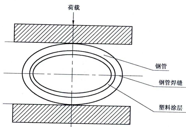
图 1 压扁试验
