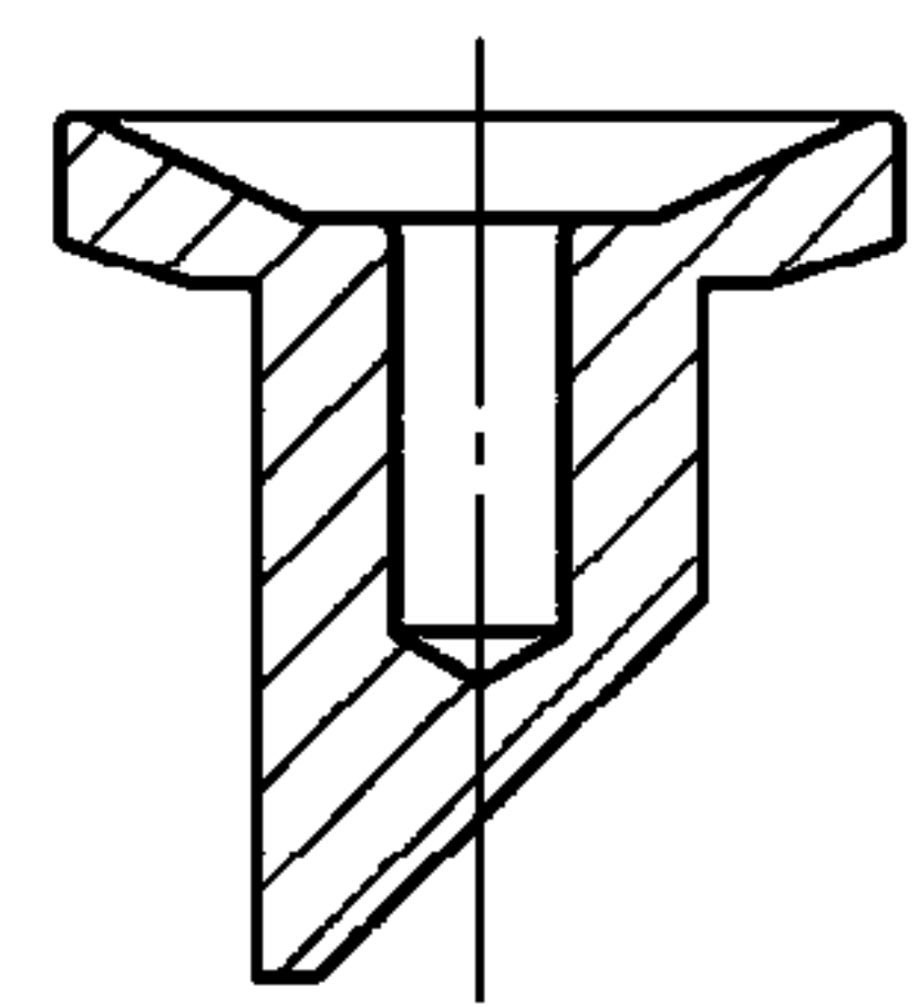
图 3 卡具组件——球座图
