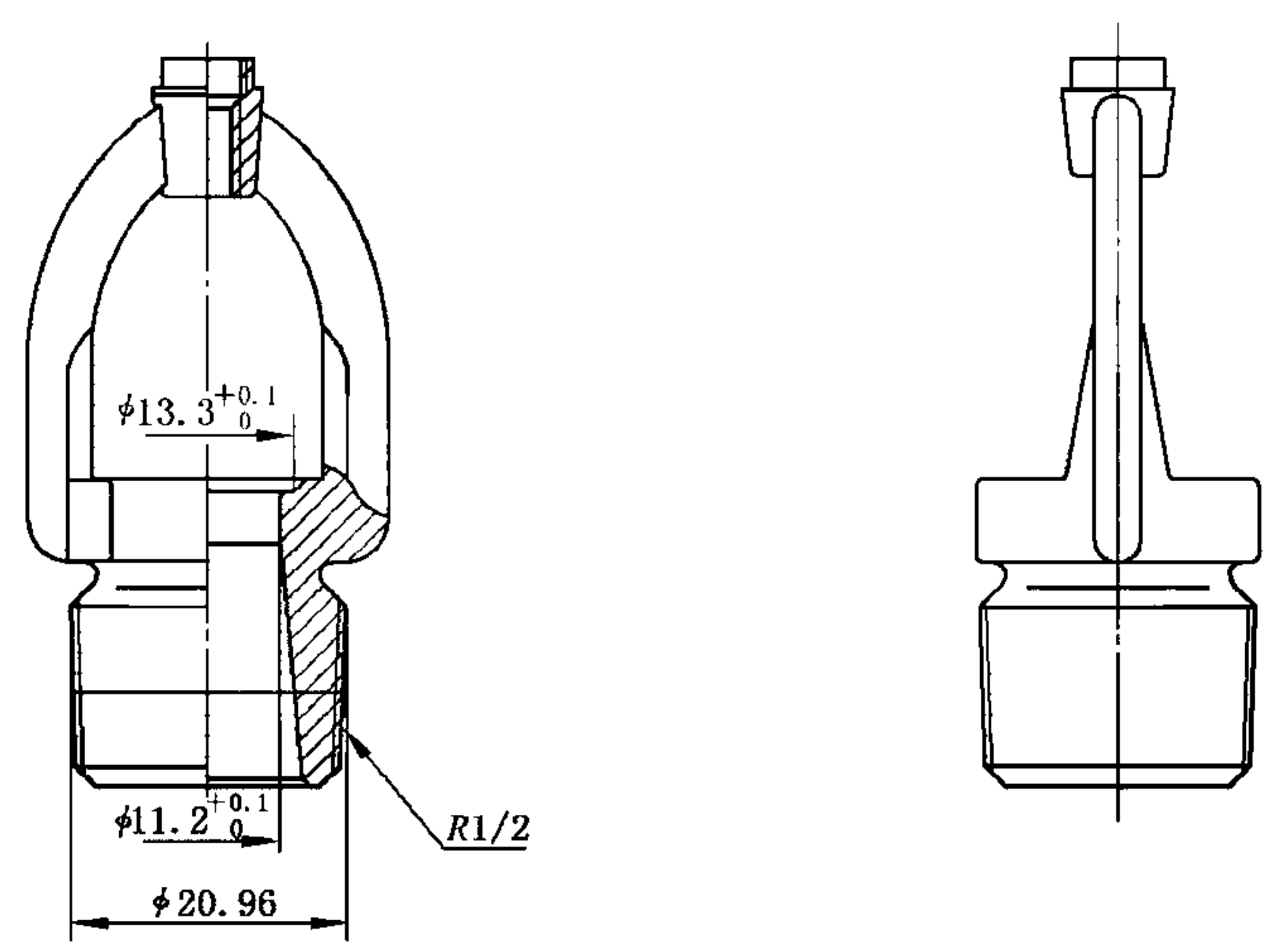
图 2 卡具组件图
