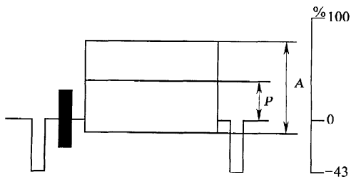
图 3.2.7 全红(绿、蓝)场信号
