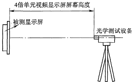
图 3.4.3 测量位置
