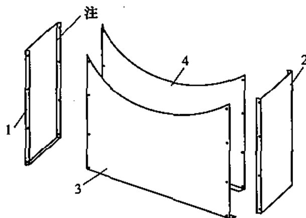
图 9.3.1 筒体支腿外保护层示意图
