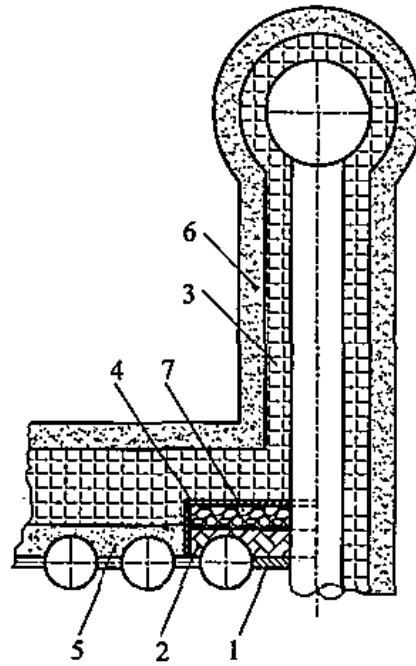
(c) 侧水冷壁与顶棚管连接处炉墙保温示意图
