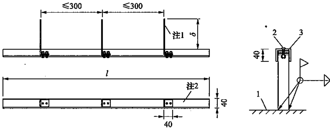
图 8.2.3 槽型带骨架示意图 (单位: mm)
