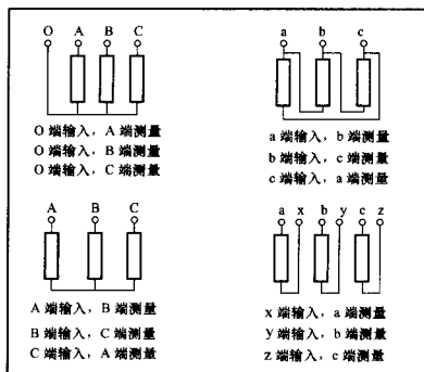
图2 变压器的几种常用检测接线方式
