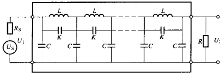
图 1 频率响应分析法的基本检测回路
