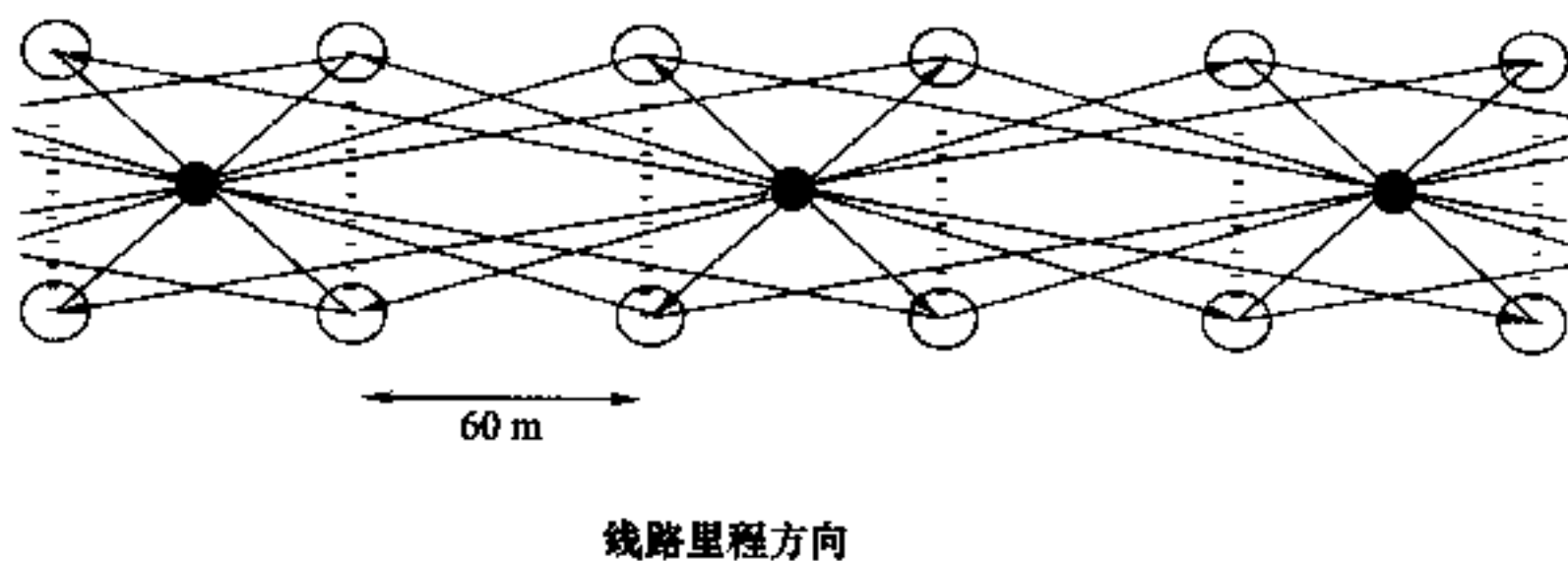
自由测站、CPⅢ点编号示意图
