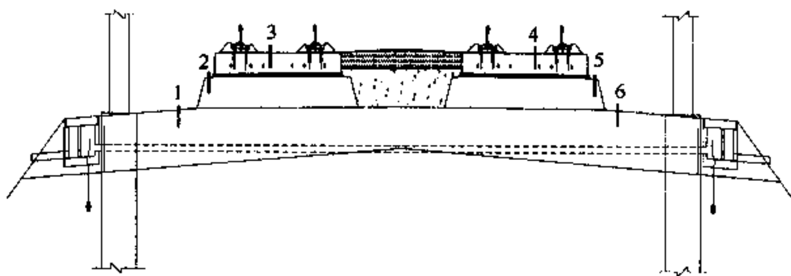
图 11.2.2—2 路基地段监测断面测点布置位置示意图
