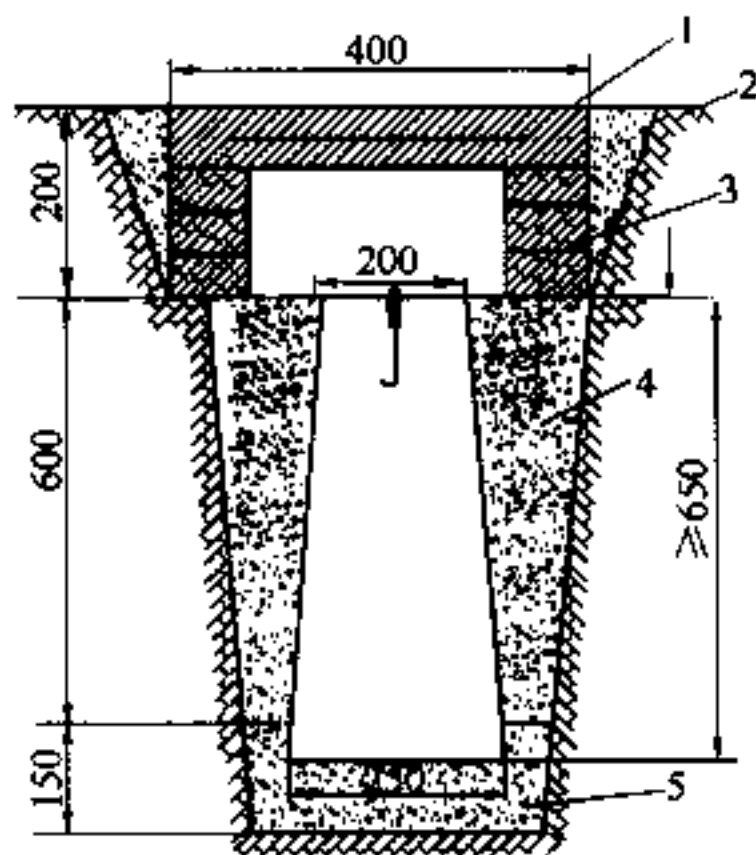
图 A. 2.5 四等平面控制点标石埋设图 (单位: mm)
