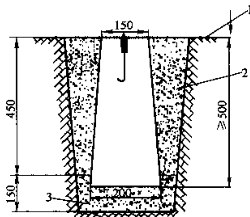
图 A. 2.6 五等及以下平面控制点标石埋设图 (单位: mm)
