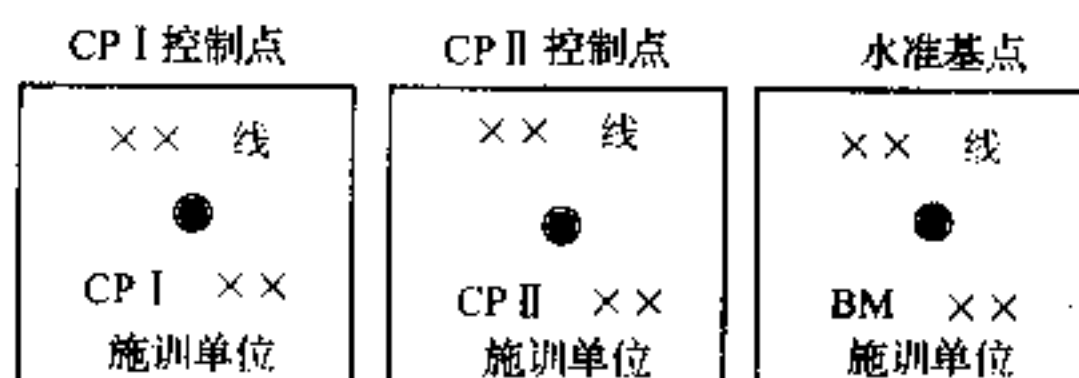
图 A. 6. 1 控制点标识示意图
