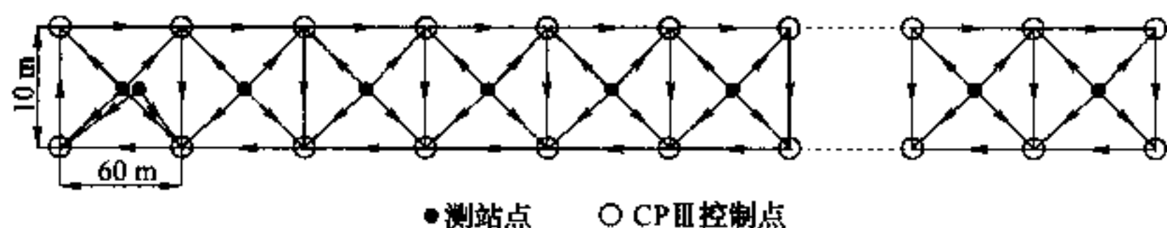
图 F. 2. 1—1 矩形环单程 CP III 水准网测量观测示意图
