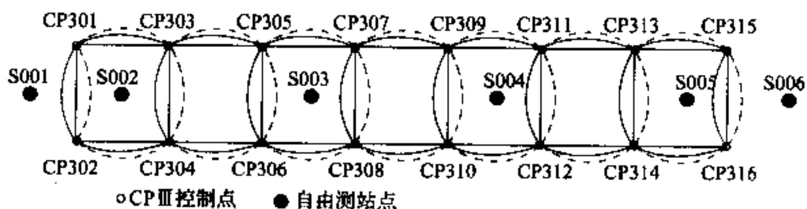
图 F.3.2 多个测站 CPⅢ控制网自由测站三角高程网示意图
