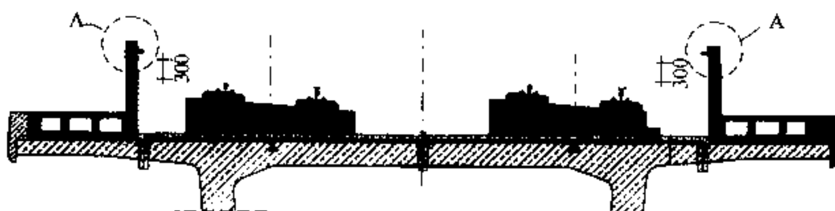
图 A. 4. 2—2 桥梁上 CPⅢ埋设示意图 (单位: mm)
