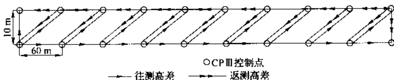
图 F. 2. 2—2 CP III 往返测水准路线返测观测示意图
