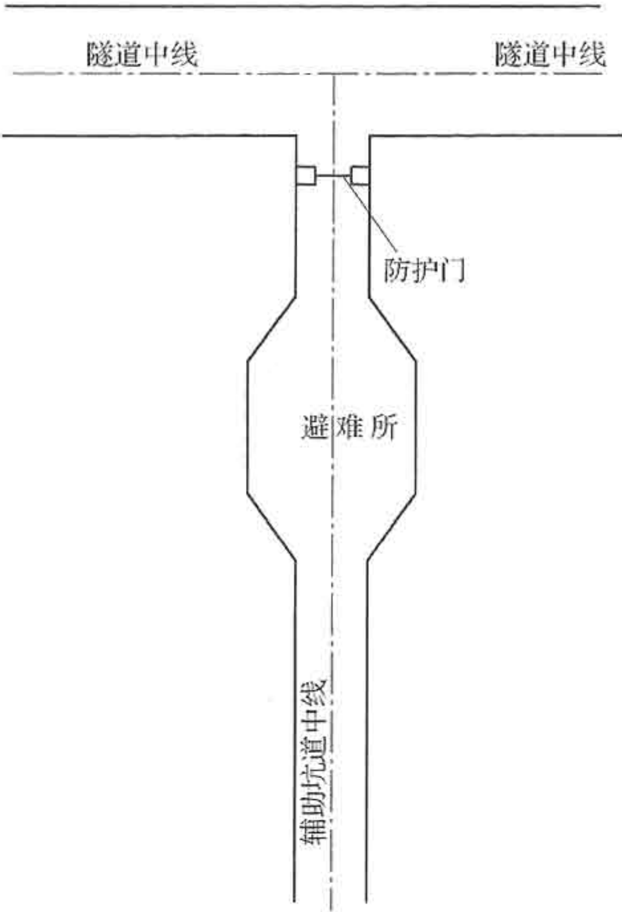
说明图 3.0.3 避难所设计示意图
