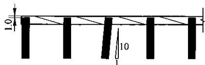
图 4 承载扁钢、横杆的偏差
