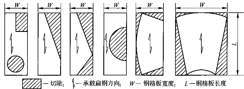
图 9 异形钢格板
