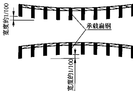
图 7 横向弯曲
