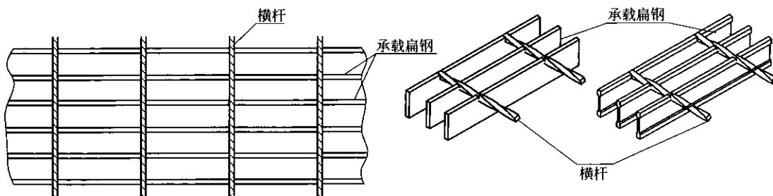
图1 压焊钢格板
