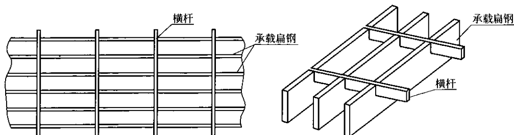
图2 压锁钢格板
