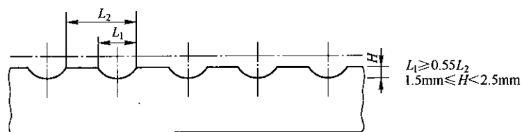
图 3 齿型尺寸
