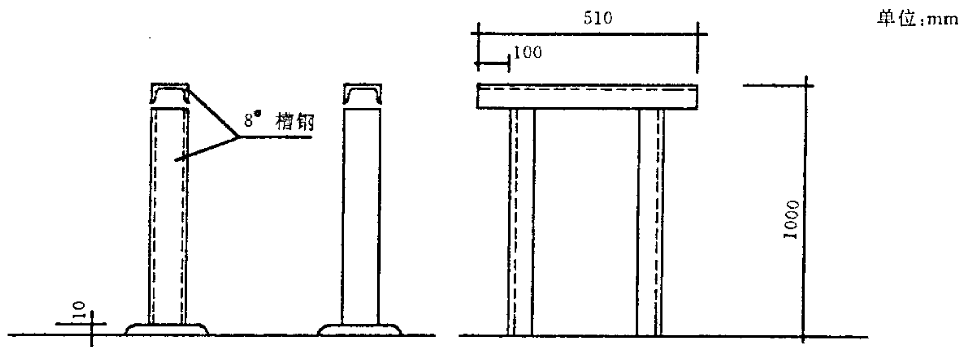
图 A1 支架
