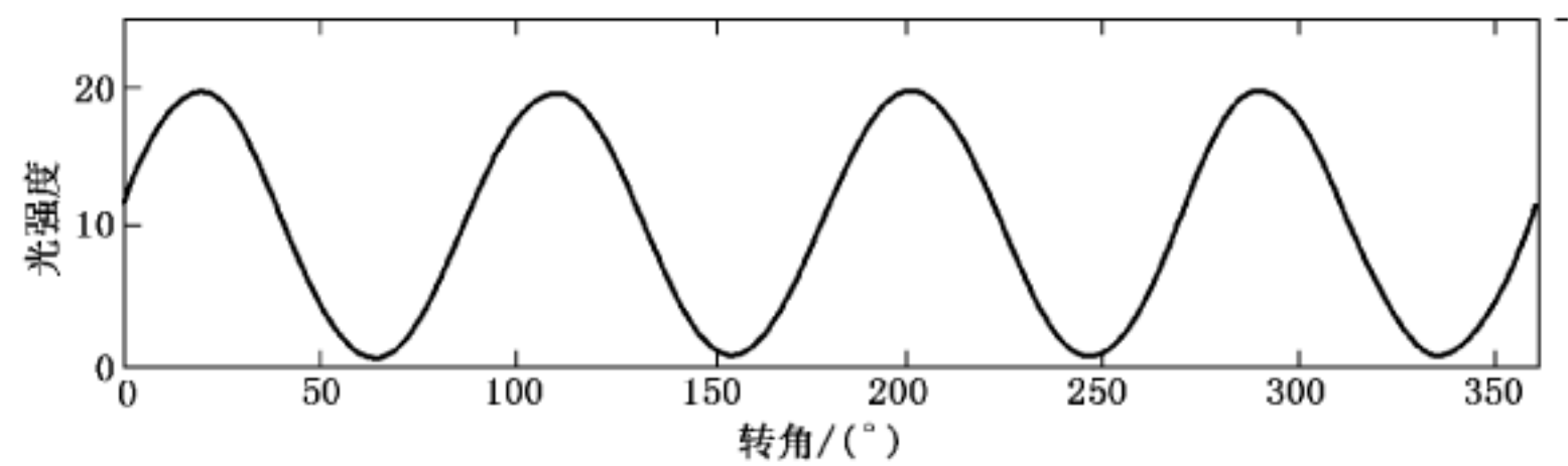
图 3 某检测点的原始测量数据
