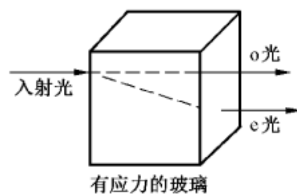
图 1 应力引起的光波双折射示意图
