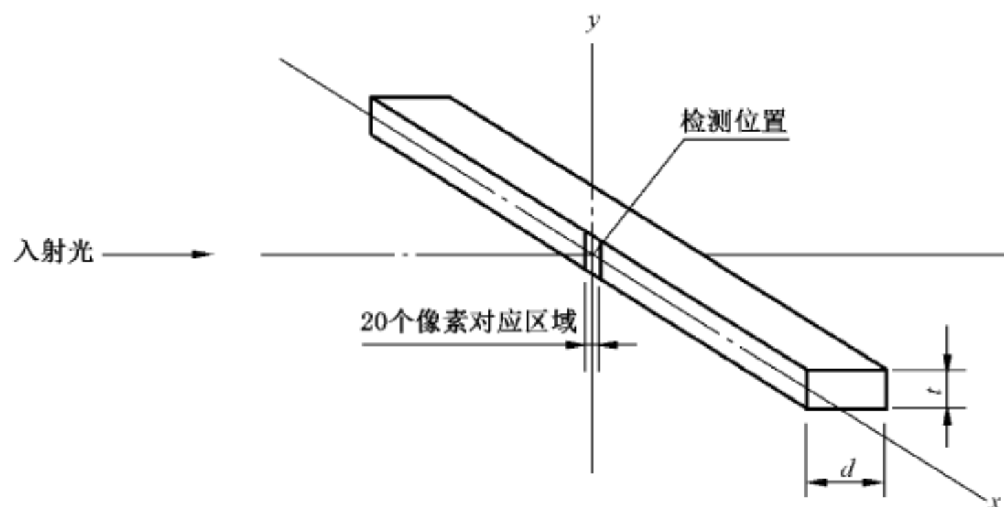
图 5 样品检测位置示意图
