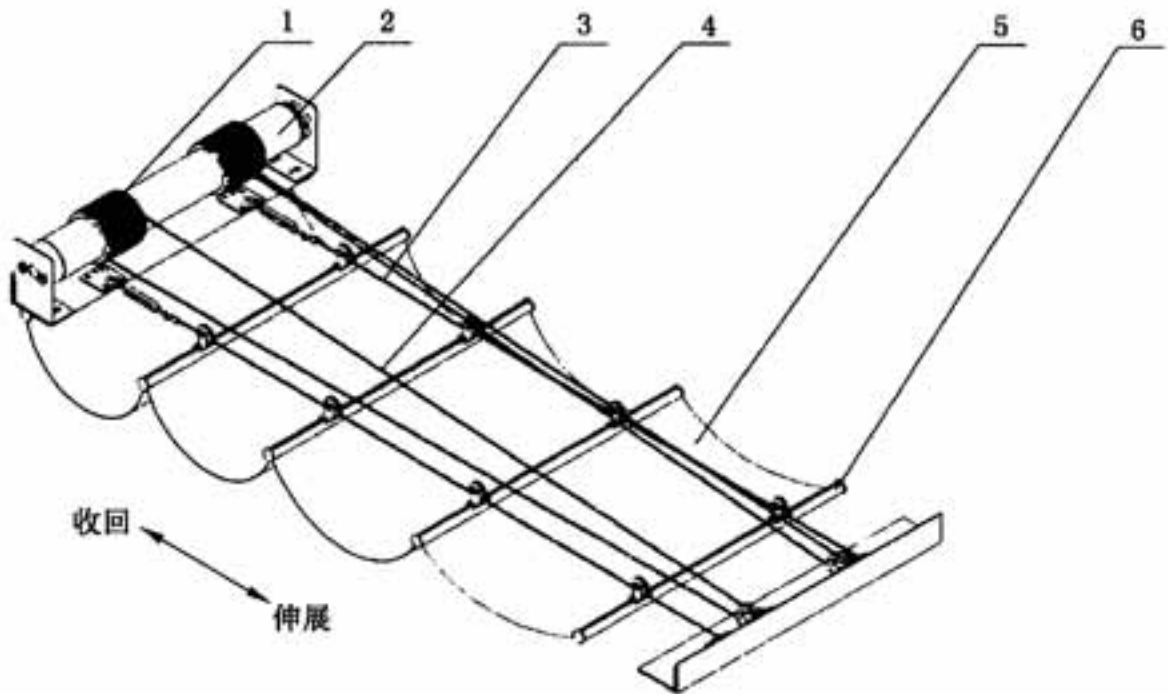
图 4 钢丝导向折叠式遮阳天篷帘结构示意图
