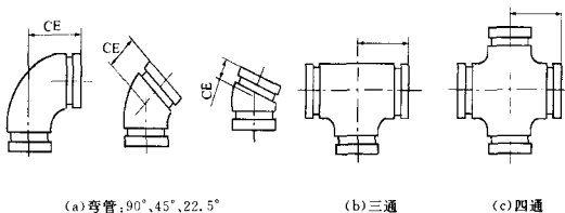
图 A. 0. 2 沟槽式管件
