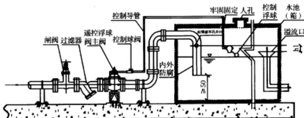
图 1 遥控浮球阀设置位置
