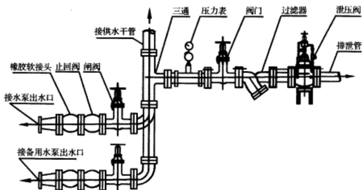
图 2 泄压阀设置位置
