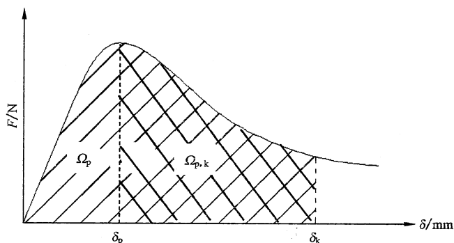
图4 等效弯曲强度计算
