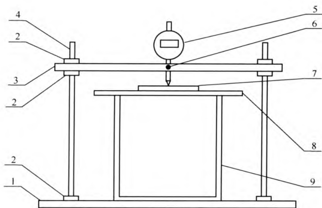
图 C.0.3 竖向膨胀率测量装置示意
