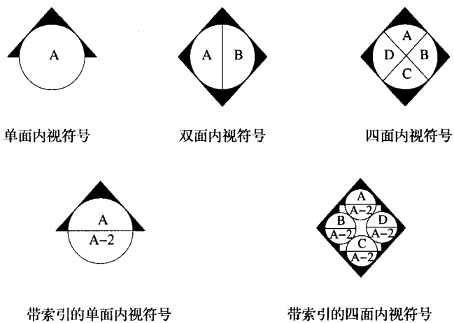
图 4.1.8-1 内视符号
