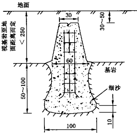
图 B. 4 基岩标石
