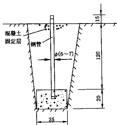
图 B.9 固定沙丘基本标石
