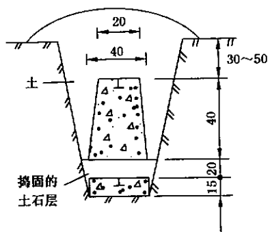
图 B.10 普通标石
