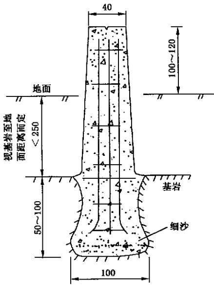
图 B. 2 基岩天线墩
