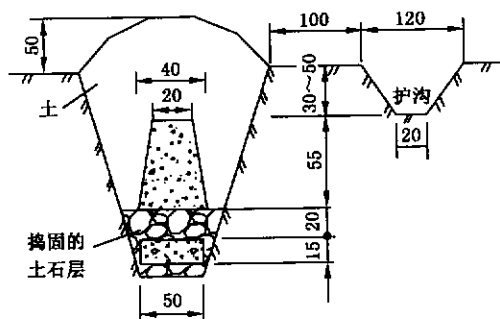
图 B.7 普通基本标石
