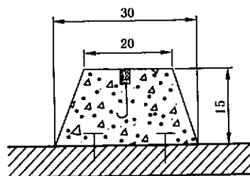
图 B.11 建筑物上标石
