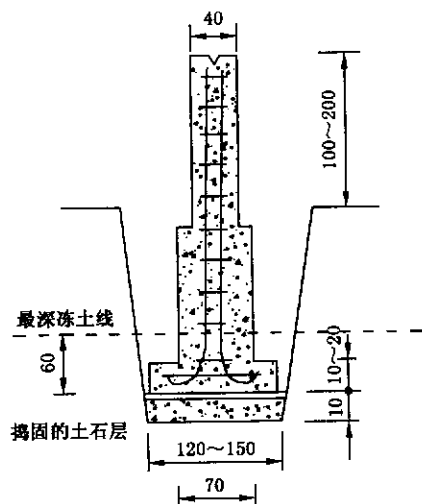
图 B.6 土层天线墩
