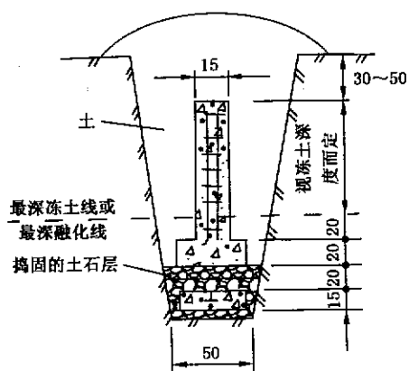
图 B.8 冻土基本标石
