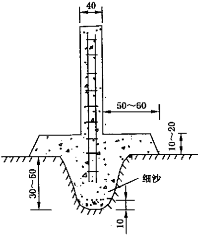
图 B. 3 岩石天线墩
