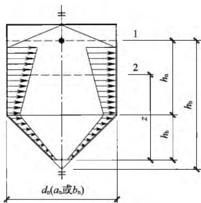
图 4.3.6-2 地震作用下贮料对钢筒仓筒壁局部压力竖向分布示意图
