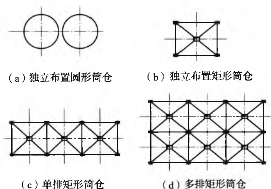
图 3.3.2 钢筒仓仓群平面布置形式示意图
