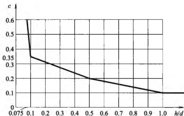
图 6.2.2-3 荷载分配系数 c
