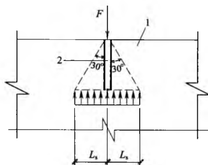
图 5.3.7 仓壁集中力示意图
