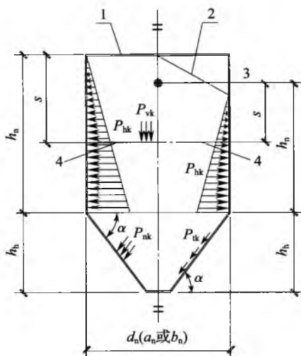
图 4.2.7 浅仓贮料压力示意图
