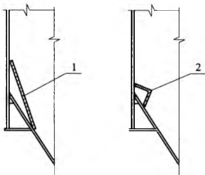
图 8.0.4 焊缝防护大样示意
