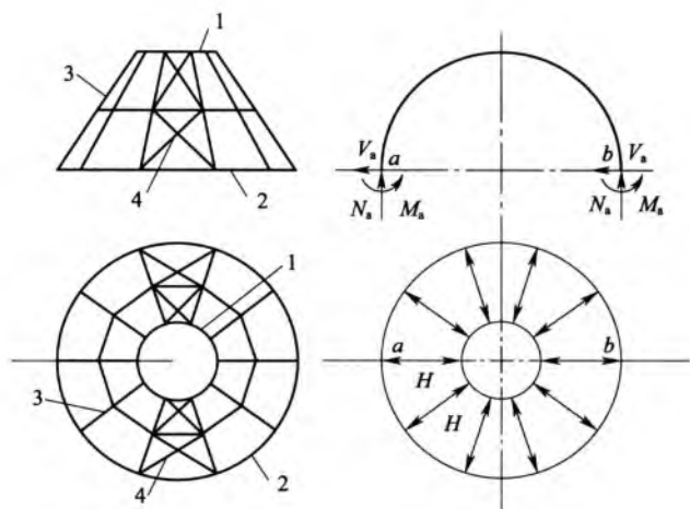
图 5.2.3 正截锥仓顶及环梁内力示意图
