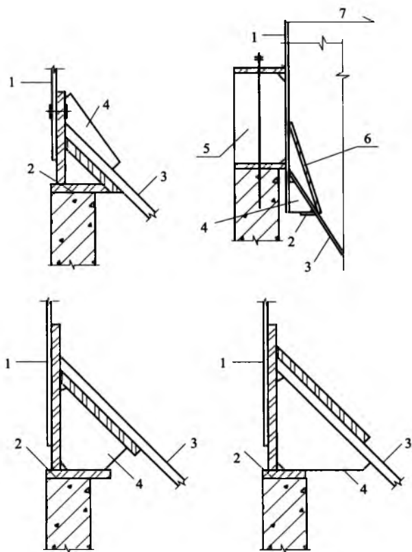
图 5.4.2 漏斗环梁示意
