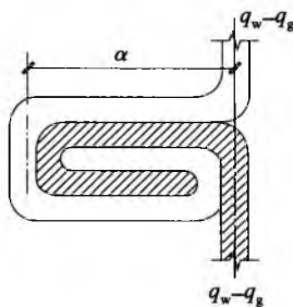
图 5.3.9 咬口弯卷示意
