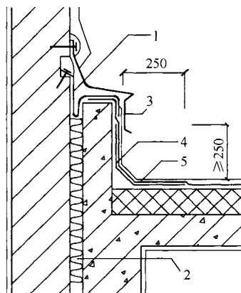
图 4.11.18-2 高低跨变形缝
