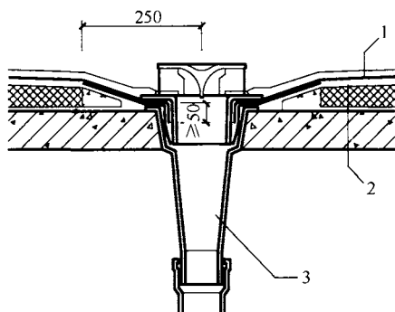
图 4.11.16-1 直式水落口
