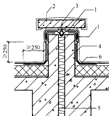
图 4.11.18-1 等高变形缝
