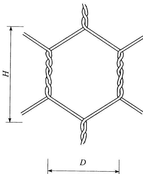
图 1 机编网目示意图
