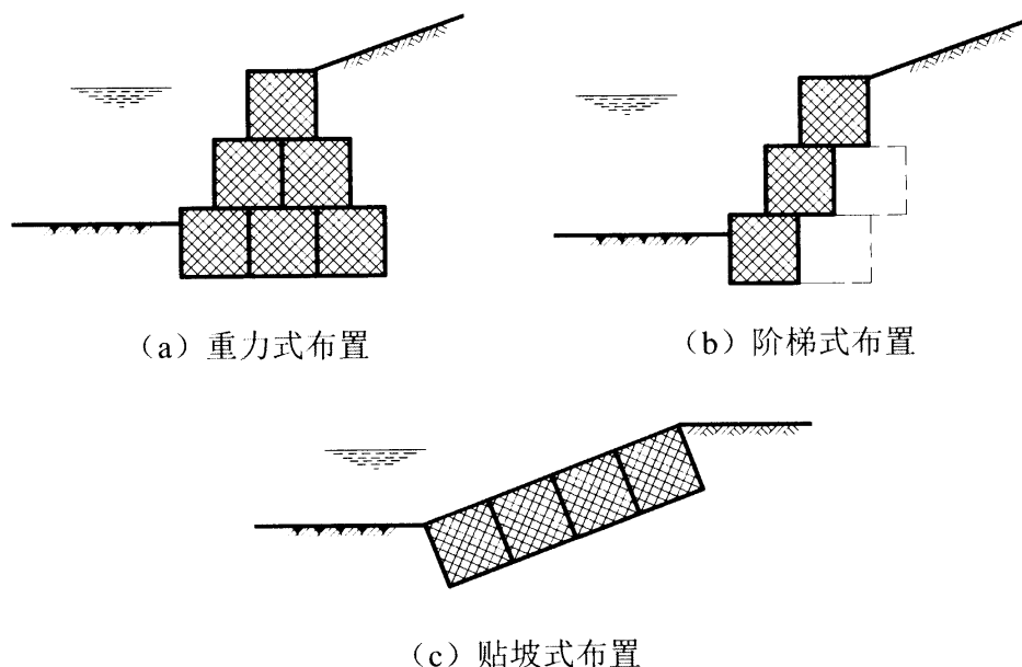
图 4.1.1 格网土石笼布置示意图
