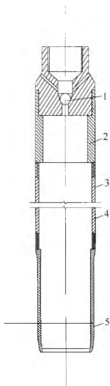
图 E. 0.1-5 束节式取土器
