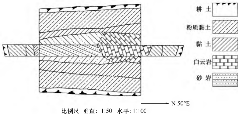
图 F.0.2 探槽剖面展开图式
