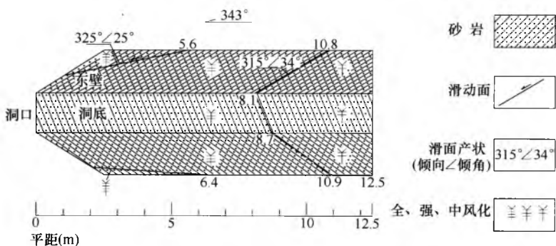
图 F.0.3 探洞剖面展开图式
