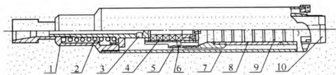
图 E.0.1-12 双管单动内环刀取砂器结构示意图
