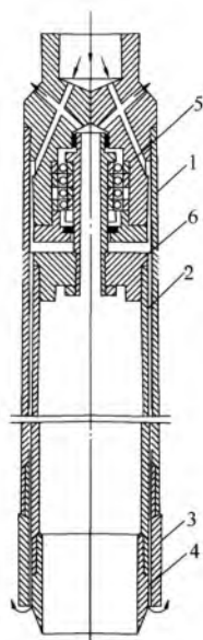
图 E. 0. 1-7 单动二(三)
