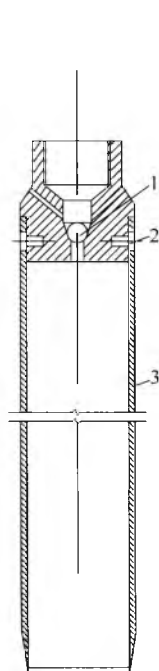
图 E. 0. 1-1 敞口薄 壁取土器
