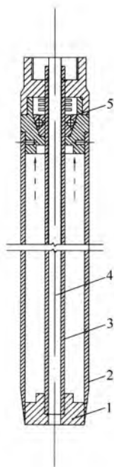
图 E.0.1-4 自由活塞 取土器
