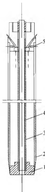
图 E. 0. 1-2 固定活塞 取土器
