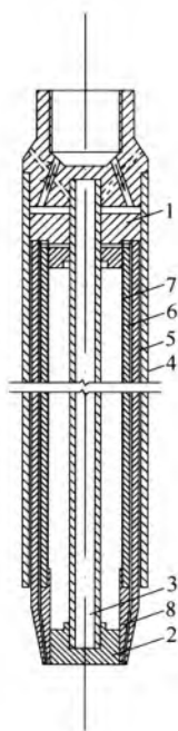
图 E.0.1-3 水压固定 活塞取土器
