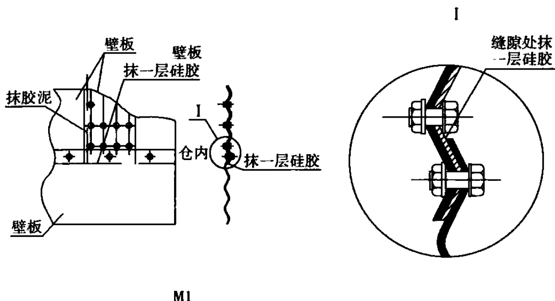
图 6.5.1 波纹板连接示意图
