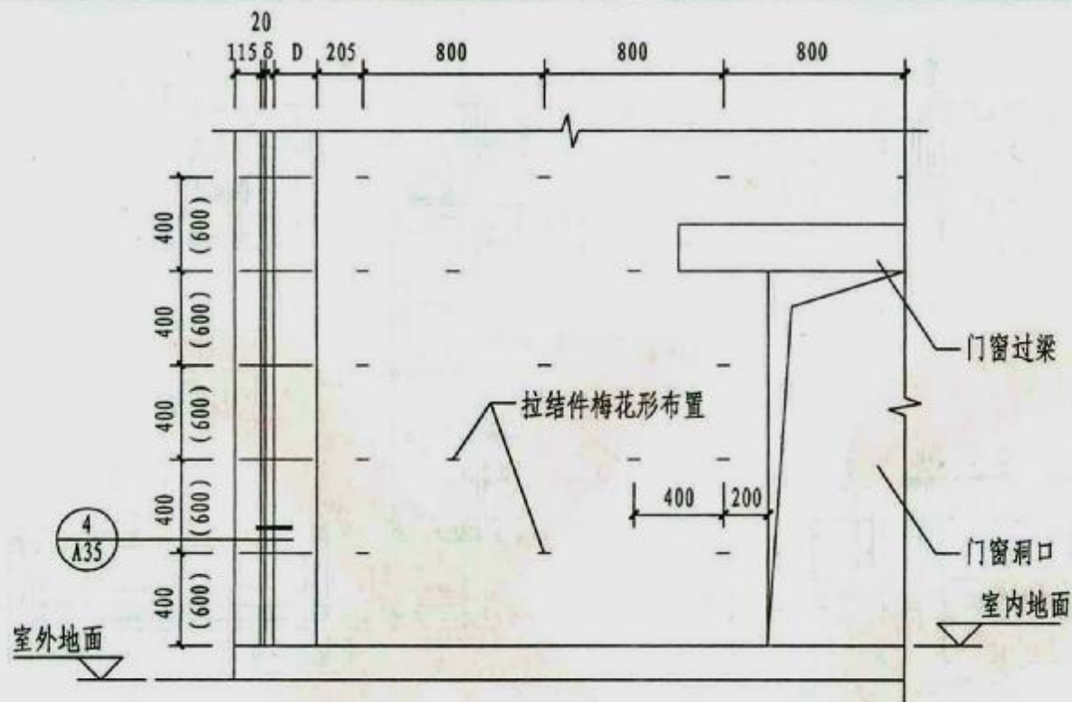
① 拉结件立面示意图
