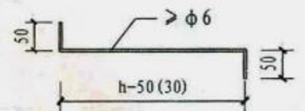
③ B Z形拉结件
