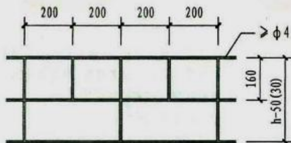
D 钢筋网片
