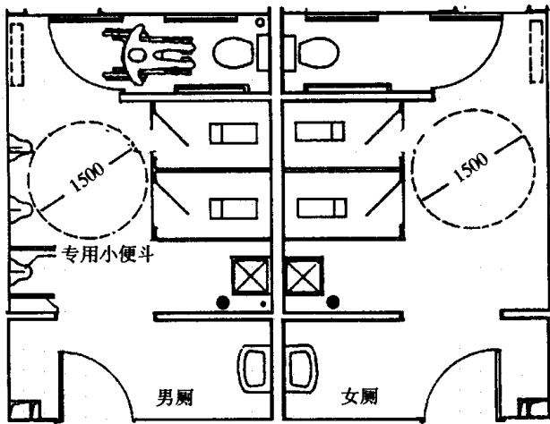
图 16 轮椅可进入的厕位 (mm)
