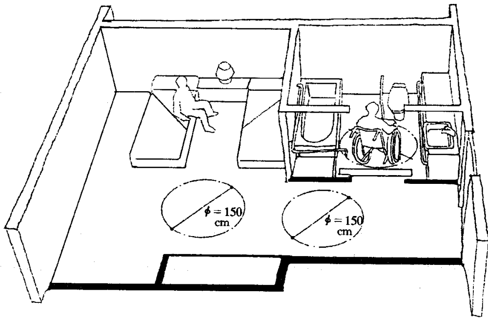
图 19 残疾人客房
