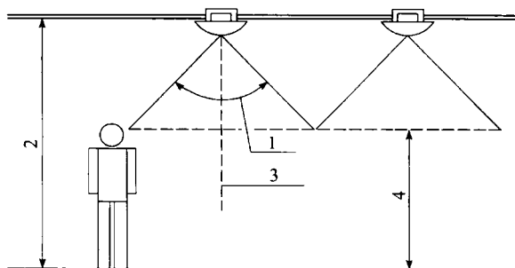
图 2.0.18 扬声器有效覆盖角示意图
