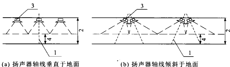
图 1 扬声器倾斜角度示意图
