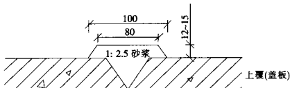
图 4.4.12 板间拼缝断面
