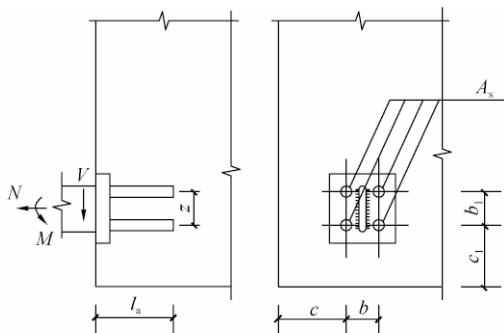
图 C.0.1 锚板和直锚筋组成的预埋件示意
