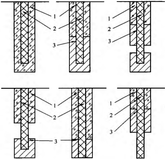
图 3 三元复合桩其他构造形式示意图
