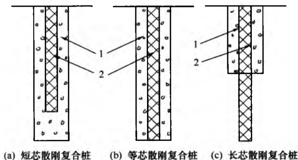
图 4.2.2 散刚复合桩构造示意图
