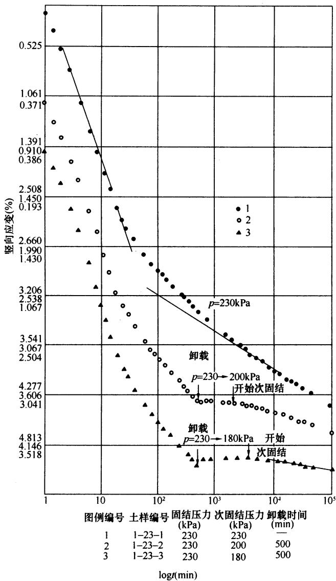
图 6 某工程淤泥质黏土的室内试验结果
