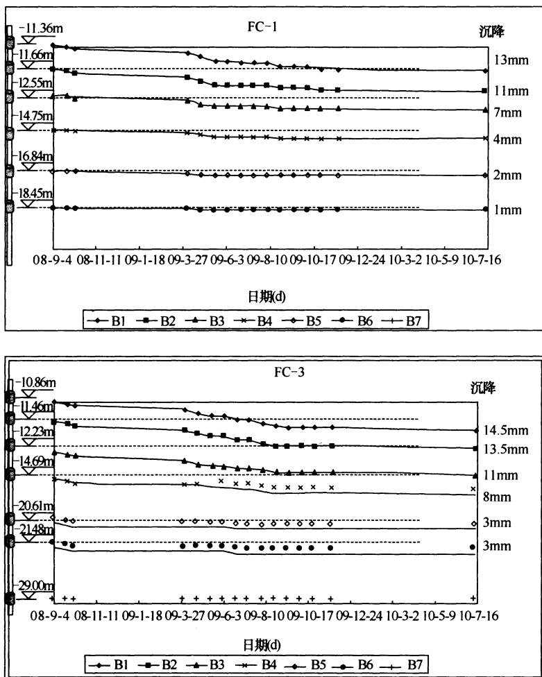
图 13 分层沉降变形曲线
