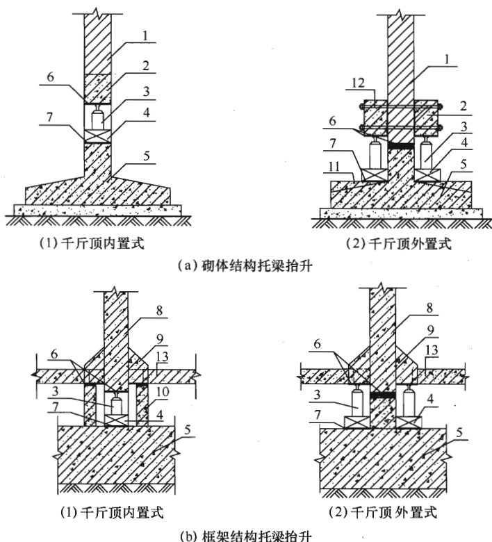
图 5.4.5 上部结构托梁抬升法示意
