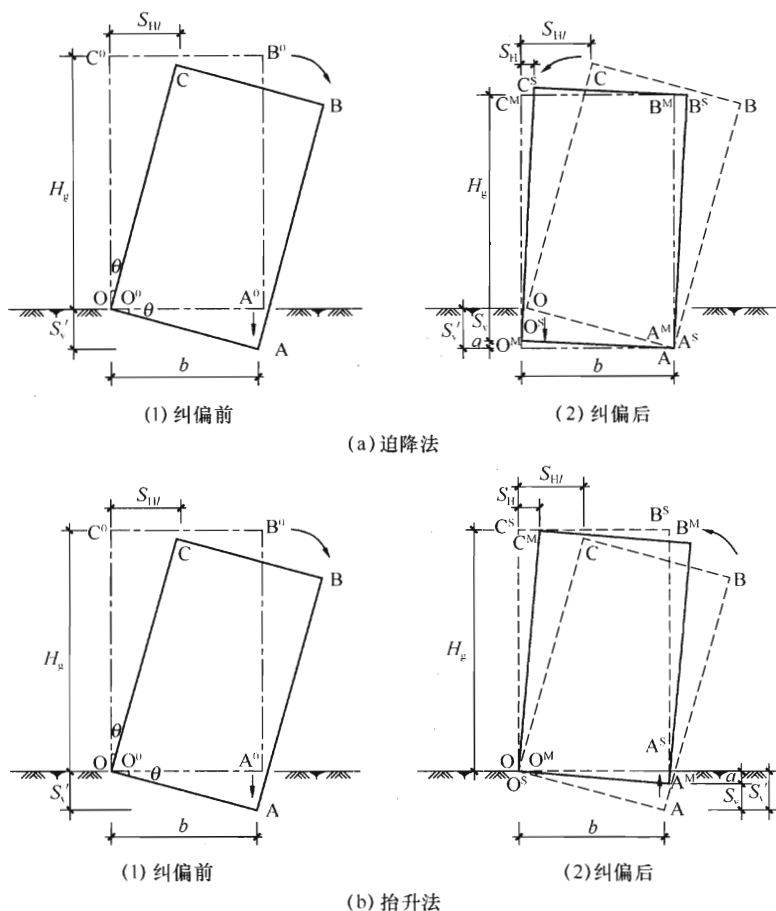
图 5.2.2 纠偏迫降或抬升计算示意
