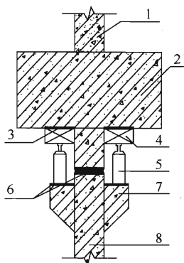
图 5.3.11 断桩托换体系示意
