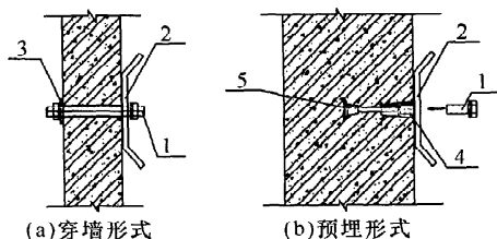
图2 承载螺栓的两种形式
