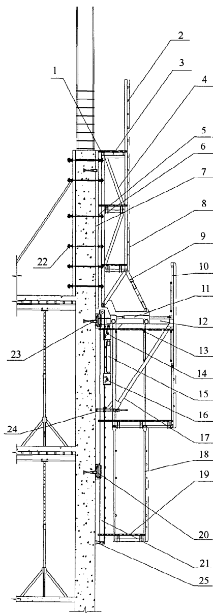
图4 油缸和架体的爬模装置示意
