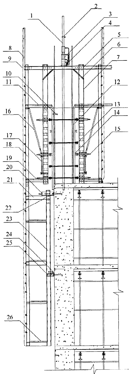
图5 千斤顶和提升架的爬模装置示意
