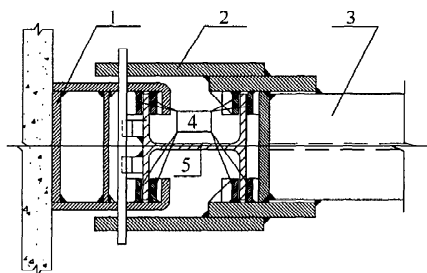
图 8 挂钩连接座与下架横梁焊缝示意
