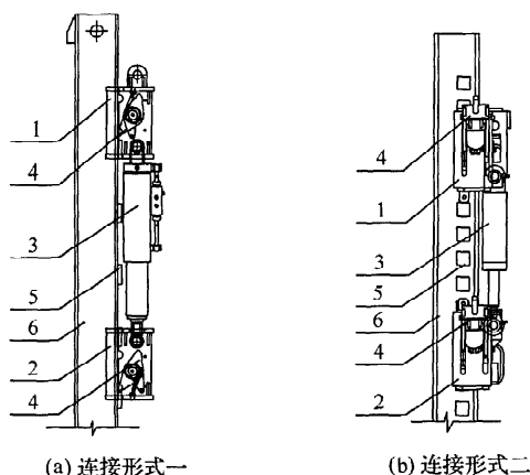
图 6 防坠爬升器与导轨的连接形式
