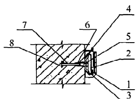
图3 挂钩连接座构造
