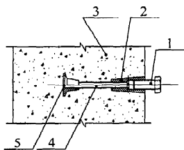
图 1 锥形承载接头构造
