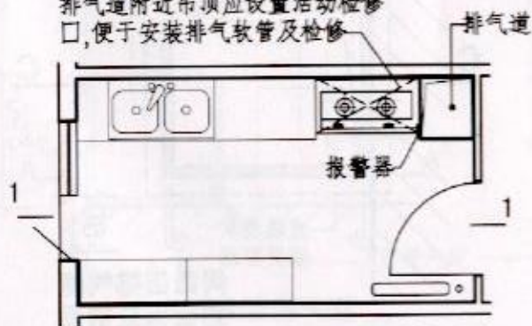
厨房平面示例
