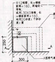
双面靠墙排气道 变截面示例
