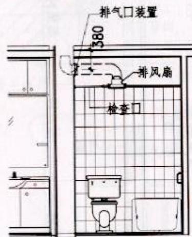
2 - 2 剖面
