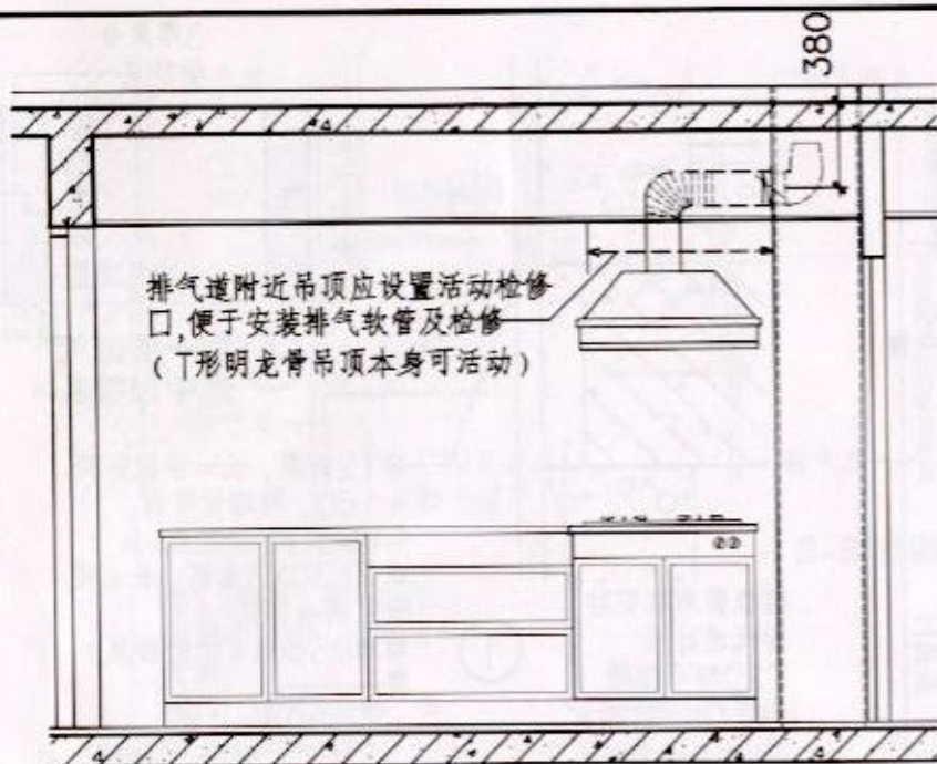
1 - 1 剖面
