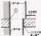
A-A变截面处断面
