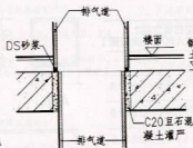
B-B变截面处断面
