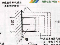
单面靠墙排气道 变截面示例
