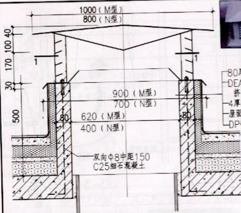
排气道出屋面处风帽剖面
