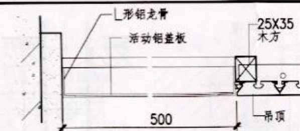
检修口示例
