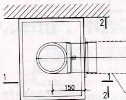
厨房排气道排气口处平面
