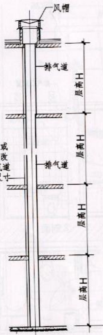
排气道竖剖面
