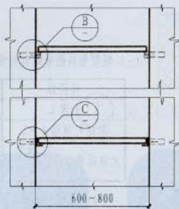
搁板立面
