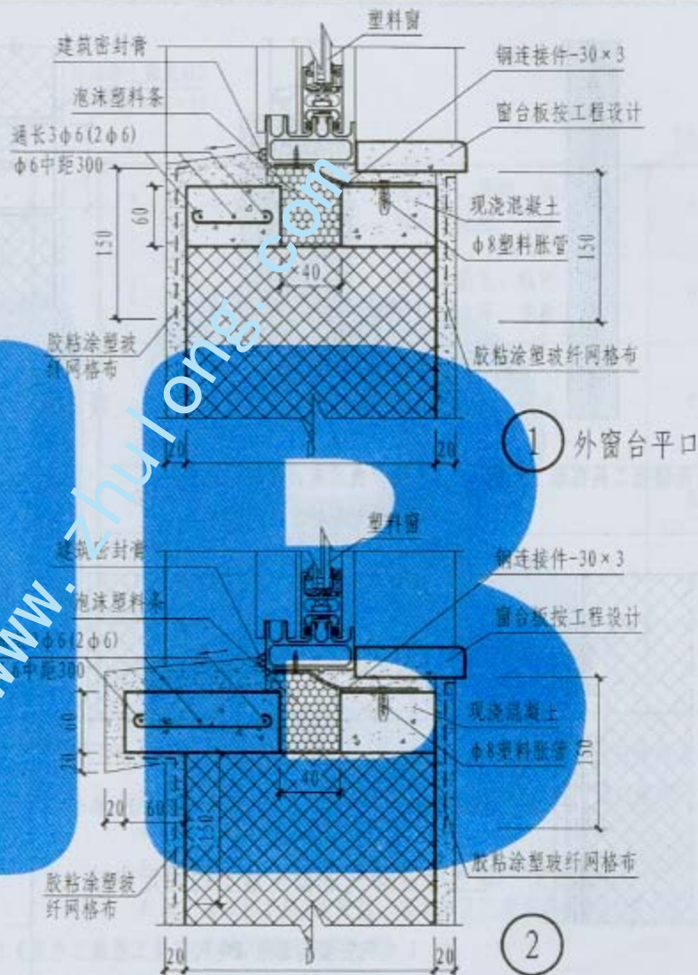
窗与墙间缝隙及窗台详图
