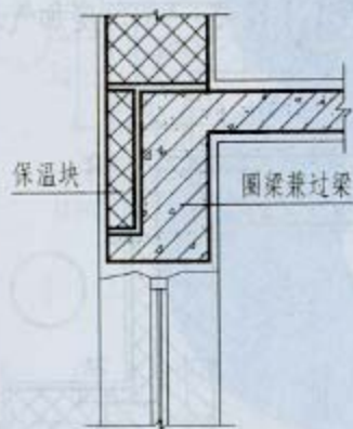
4 外墙窗口
