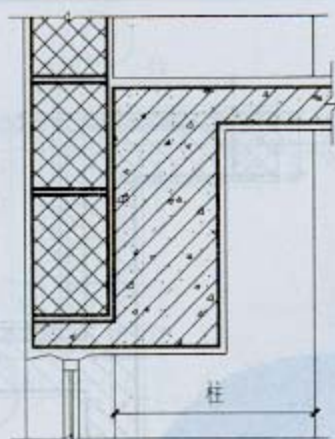
1 外墙窗口 (框架)
