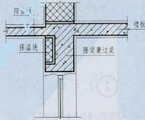
6 阳台部位
