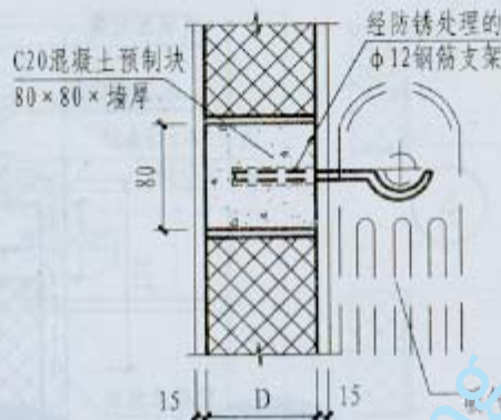
暖气片与墙体连接
