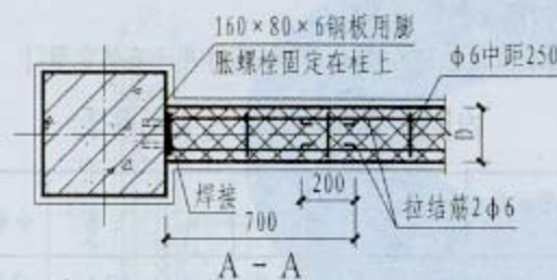
1 加气混凝土填充墙与框架柱拉结
