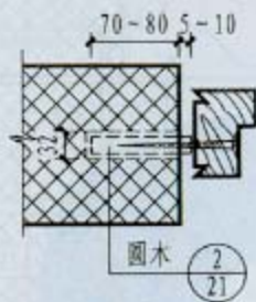
2 胶粘圆木安装法
