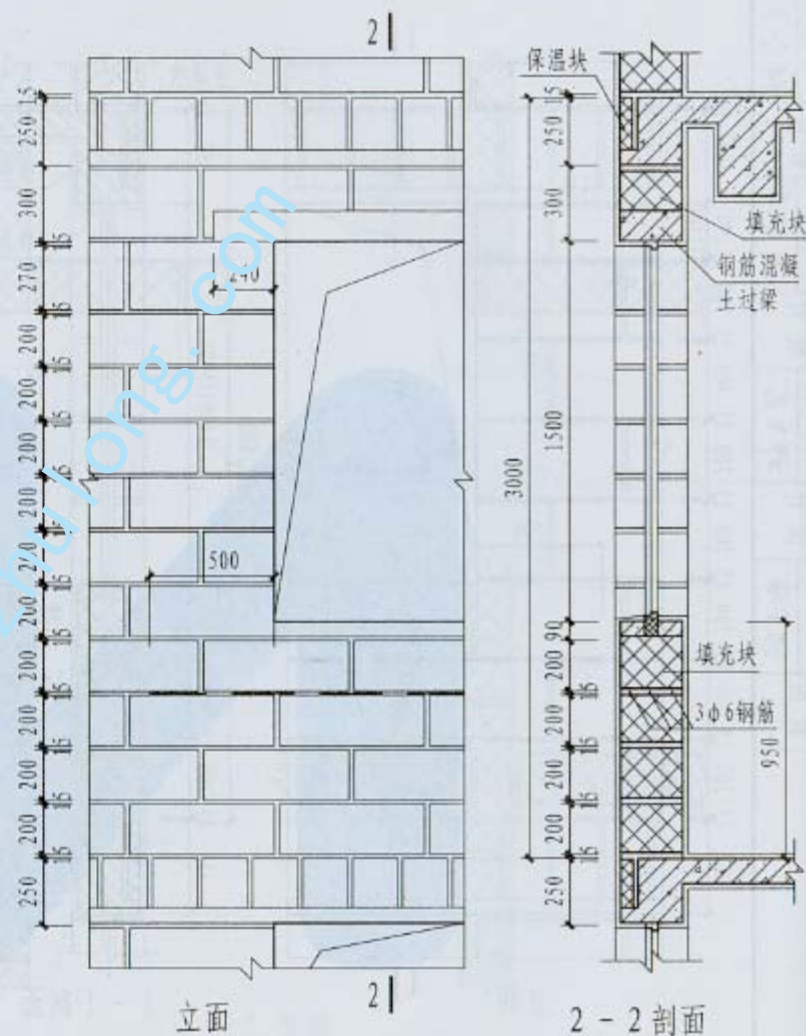
3000层高, 200高砌块, 1500窗高外墙砌块排列示例
