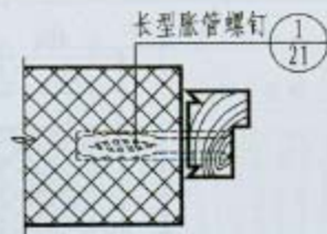
1 塑料胀管螺钉安装法
