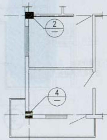
平面示例 (墙在柱间)
