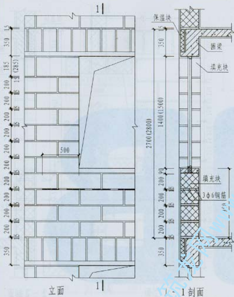
2700(2800)层高, 200高砌块, 1400(1500)窗高外墙砌块排列示例
