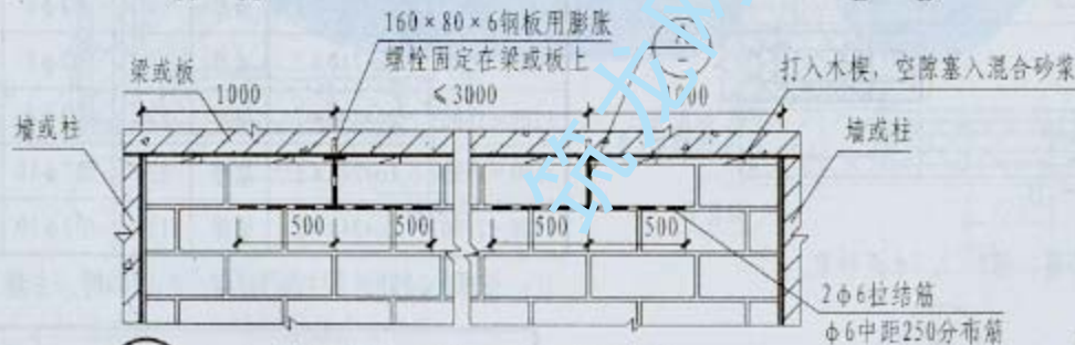
3 加气混凝土填充墙顶与梁或板拉结
