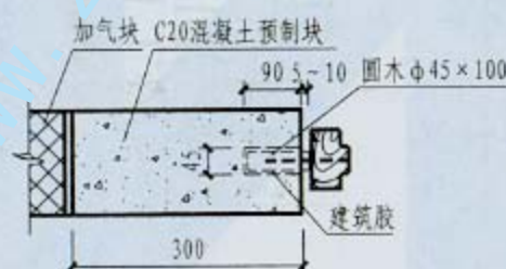
6 重型门固定法 (适用于内门)
