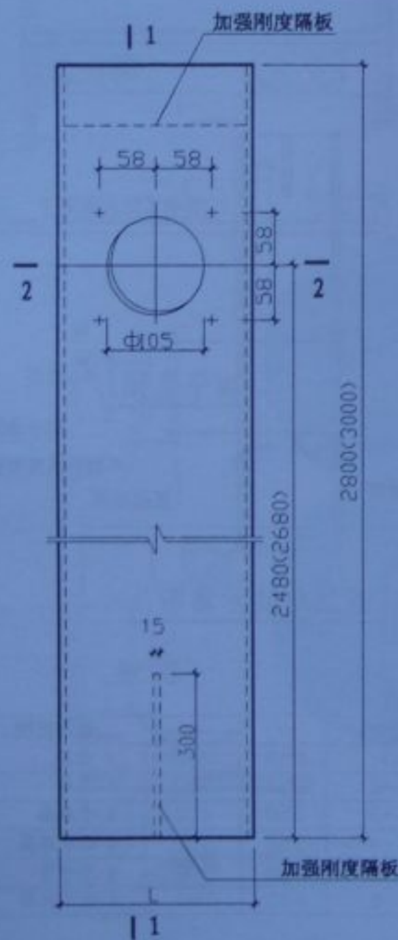
立面图
