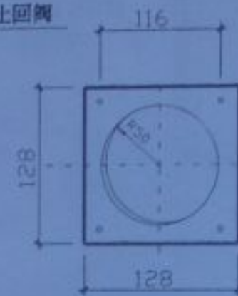
卫生间止回阀连接底板 (成品)
