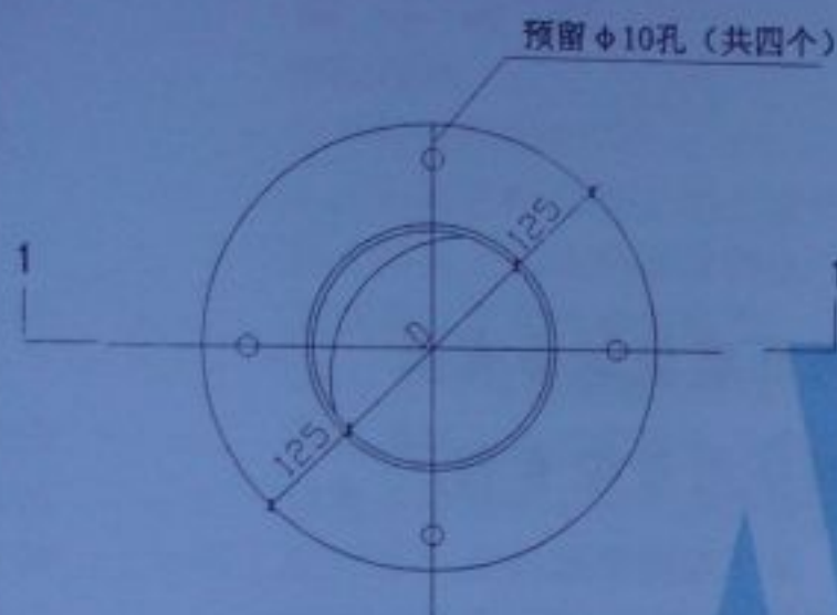
无动力排气风帽底座接口钢板
