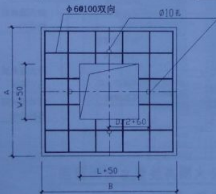
出气口盖板配筋平面图
