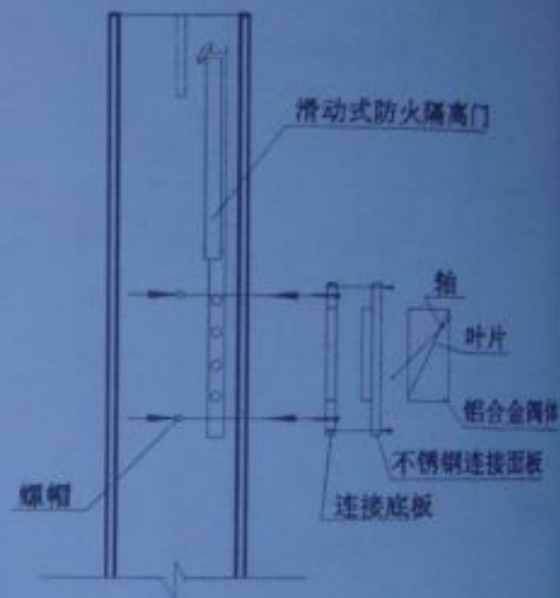
系统组装示意图
