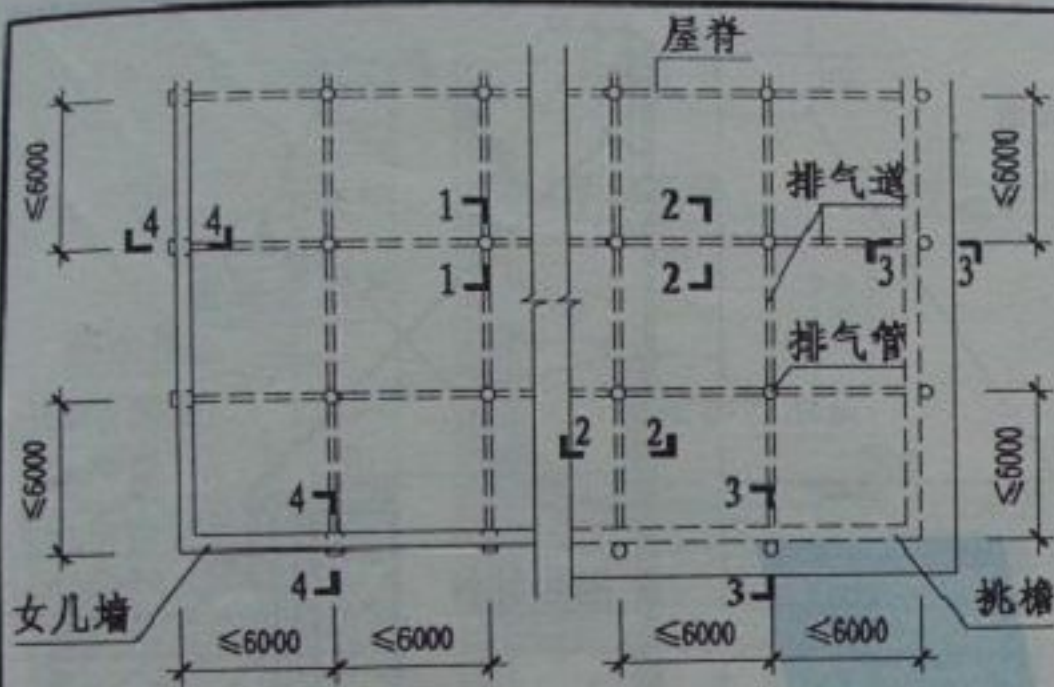
排气道、排气管平面布置
