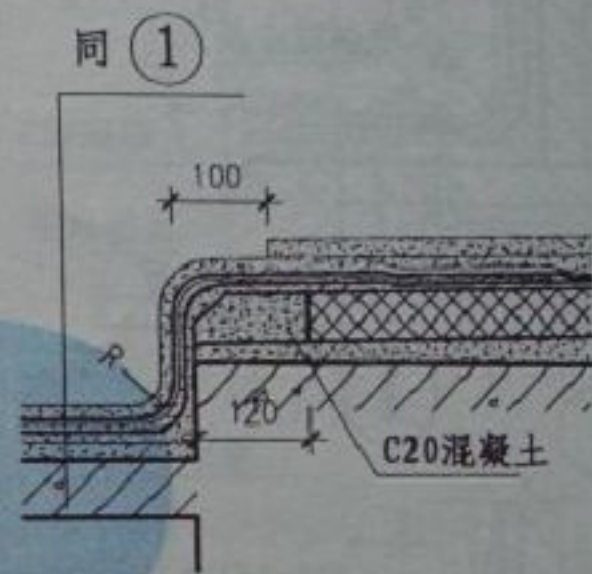
③ 细石混凝土屋面
