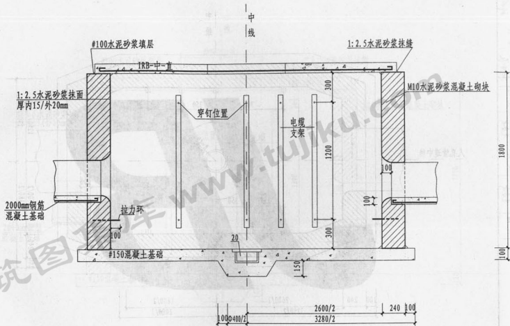
中号直通型人孔断面图
